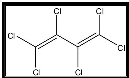
Figur 5. Molekylstrukturen av HCBD
