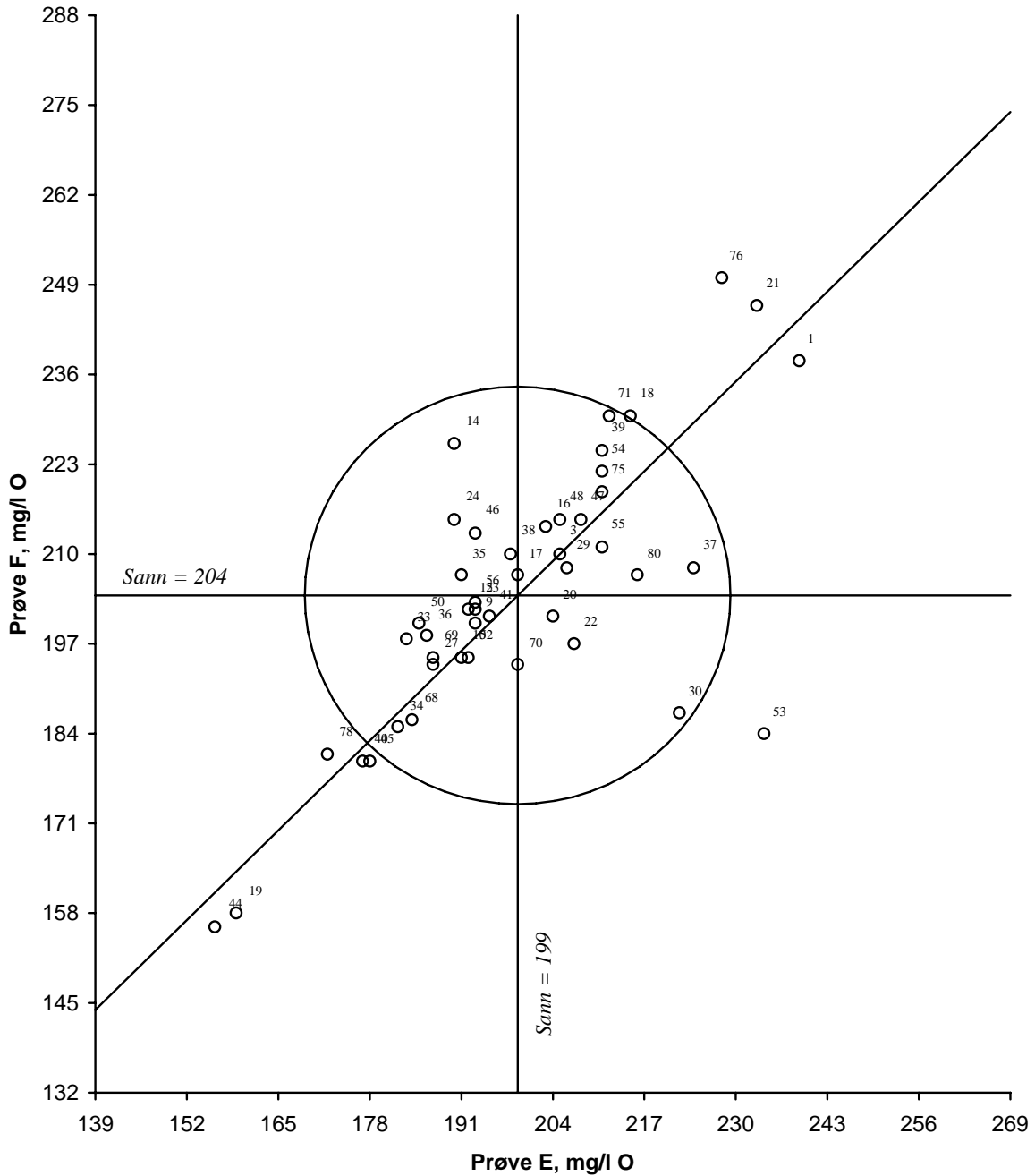
Figur 7. Youtendiagram for kjemisk oksygenforbruk, COD_{Cr} , prøvepar EF Akseptansegrensen, angitt med en sirkel, er 15 %
