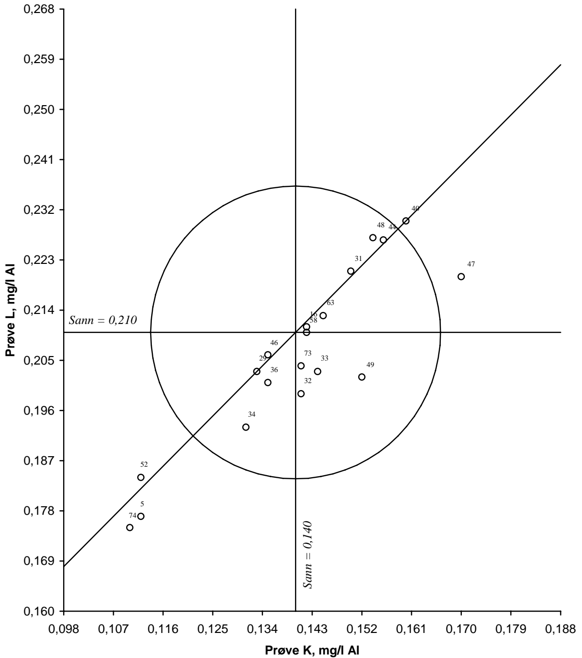
Figur 20. Youdendigram for aluminium, prøvepar KL Akseptansegrensen, angitt med en sirkel, er 15 %
