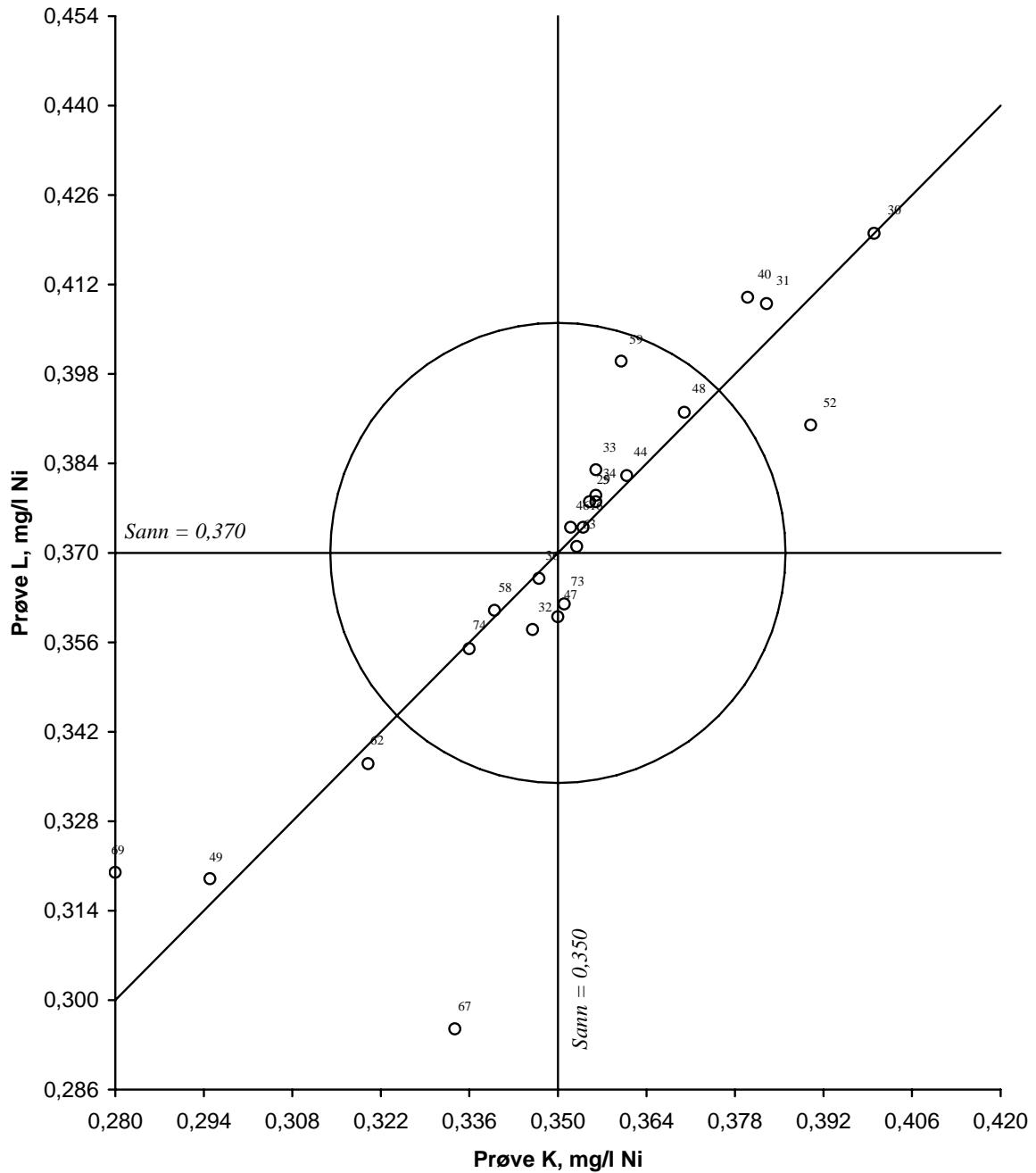
Figur 34. Youdendiagram for nikkell, prøvepar KL Akseptansegrensen, angitt med en sirkel, er 10 %
