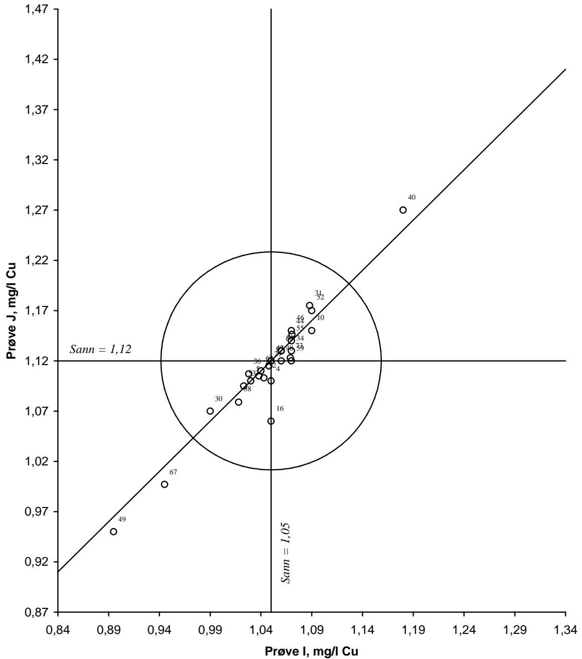
Figur 27. Youtendigram for kobber, prøvepar IJ Akseptansegrensen, angitt med en sirkel, er 10 %
