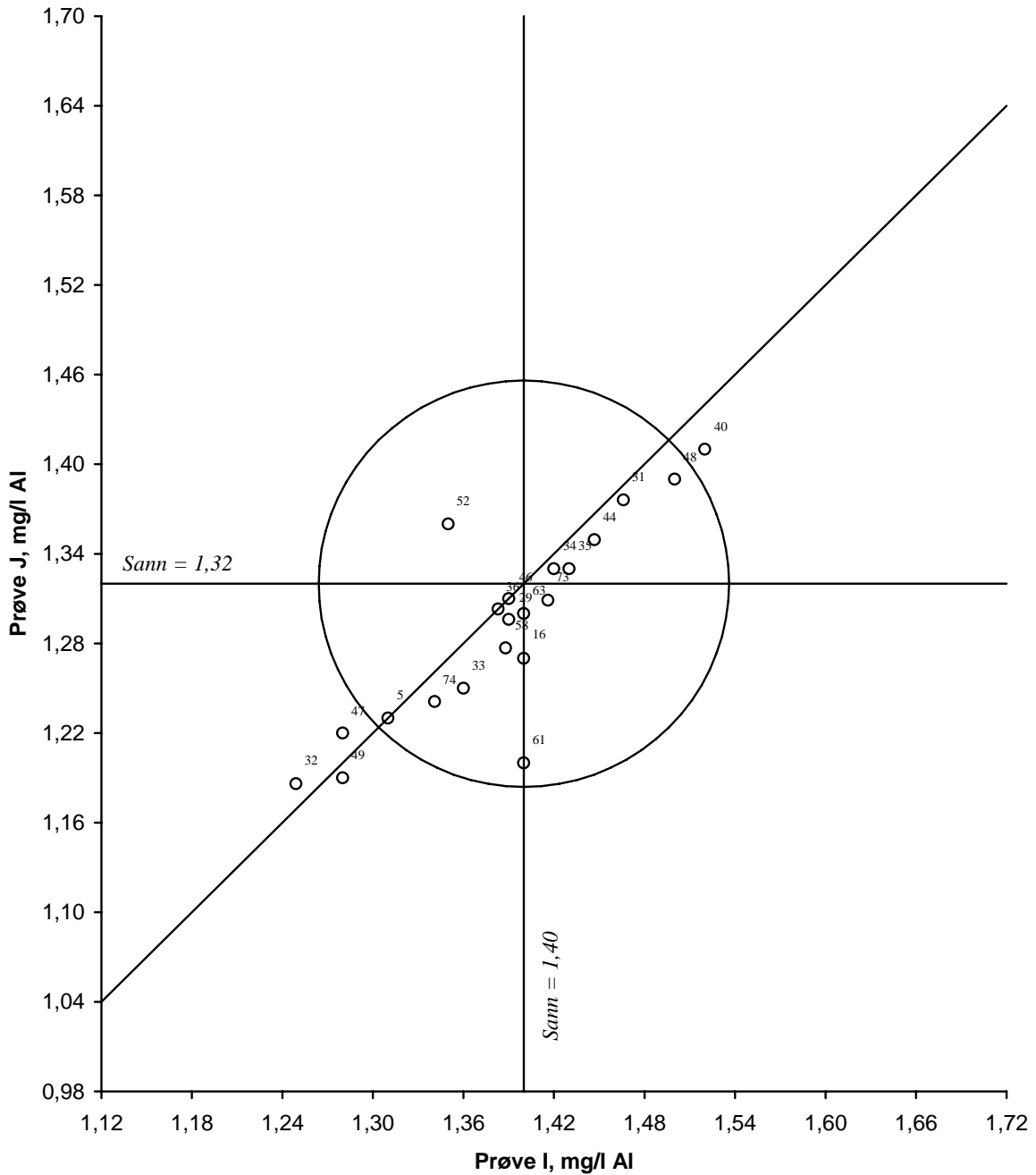
Figur 19. Youdendigram for aluminium, prøvepar IJ Akseptansegrensen, angitt med en sirkel, er 10 %
