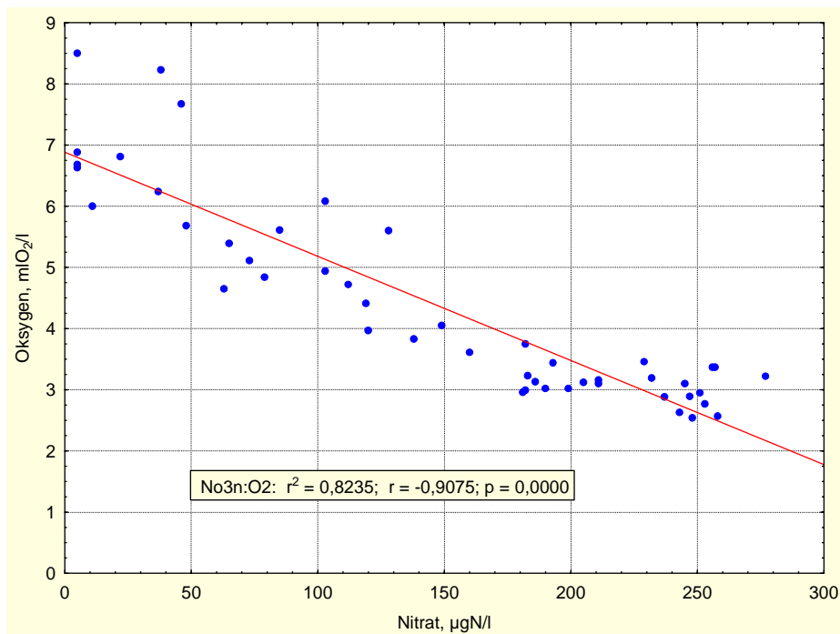
Figur 6. Oksygen og nitrat i hhv. 10-40 m dyp i Havnebassenet (øverst) og i 10-80 m dyp ved Lindenes (nederst) i 2006. Korrelasjoner på ca. r^2=0,86 ca. r^2=0,82 forteller at mer enn 80 % av endringene i oksygenkonsentrasjon kan forklares med tilsvarende endringer i konsentrasjonen av nitrat (høy N-konsentrasjon gir lav \text{O}_2 -konsentrasjon, og omvendt). Dette kan regnes som en sterk sammenheng. Utlekkingen av nitrat fra dicy-kalk på bunnen fører fortsatt til økt oksygenforbruk i vannmassene.
