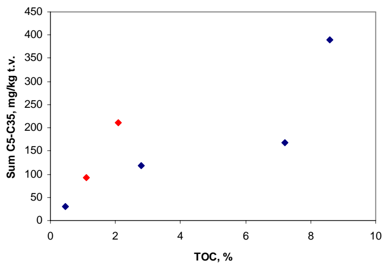
Figur 3. Sammenhengen mellom andelen totalt organisk karbon (TOC) og konsentrasjon av sum alifatiske hydrokarboner (Fraksjon C5-C35). Figuren viser resultater fra både molofyllmasse (rød punkter) og sedimenter (blå punkter).
