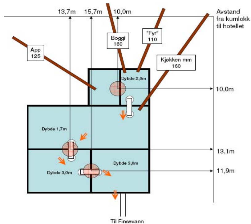
Fig 5. Kartskisse av avløpssystem for Finseområdet med tilhørende infoog tegn av kum nr 4.
