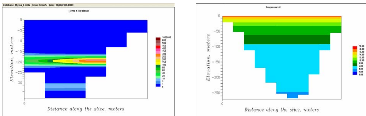
Figur 11. Vest-øst tverrsnitt av bakterier ved Moelv rensanlegg og temperatur ved fra Rambekk rensanlegg
