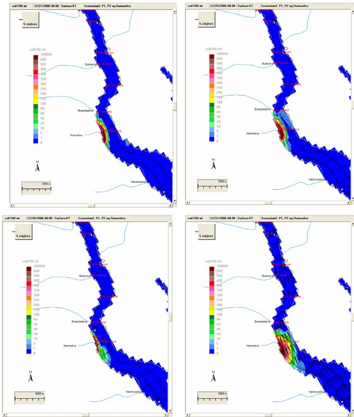
Figur 37. Scenario 2: Brudd på kloakkledningen ved stasjon P1, P2 og Hunnsetelva. E. coli på overflaten 21., 25., 28., og 31. desember 2006.
