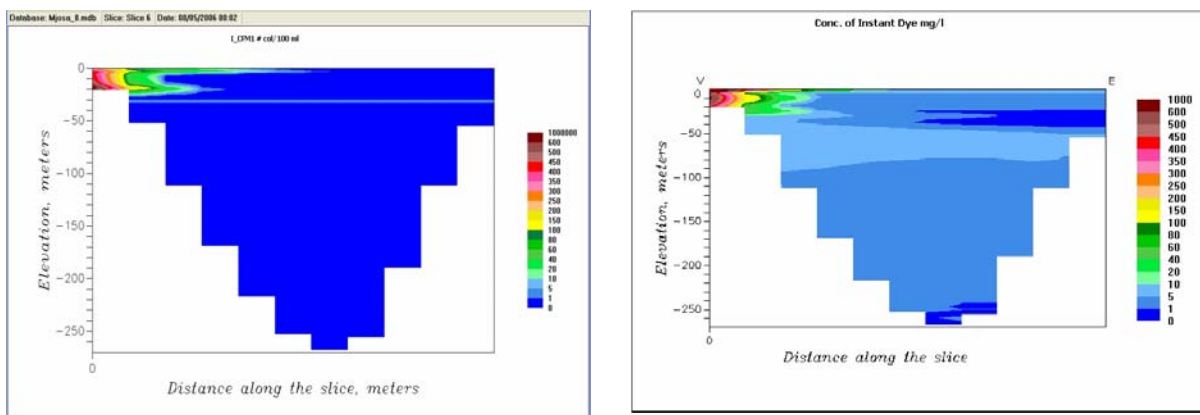
Figur 10. Vest-øst tverrsnitt ved fra Rambekk rensanlegg av bakterier (v) og konservativt stoff (h).
