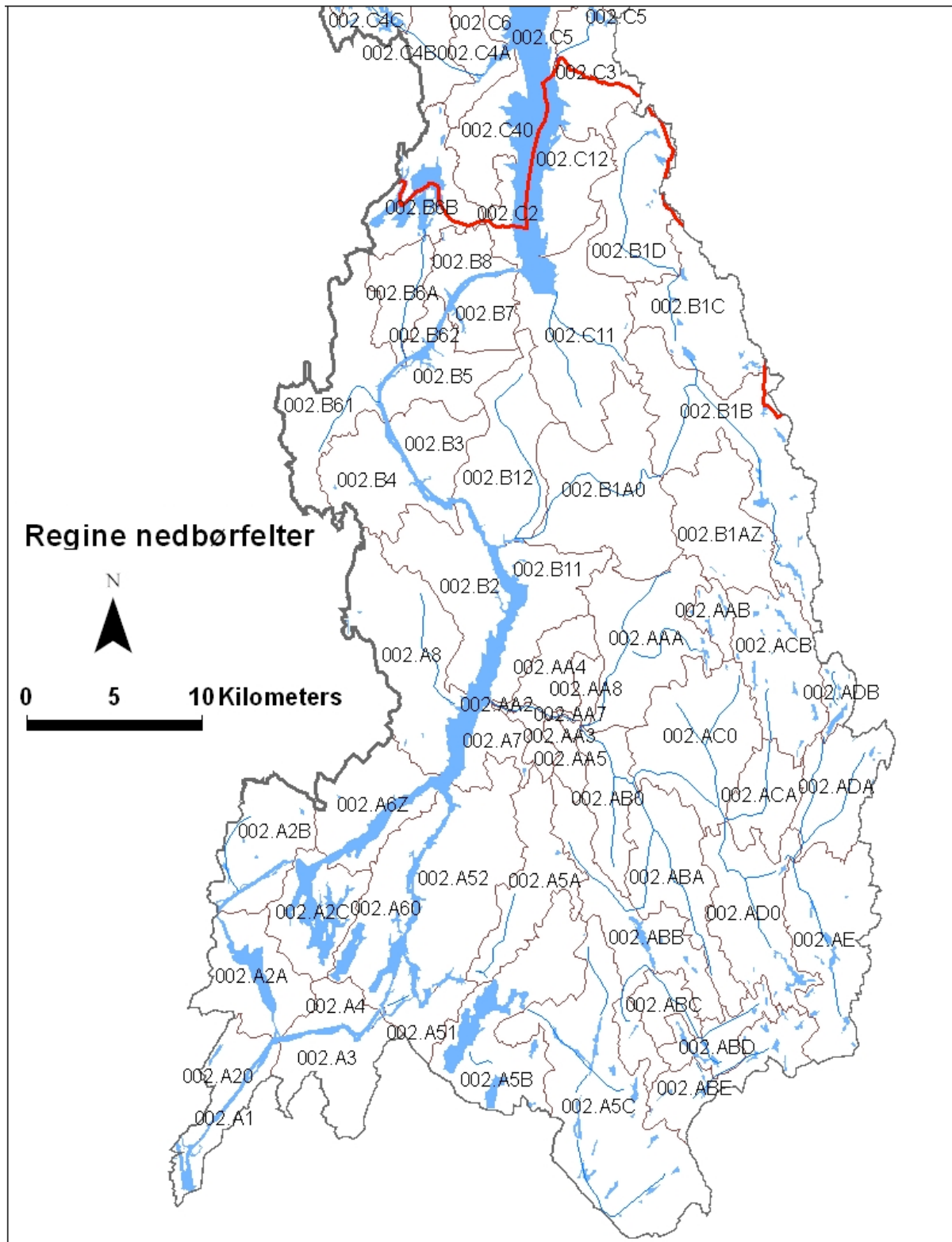
Figur. Inndelingen i Regine nedbørfelt.
