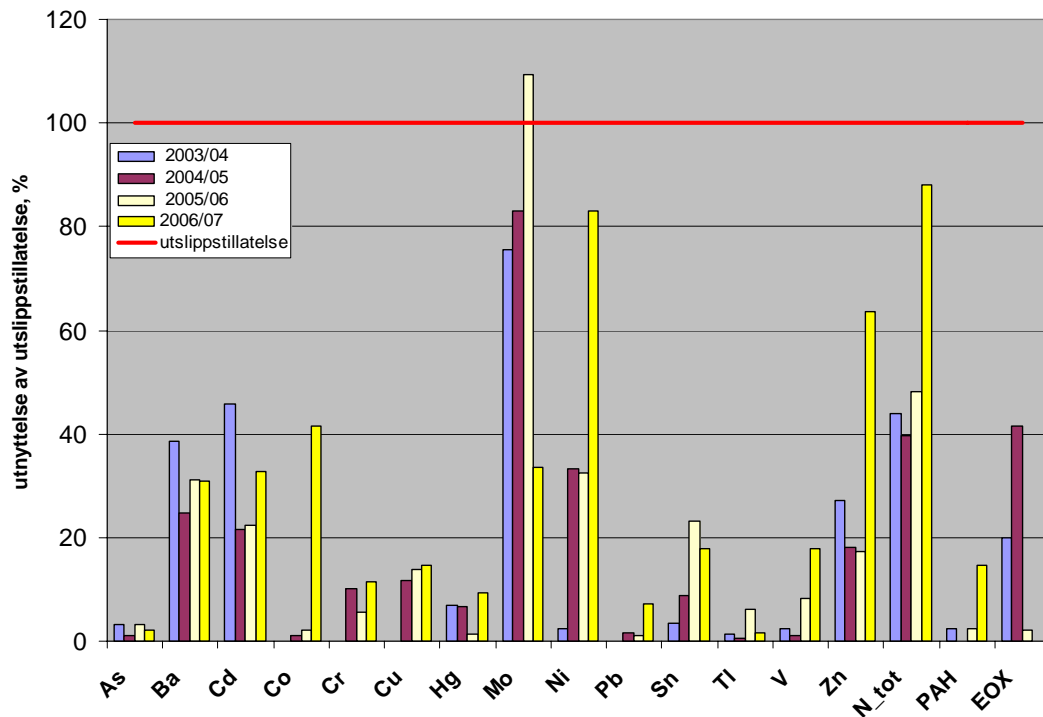
Figur 1. Utslipp fra NOAH-Langøya i perioden oktober til september for 2003/2004, 2004/2005, 2005/2006 og 2006/2007. Utslipp av den enkelte komponent er oppgitt som prosent utnyttelse av konsesjonsbestemte maksimalutslipp og er beregnet på bakgrunn av analyserte mengder i utslippsvannet; arsen (As), barium (Ba), kadmium (Cd), kobolt (Co), krom (Cr), kobber (Cu), kvikksølv (Hg), molybden (Mo), nikkel (Ni), bly (Pb), tinn (Sn), vanadium (V), sink (Zn), total-nitrogen (N(tot)), tjærestoffer (PAH) og summen av ekstraherbare klorerte organiske forbindelser (EOX). Etter figur fra NOAH Langøya.
