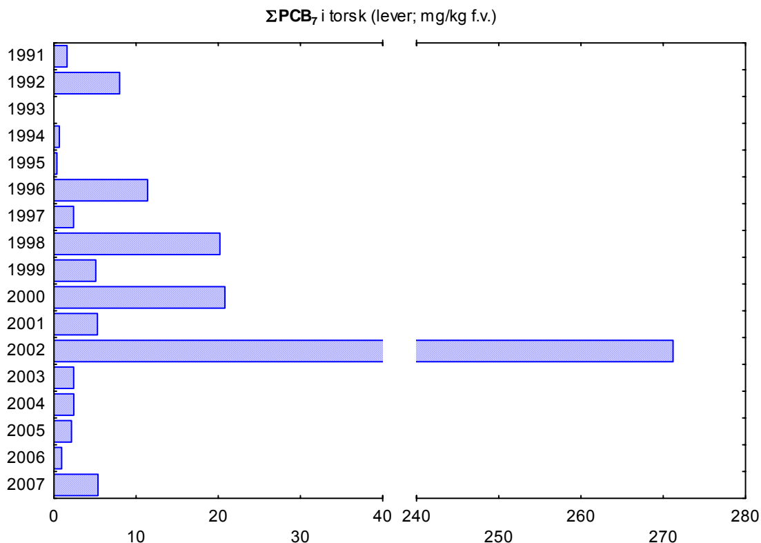
Figur 26. Gjennomsnitt av \Sigma PCB_7 i lever av torsk fra indre Sør fjorden (1991-2007), mg/kg fettvekt . Verdiene er også gjengitt i Tabell 10. Mrk. brudd på akse mellom 40 og 240.
