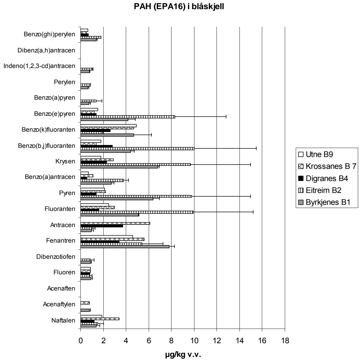
Figur 30. Konsentrasjoner ( \mu\text{g}/\text{kg} våtvekt) av polysykliske aromatiske hydrokarboner (PAH) i blåskjell fra stasjonsnettet i Sør fjorden, 2007. Median av 3 replikater på stasjon B1 (Byrkjenes) og stasjon B2 (Eitrheim). Standard avvik er angitt for disse.
