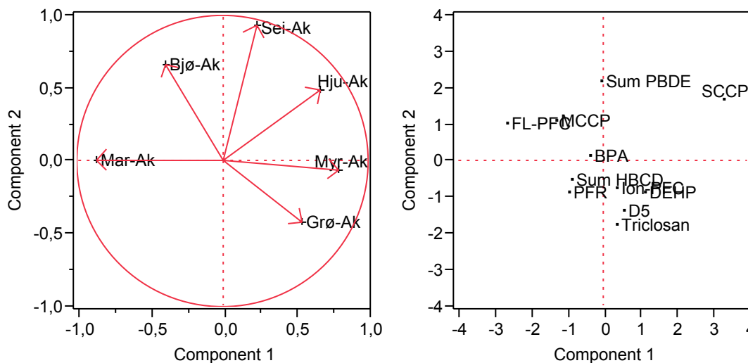
Figur 28. Loading- og scoreplot basert på PCA-analyse av konsentrasjoner av utvalgte miljøgifter i Akerselva. Stasjonene er identifisert ved stasjonskodene. Med unntak av flyktige PFC (FL-PFC) og ioniske PFC (Ion-PFC) er samme forkortelse som tidligere benyttet.
