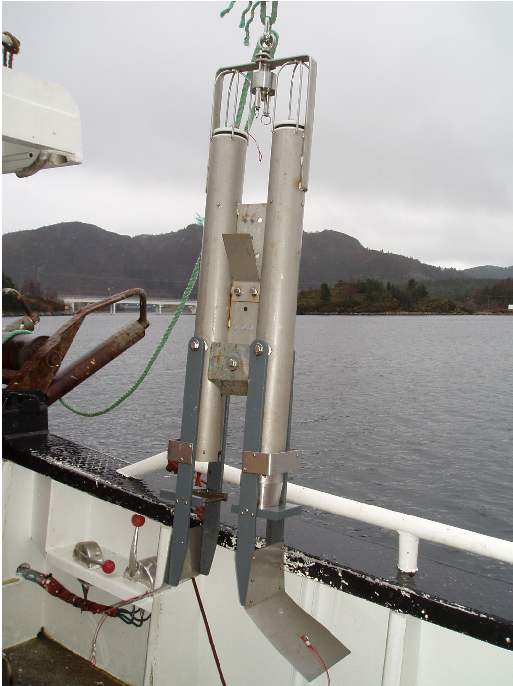
Figur 3. Geminicorer. (Indre rør kun i den ene holderen). (Foto: John Arthur Berge)
