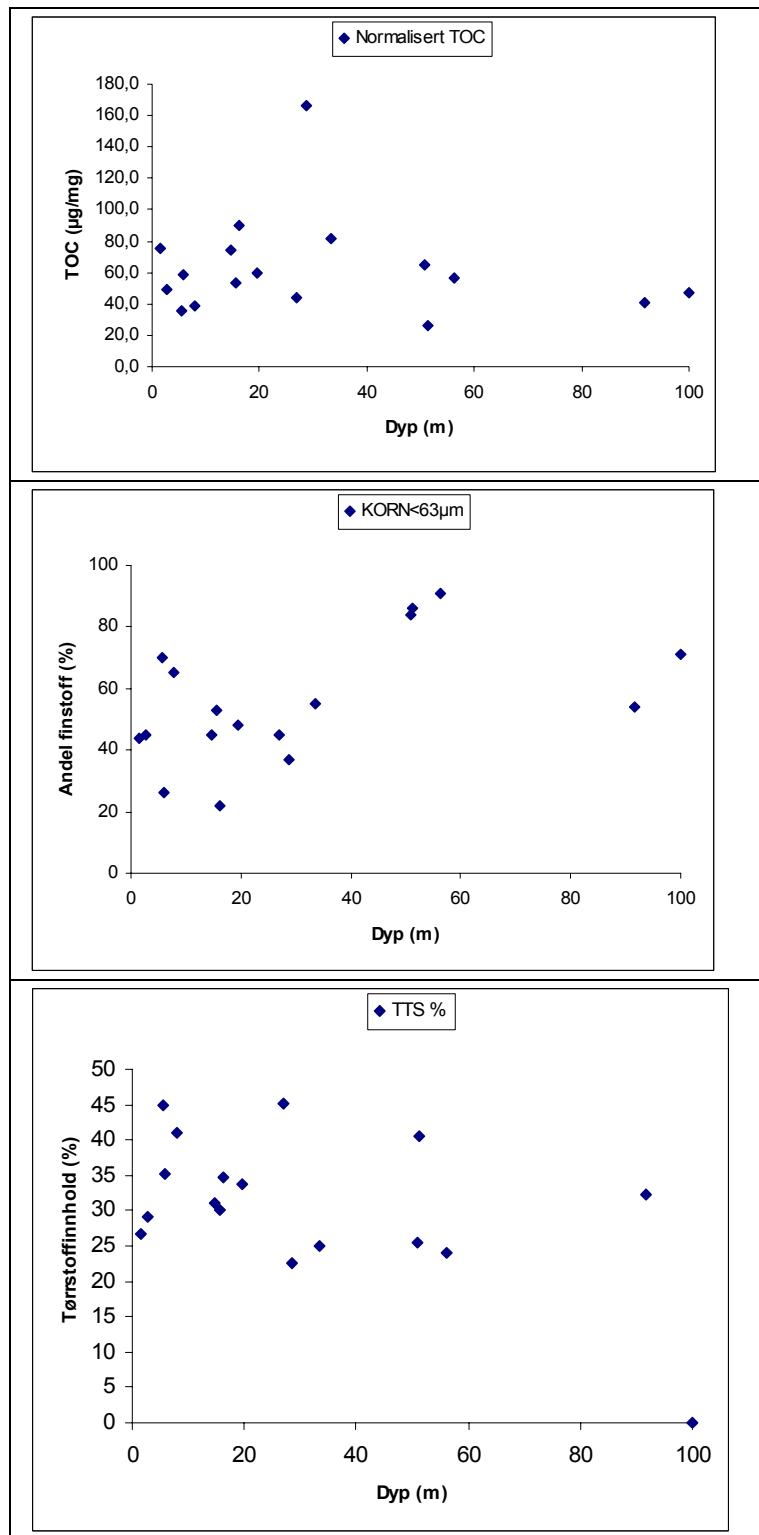
Figur 6. Organisk innhold (TOC normalisert, µg/mg), andel finfraksjon (Korn<63 µm) og tørrstoffinnhold (TTS %) i overflatesediment som funksjon av bunndyp på prøvetakingsstedet.
