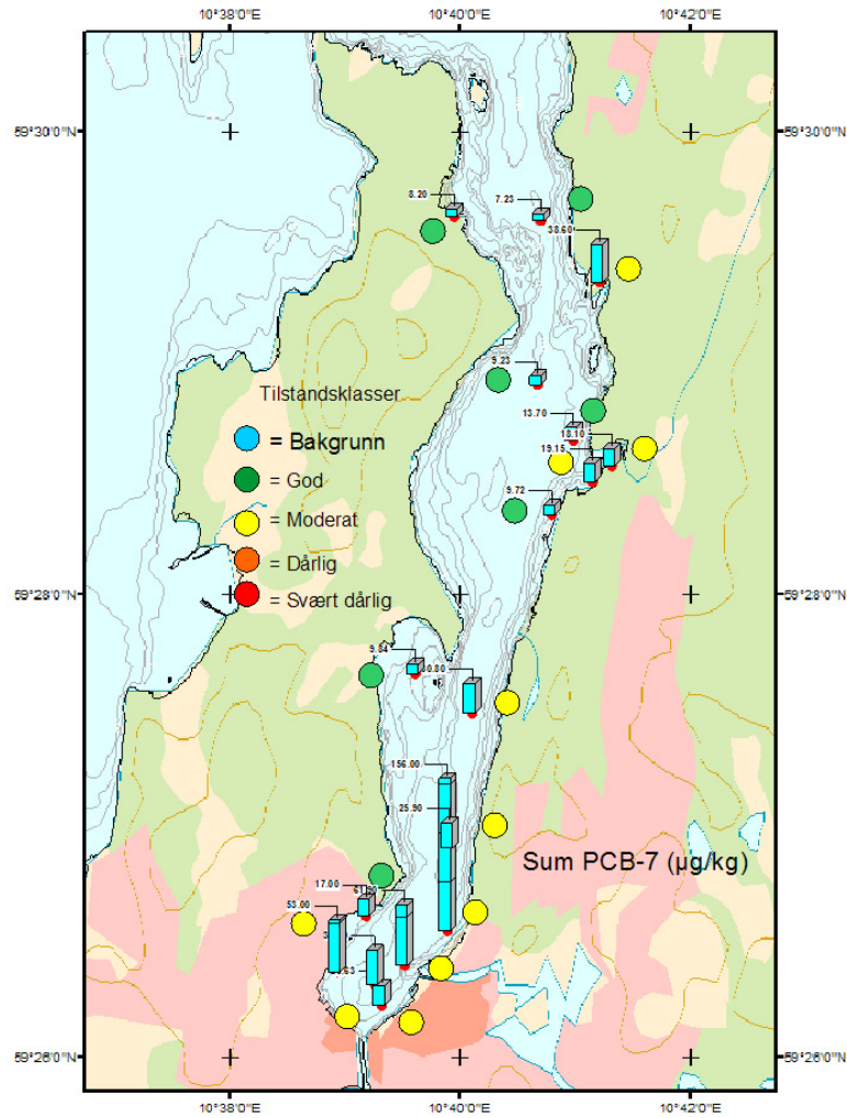
Figur 11. Konsentrasjonen av polyklorerte bifenyler ( \Sigma PCB 7 ) i sediment vist som stolpediagram. Stolpediagramme er plassert i kartet på posisjonen hvor prøven er tatt. For hvert stolpediagram er det plassert et farget punkt som markerer sedimentets tilstand klassifisert i henhold til SFTs miljøkvalitetskriterier basert på effekter (TA-2229/2007).
