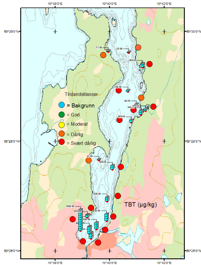
Figur 9. Konsentrasjonen av tributyltinn (TBT) i sediment vist som stolpediagram. Stolpediagrammet er plassert i kartet på posisjonen hvor prøven er tatt. For hvert stolpediagram er det plassert et farget punkt som markerer sedimentets tilstand klassifisert i henhold til SFTs miljøkvalitetskriterier basert på effekter (TA-2229/2007).
