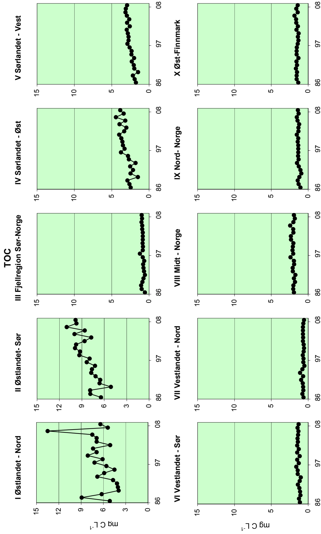
Figur 20. Trender i TOC (total organisk karbon) for perioden 1986-2008 for innsjøer i de 10 regionene.
