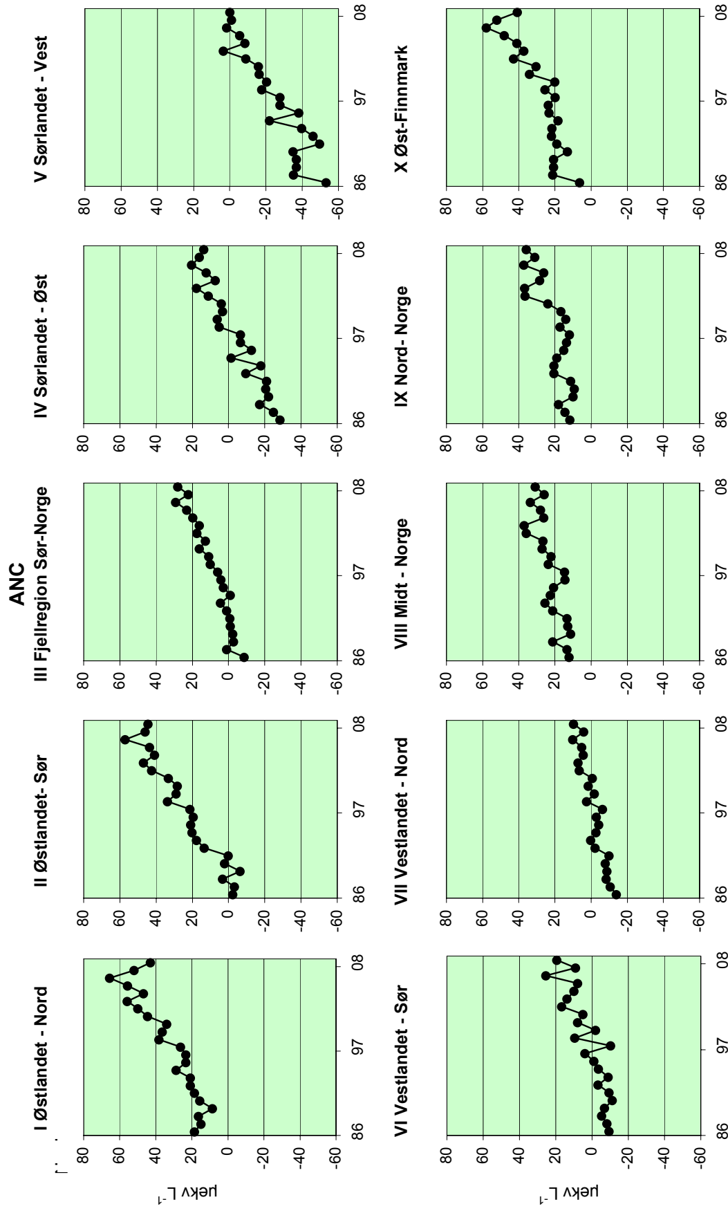
Figur 17. Trends for perioden 1986-2008 for ANC (syrenøytraliserende kapasitet) for innsjøer i de 10 regionene.
