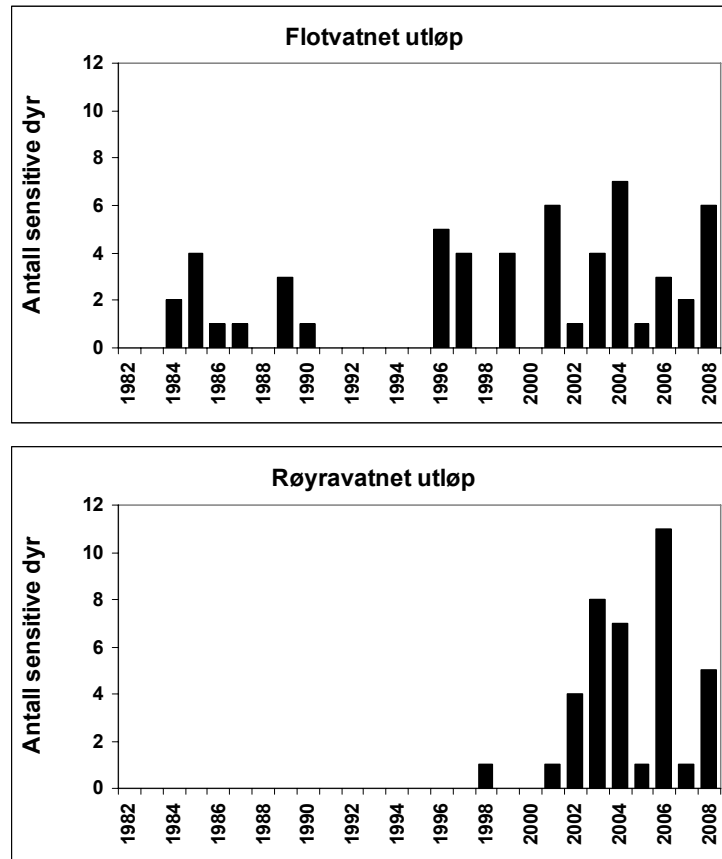
Figur 23. Forekomst av forurensningssensitive bunndyr i utløpselvene fra Flotvatnet og Røyrvatnet, Vikedal, i perioden 1982-2008.
