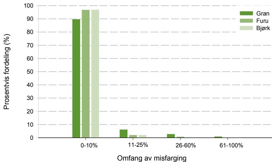
Figur 42. Omfang av misfarging i de forskjellige klassene, i hht. ICP Forests standard metode.
