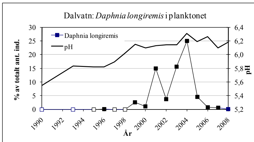
Figur 26. Andel (% av totalt individtall) av vannloppen Daphnia longiremis i Dalvatn (Reg. X, Øst-Finnmark) i 1990-2008. Åpne symboler: ingen funn av dafnier i planktonprøver. pH fra høstprøver i samme periode.
