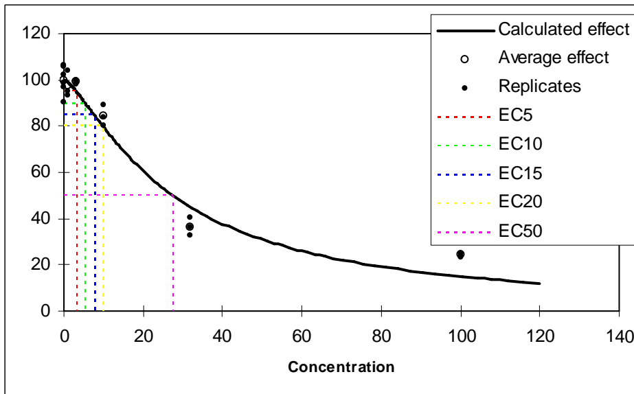
Fig.:2 Effekt av avløpsvann på veksthastigheten til Pseudokirchneriella subcapitata . Stiplede linjer viser fra venstre EC, økende effekt nivåer
