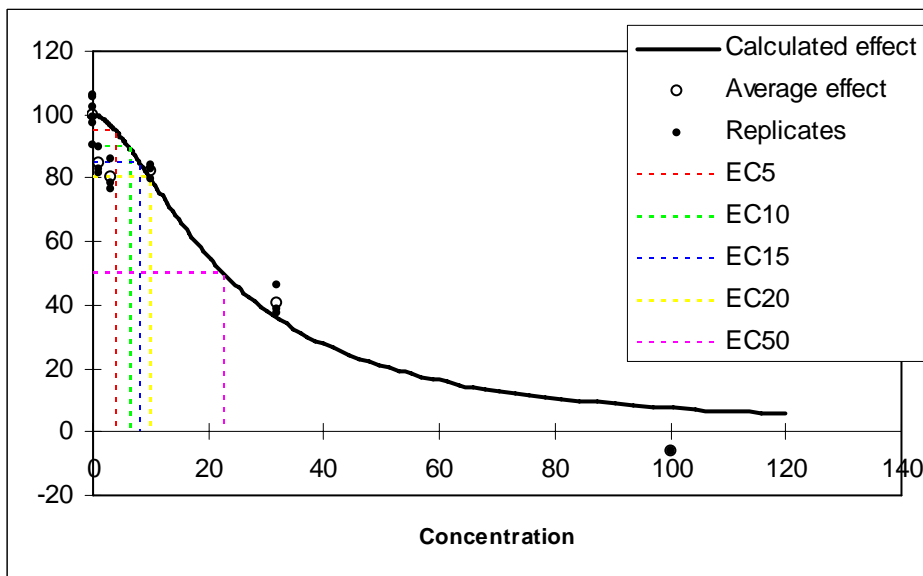
Fig.:2 Effekt av avløpsvann på vekststigheten til Pseudokirchneriella subcapitata . Stiplede linjer viser (fra venstre) EC 10 og EC 50 .
