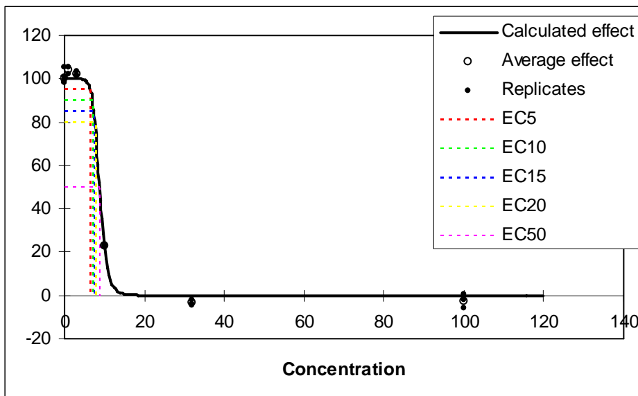
Fig.:2 Effekt av avløpsvann på veksthastigheten til Pseudokirchneriella subcapitata . Stiplede linjer viser (fra venstre) de ulike EC effekt nivåer
