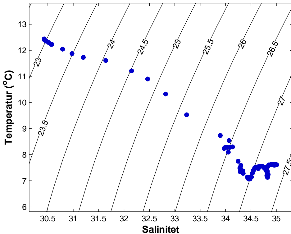
Figur 10. T/S-diagram for hydrografiprofilen ved Haugneset 11. juni 2009. De tynne svarte linjene er isolinjer for lik densitet (enhet: \text{kg/m}^3 \cdot 1000 ).
