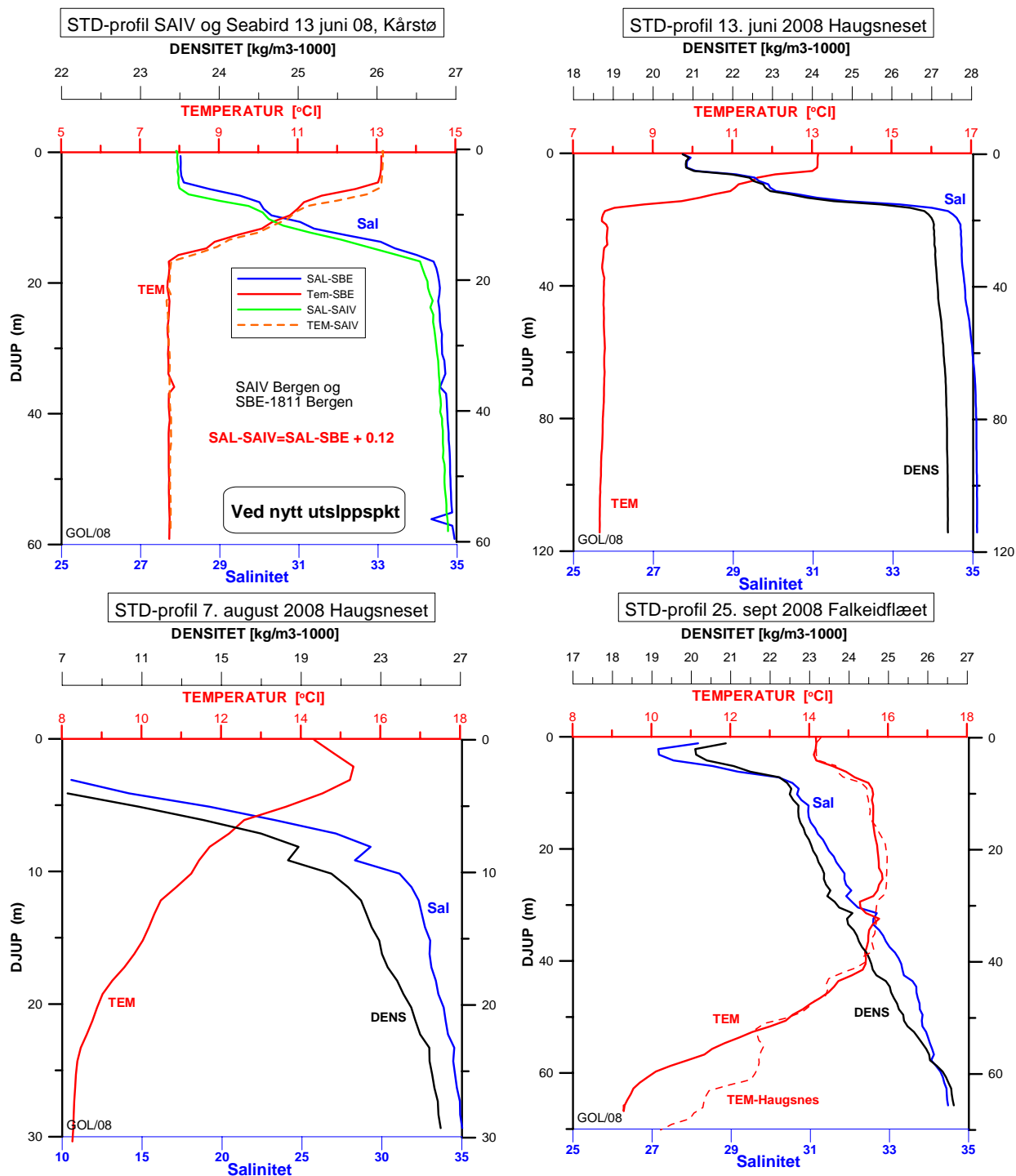
Figur 7. Målte vertikale profiler av sjøens temperatur, salinitet og densitet (beregna) den 13. juni, 7. august og 25. september 2008. Merk ulik skala i de fire figurene både for dyp og målevariable.
