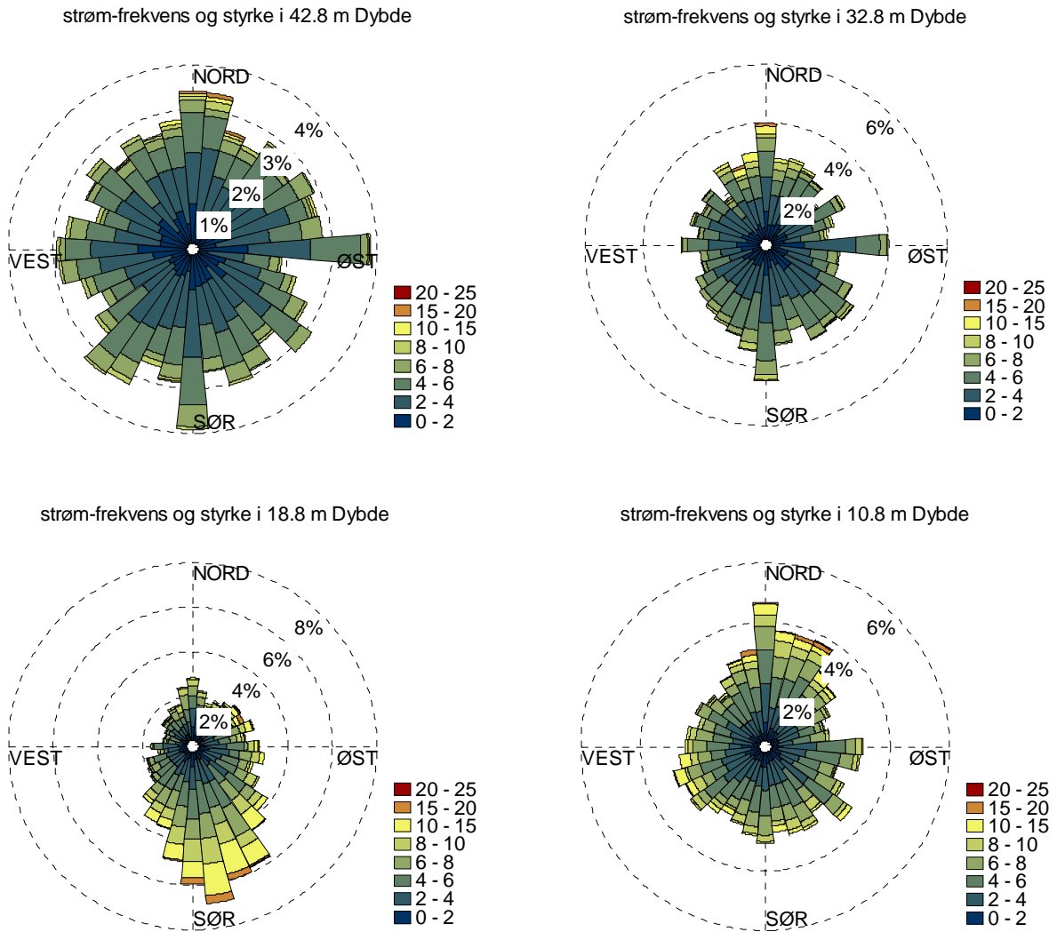
Figur 20: Strømroser for fire utvalgte dyp i 4. måleperiode. Lengden på stolpene angir hvor stor del av målingene som er innafor den gitte retningen. Fargene angir strømfartfordelingen (cm/s) innafor den gitte retningen.
