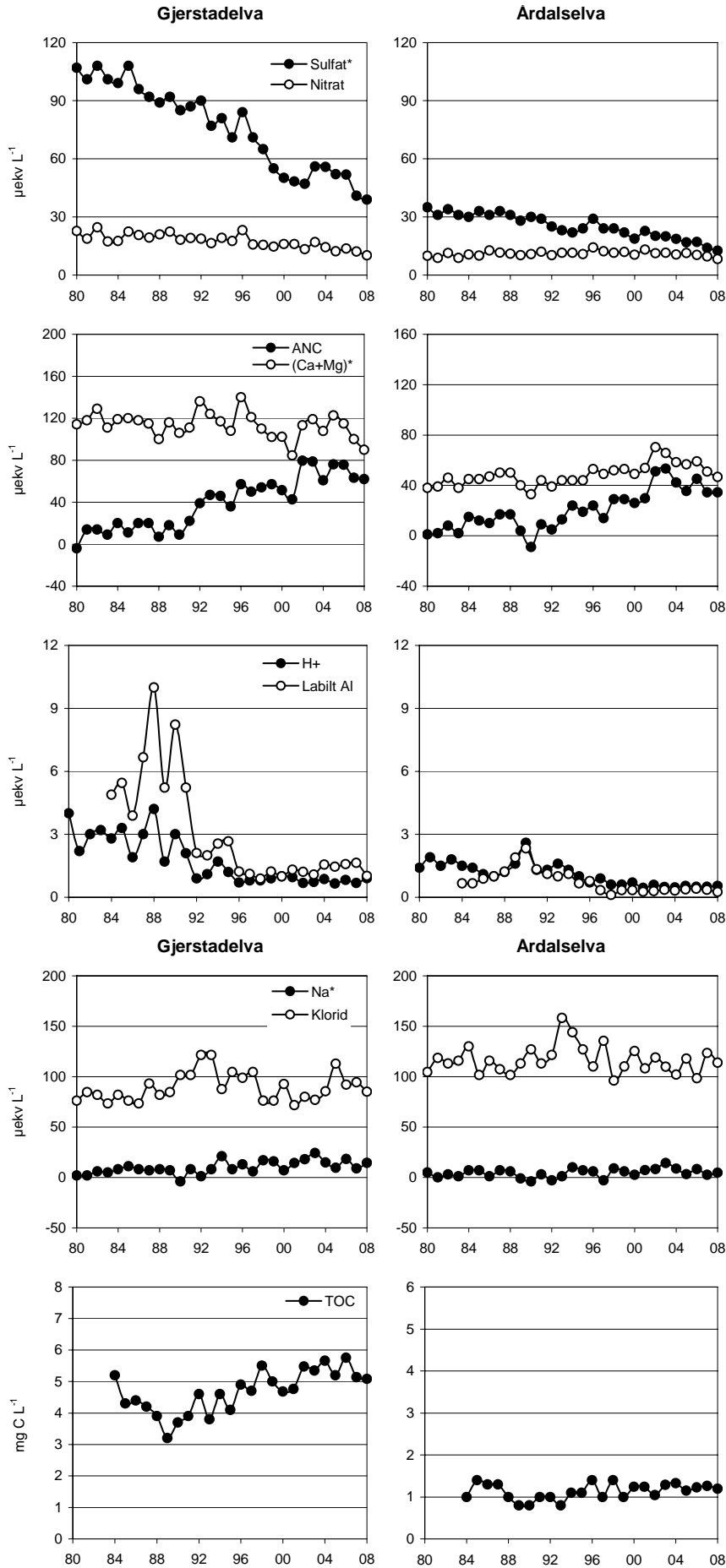
Figur 36. Årsmiddelverdier av utvalgte parametre i Gjerstadelva og Ardalselva for perioden 1980-2008.
