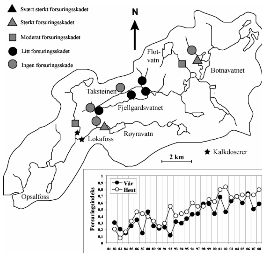
Figur 69. Oversikt over innsamlingslokaliteter og sammensetning av bunndyr i Vikedalsvassdraget i 2008. Figuren viser også gjennomsnittlige forsuringssverdi vår (V) og høst (H) i perioden 1982-2008. Kalkdoserere er merket stjerne.
