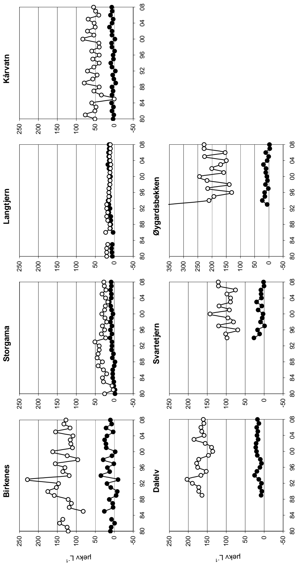
Figur 40. Klorid og ikke-marin natrium i feltforskningsstasjonene. Ikke-marin natrium ● og klorid ○. Enhet: µekv L -1 . OBS! Skala Øygardsbekken.
