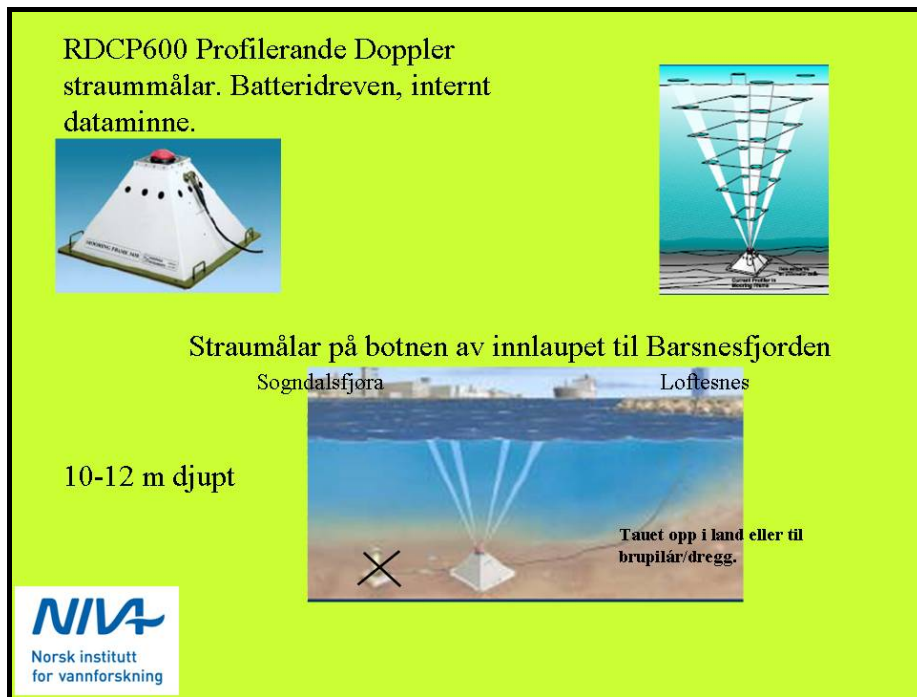
Figur 11. Opplegg for måling av strøm med profilerande Doppler (ADCP) målar.
