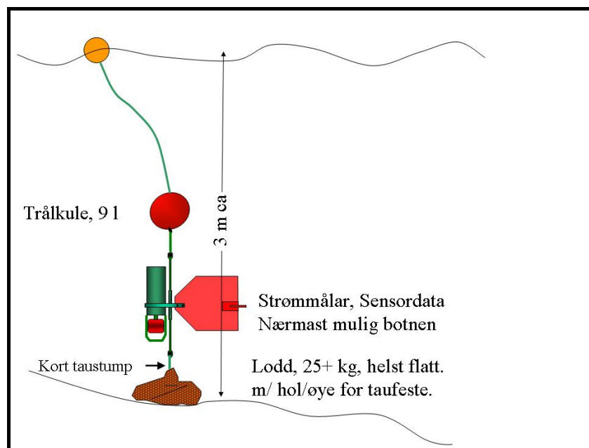
Figur 12. Illustrasjon av Sensordata strømmålaren og opphenget. Denne riggen stod litt sør for fyllinga ved Loftesnes.
