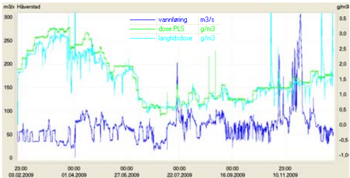
Figur 5. Vannføring, PLS-dose (styringssignal som dose) og langtidsdose ved Håverstad doseringsanlegg i 2009. (Januar er ikke med, da mangler logg). Det er godt samsvar mellom styringssignalet som PLS dose og langtidsdose, særlig siste halvdel av året.
