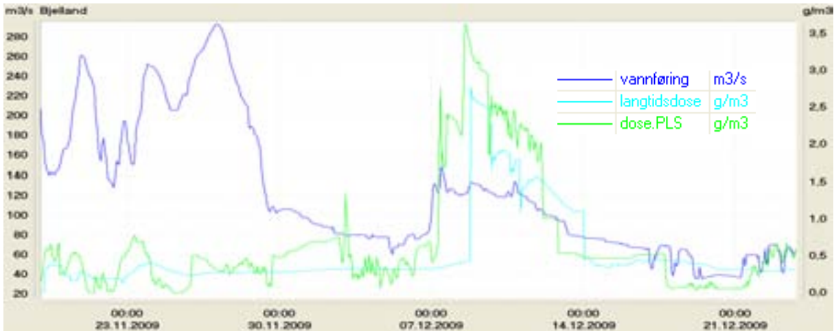
Figur 11. Vannføring, langtidsdose og PLS-dose på Bjelland doseringsanlegg fra 19. november og ut året 2009. Det var stor forskjell i avgitte doser ved flomperioden i november kontra flommen i desember.
