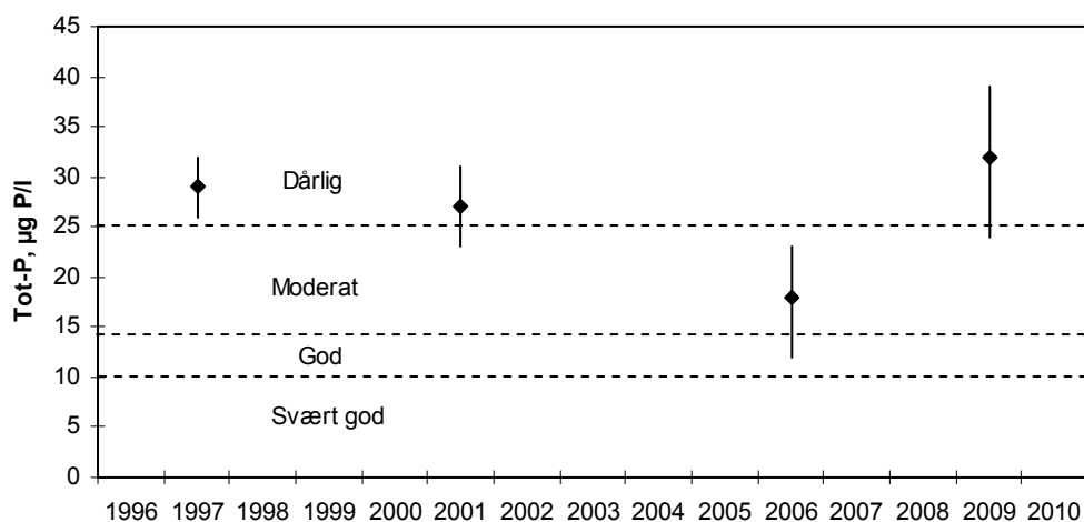
Figur 10. Konsentrasjoner av tot-P i Stavsjøen (0-5 m) i 1997, 2001, 2006 og 2009. Figuren viser middelværdier og variasjonsbredder de enkelte årene. Tilstandsklasser i henhold til Veileder 01:2009 (grenseverdier for kalkrike, klare innsjøer i lavlandet).
