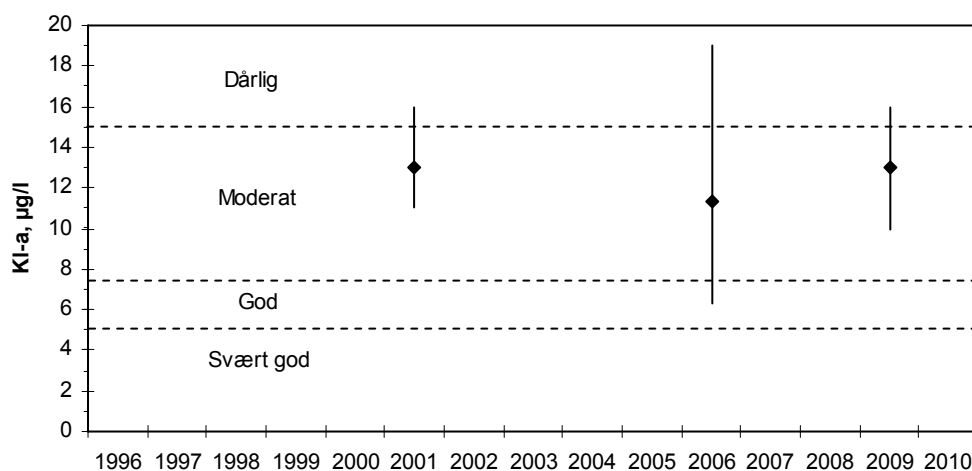
Figur 13. Algemengder i Stavsjøen i 2001, 2006 og 2009, målt som klorofyll- a i epilimnion (0-5 m). Figuren viser middelværdier og variasjonsbredder. Intervaller for de ulike tilstandsklassene er også vist (grenseverdier for kalkrike, klare innsjøer i lavlandet).
