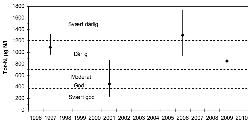
Figur 11. Konsentrasjoner av tot-N i Stavsjøen (0-5 m) i 1997, 2001, 2006 og 2009. Figuren viser middelværdier og variasjonsbredder. Tilstandsklasser i henhold til Veileder 01:2009 (grenseverdier for kalkrike, klare innsjøer i lavlandet).
