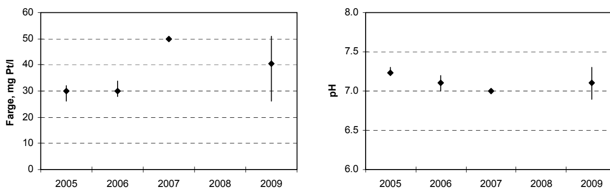
Figur 1. Farge og pH i Næra i 2005-2007 og 2009 (0-10 m). Figurene viser middelverdier og variasjonsbredder de enkelte årene. Kun én observasjon i 2007.
