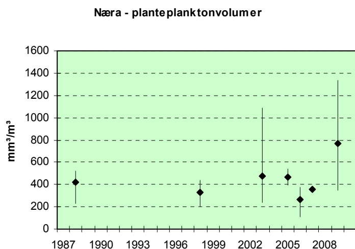
Figur 8. Tidsutvikling i totalvolumer av planteplankton i Næra. Figuren viser middelveier og variasjonsbredder (kun én observasjon i 2007).
