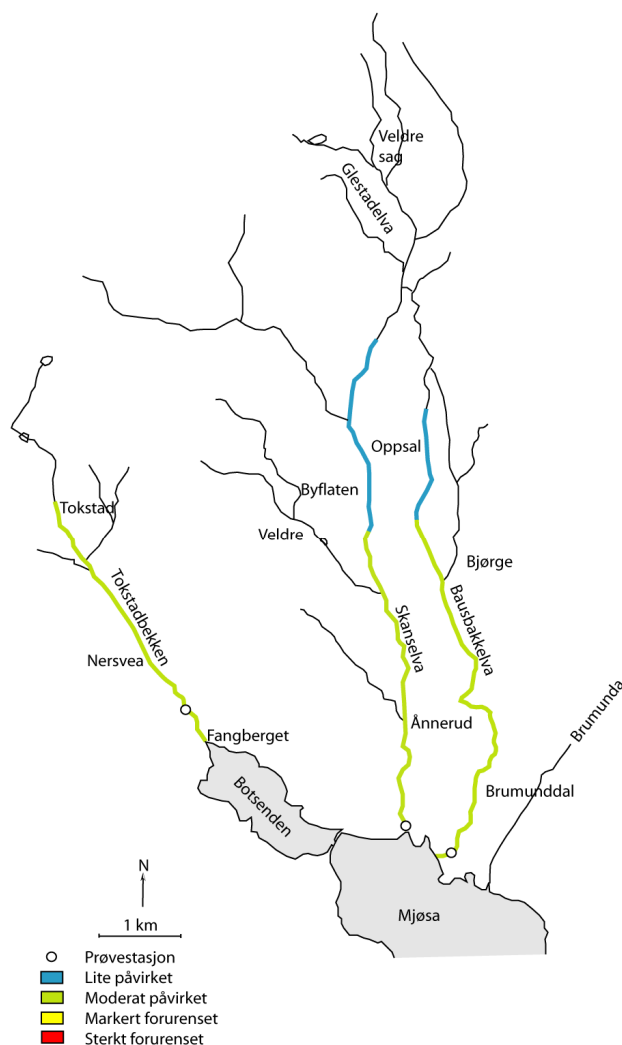
Figur 17. Miljøtilstanden i tre bekker/elver i Ringsaker i september 2009, vurdert ut fra biologiske feltobservasjoner.
