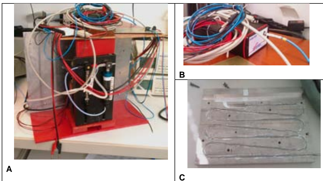
Figur 56. Konstruert i GKSS enheten for gang ombord pH målinger. A- main block with two syringes for addition of dye (front side), photometer (on top) and flow cell (back side), B – photometer, C – thermostated flowcell. A-hovedbygning med sprøyter for tilsetning av fargestoff (front side), fotometeret (øverst) og flow cell (baksiden), B - fotometeret, C - thermostated flowcell.
