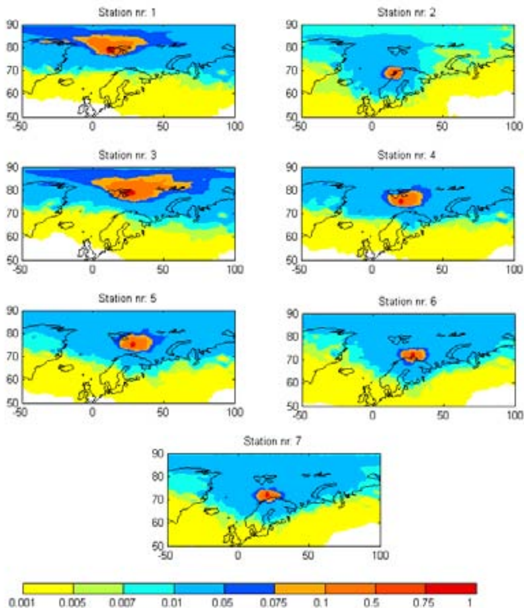
Figur 62. Fotavtrykkskart som viser gjennomsnittlig utslipps sensitivitet (ES) (0-100 m) for luft [ \text{ng}/\text{m}^3 ] representert med PCB- 28 tracer og gjennomsnitt for alle syv lokaliteter for stasjonene 1-7, hele 2007.
