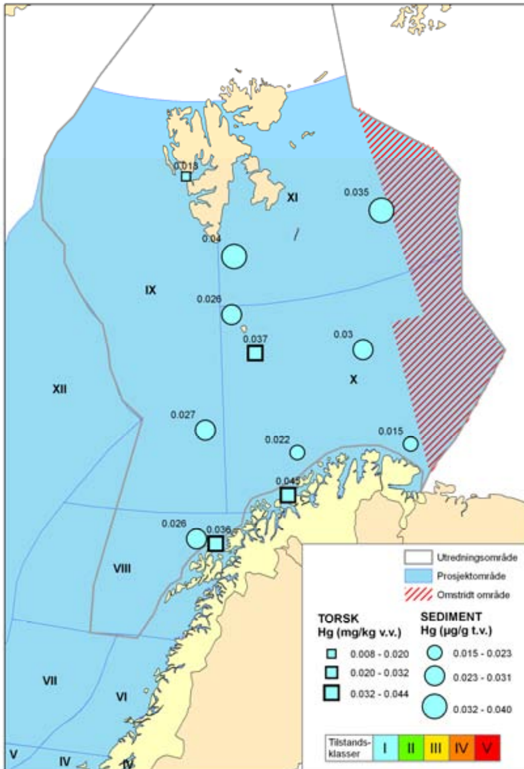
Figur 26. Gjennomsnittskonsentrasjoner av kvikksølv i overflatesediment (mg/kg tørrvekt) og i torskefilet (mg/kg våtvekt) i 2009. Tilstandsklassene gjelder sediment.
