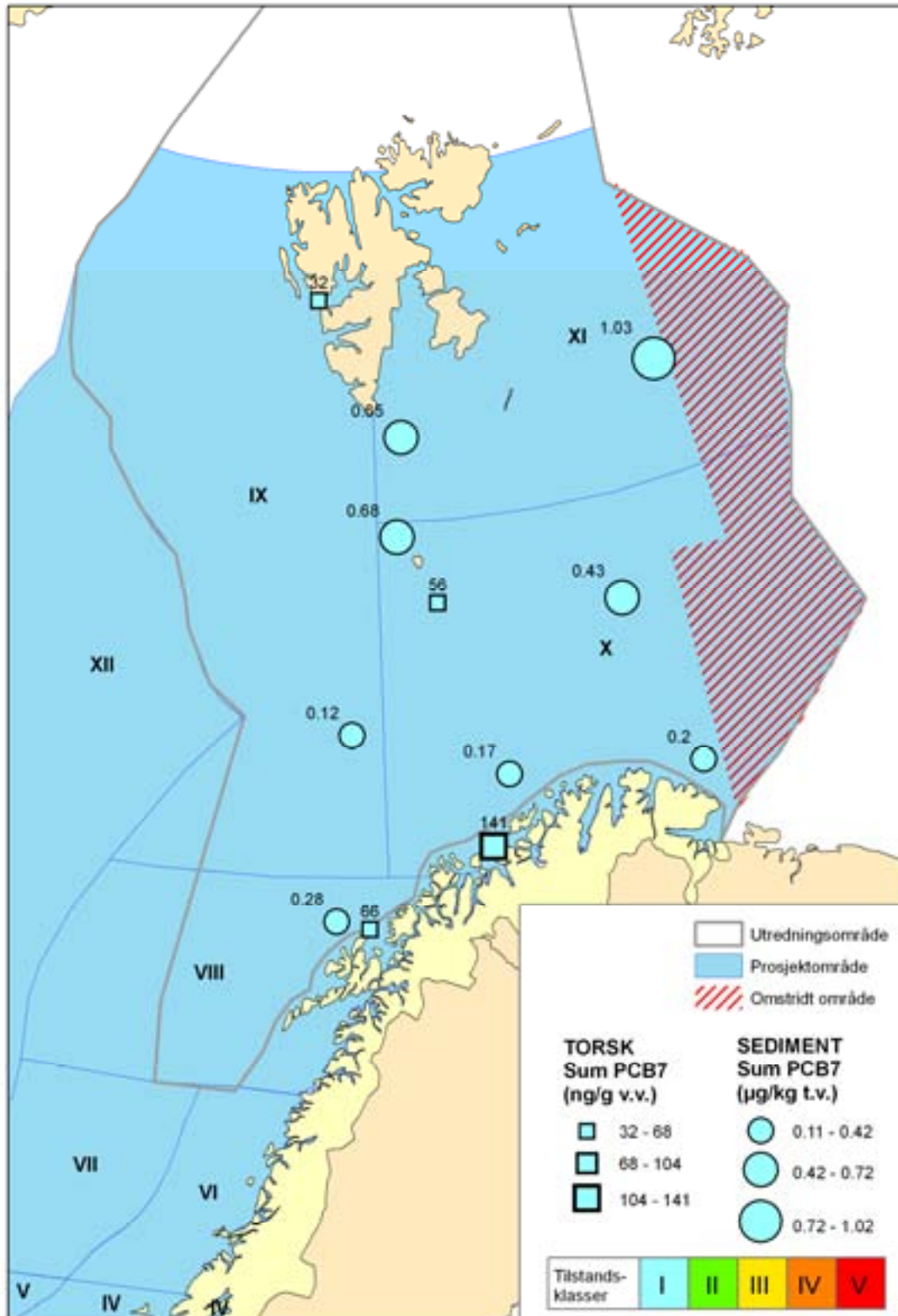
Figur 31. Gjennomsnittskonsentrasjoner av PCB i overflatesediment ( \mu\text{g}/\text{kg} tørrvekt) og i torskelever ( \mu\text{g}/\text{kg} våtvekt) i 2009.
