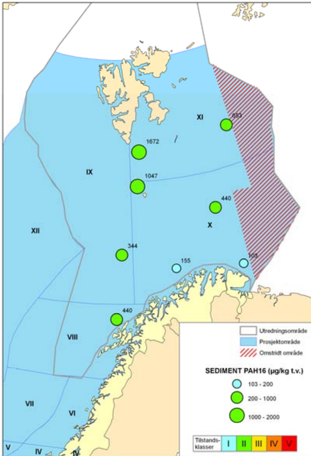
Figur 34. Gjennomsnittskonsentrasjoner av PAH i overflatesediment (µg/kg tørrvekt) i 2009.
