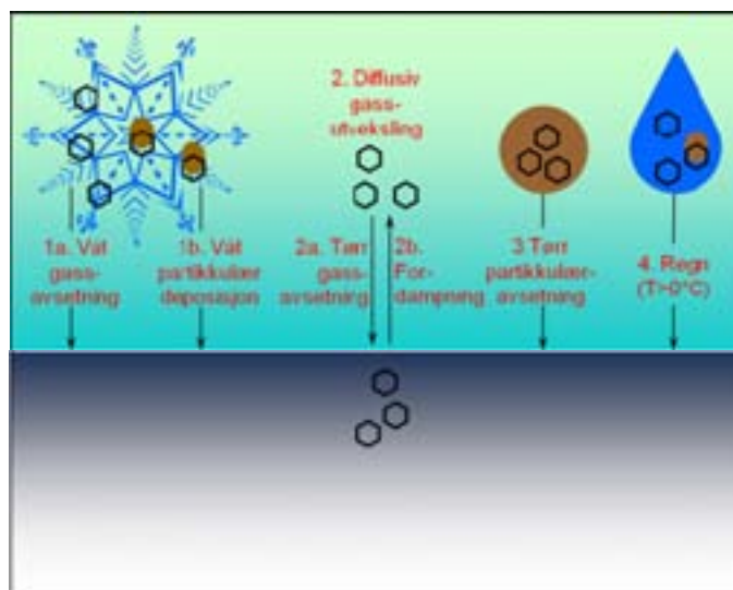
Figur 5. Prosesser som er bestemmende for avsetning og utveksling av organiske miljøgifter mellom luft og hav (modifisert etter Daly og Wania, 2004).
