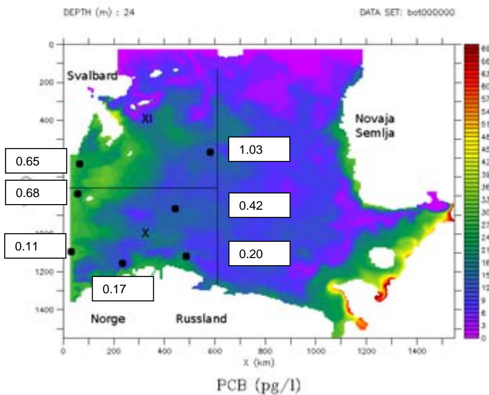
Figur 24. Konsentrasjoner av arsen (As) og PCB i bunnvann (pg/l, beregnet for en intens sirkulasjon) og i sediment (hhv. mg/kg t.v. og µg/kg t.v., stasjonsposisjon markert med svart sirkel). Konsentrasjonsskala er vist i figurens høyre kant.
