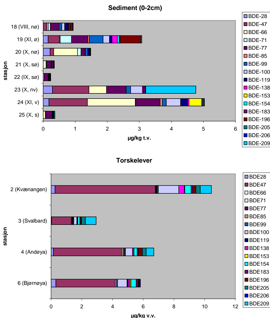
Figur 37. Gjennomsnittskonsentrasjoner av de forskjellige PBDE forbindelser i overflatesediment (µg/kg tørrvekt) og i torskelever(µg/kg våtvekt) i 2009. Innen for parenteser er det angitt region og posisjon innen regionen (sediment) eller stedsnavn (torsk).
