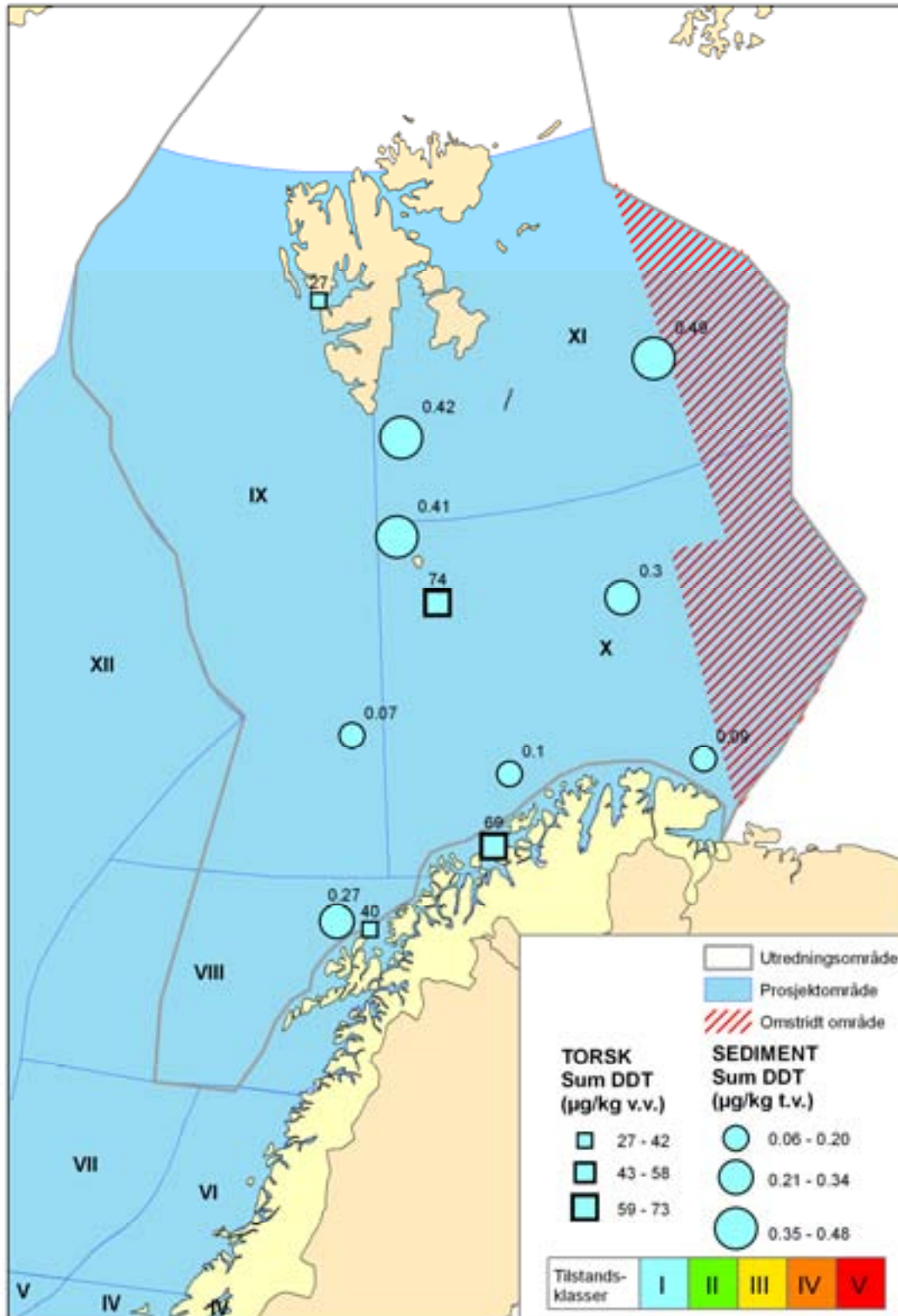
Figur 32. Gjennomsnittskonsentrasjoner av sum DDT i overflatesediment ( \mu\text{g}/\text{kg} tørrvekt) og i torskelever ( \mu\text{g}/\text{kg} våtvekt) i 2009.
