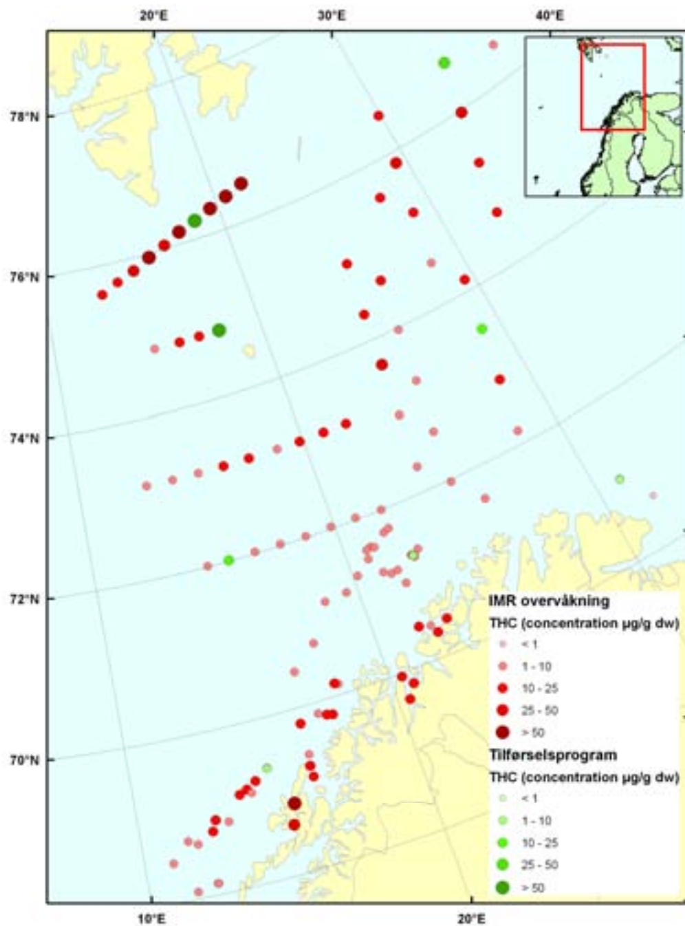
Figur 53. THC nivåer i overflatesedimenter fra Barentshavet, µg/g tørrvekt. Røde punkter viser resultatene fra Havforskningsinstituttets overvåkningsprogram 2003-2008, mens grønne punkter viser resultatene fra Tilførselsprogrammets prøvetaking i 2009.
