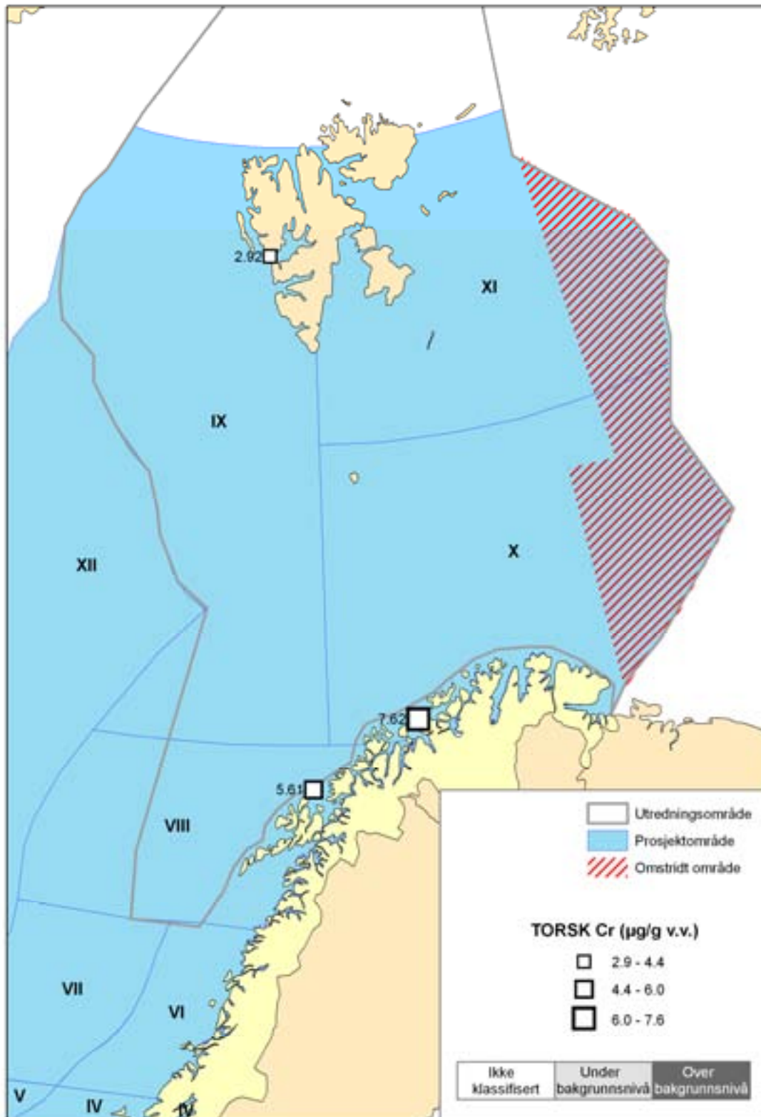
Figur 29. Gjennomsnittskonsentrasjoner av krom i torskelever (mg/kg våtvekt) i 2009. (Krom ble ikke undersøkt i torsk ra Bjørnøya (st.6).
