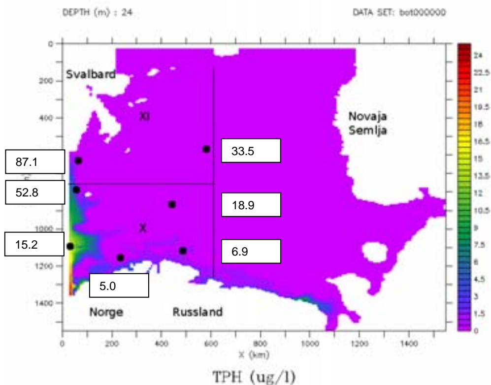
Figur 25. Konsentrasjoner av PAH (fg/l = femtogram/l = 10^{-15} g pr.liter) og olje (TPH, her sammenlignbart med THC) ( \mu\text{g/l} ) i bunnvann (beregnet for en intens sirkulasjon) og konsentrasjoner av PAH ( \mu\text{g/kg t.v.} ) og olje (THC, \text{mg/kg t.v.} ) i sediment (stasjonsposisjon merket med svart sirkel). Konsentrasjonsskala er vist i figurens høyre kant.
