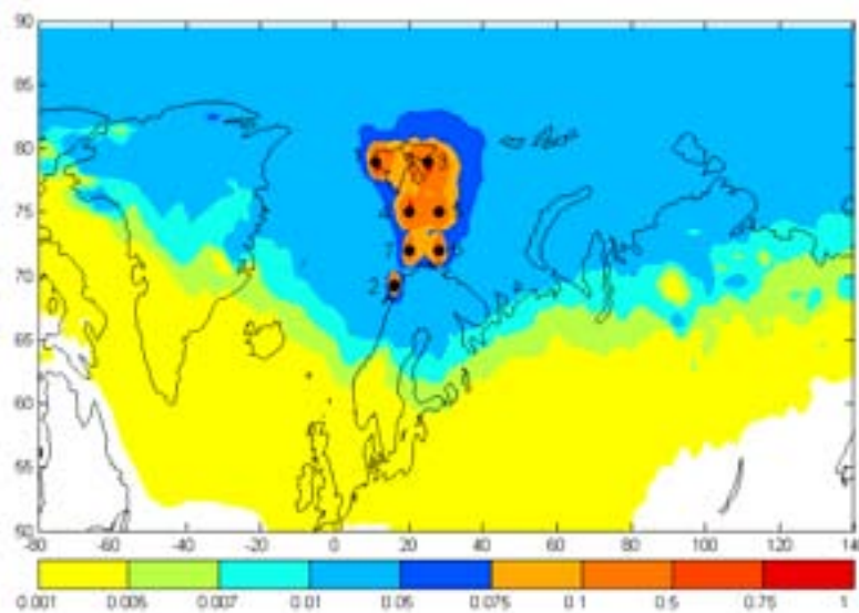
Figur 60. Fotavtrykkskart som viser gjennomsnittlig utslippssensitivitet (ES) (0-100 m) for luft [ \text{ns}/\text{m}^3 ] representert med PCB- 28 tracer og gjennomsnitt for alle syv lokaliteter for hele 2007.
