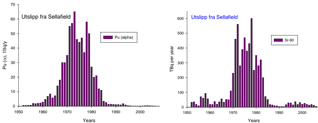
Figur 11. Årlig utslipp av strontium-90 og plutonium-239+240 fra Sellafield-anlegget til Irskehavet (Jackson et al. 2000; Vives i Baille et al. 2007).
