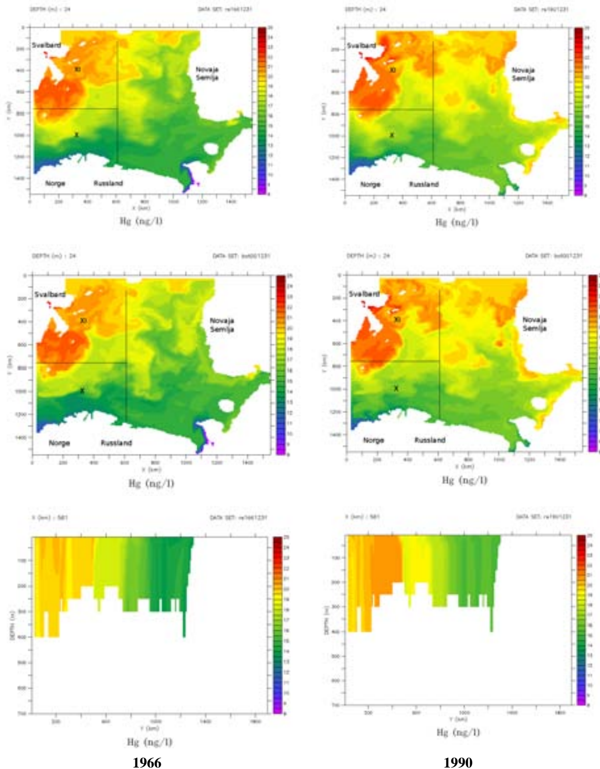
Figur 14. Beregnede konsentrasjoner av kvikksølv (ng/l) i 24m dyp (øverst), i bunnvann (midten) og transekt (overflate-bunn) langs den østre grense til Regionene XI og X fra nord til syd (nederst). Beregningene gjelder for svak sirkulasjon (1966) og intens sirkulasjon (1990).
