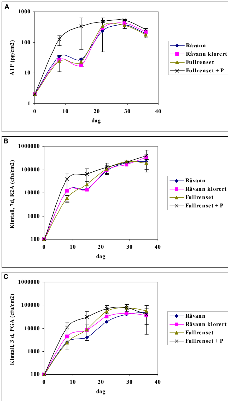
Figur 1. Utvikling av biofilm i rørene med ulik vannkvalitet målt som ATP (figur A), kimtall 7 døgn R2A (figur B) og kimtall 3 døgn PGA (figur C). Hvert punkt er gjennomsnittsverdi for 3 parallelle rør ± standardavvik for fullrenset og fullrenset + P, og for 2 parallelle rør med råvann og klorert råvann.
