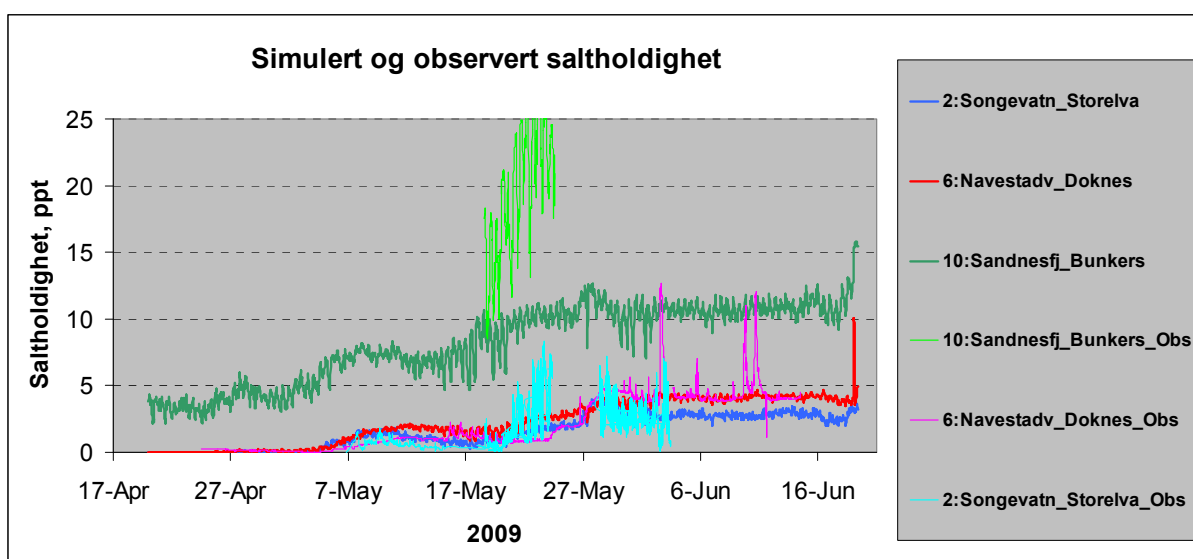
Figur 21. Simulert og observert saltholdighet 2009 i overflaten, tidsserie
