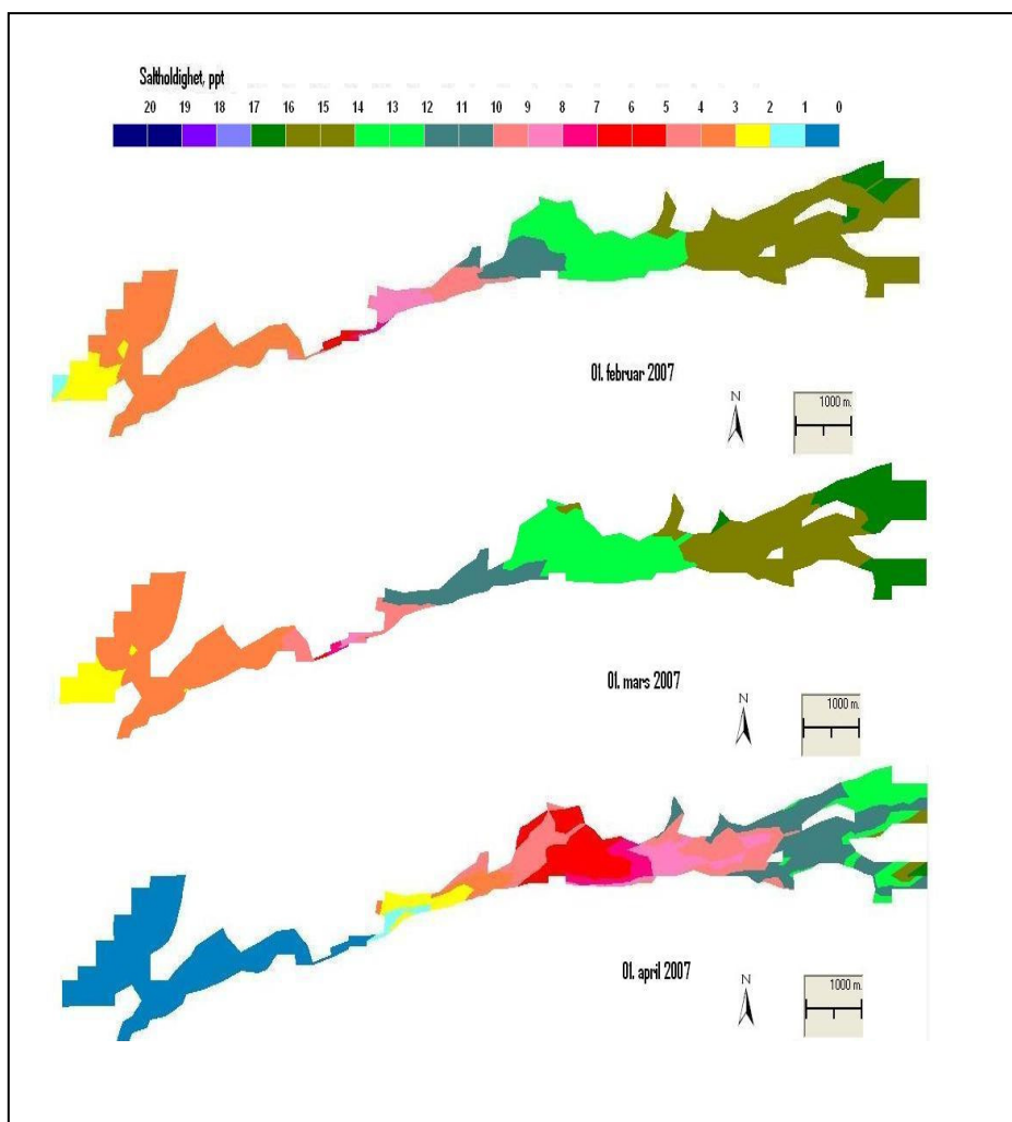
Figur 17. Simulert saltholdighet i overflaten
