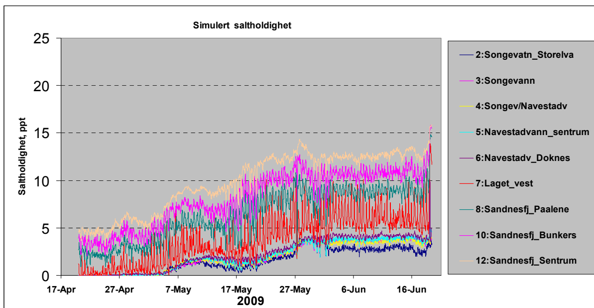
Figur 23. Simulert saltholdiget 2009 i overflaten, tidsserie
