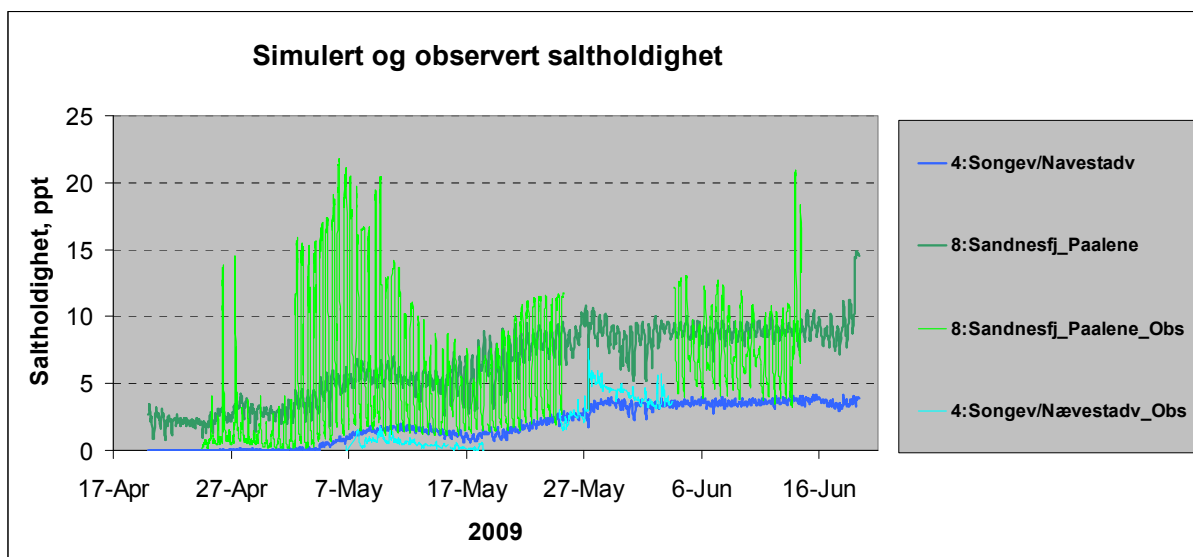
Figur 22. Simulert og observert saltholdiget 2009 i overflaten, tidsserier
