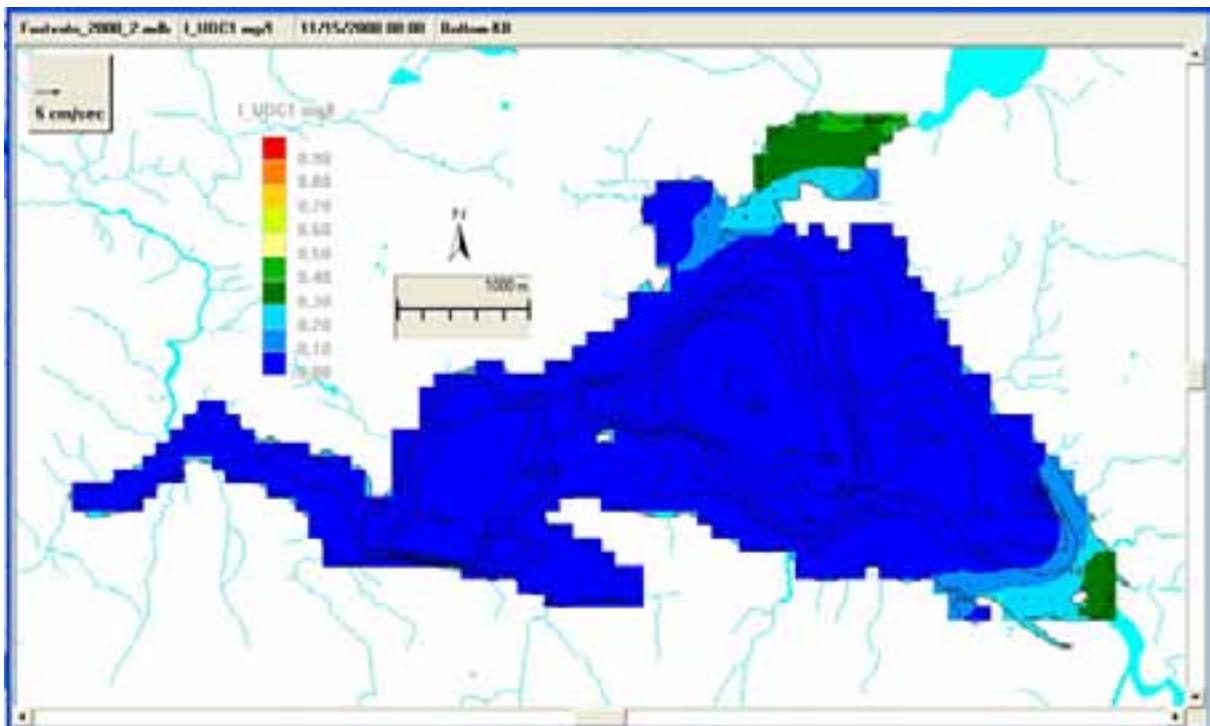
Figur 32. 15. november. Konsentrasjoner på bunnen. Kontinuerlig dosering i bekketilløpene fra 1. september av 5 % rotenonholdig væske svinrate.
