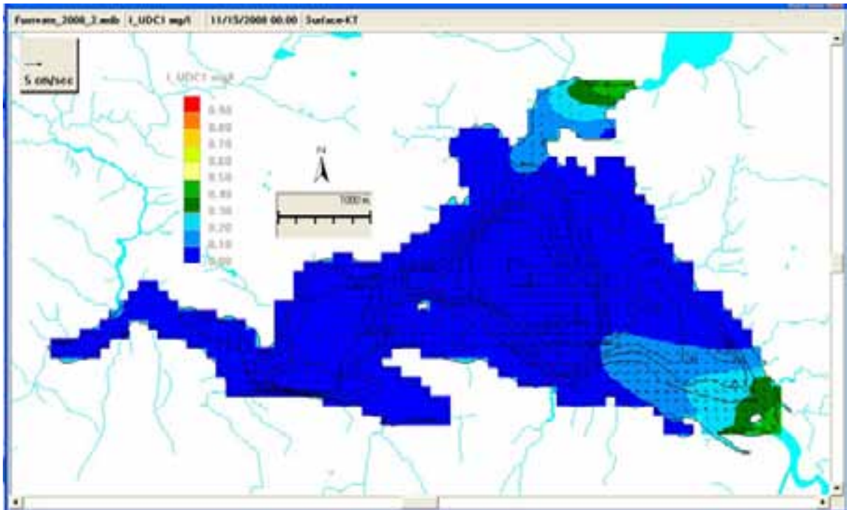
Figur 31. 15. november. Konsentrasjoner på overflaten. Kontinuerlig dosering i bekketilløpene fra 1. september av 5 % rotenonholdig væske med svinrate.
