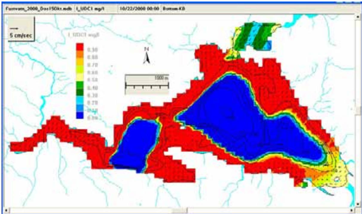
Figur 9. Dosert 15. oktober 2008 kun på overflaten. I de dypeste områdene ble konsentrasjonene for lave.
