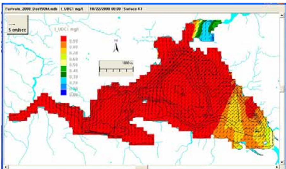
Figur 8. Dosert 15. oktober 2008 kun på overflaten. I overflaten ble konsentrasjonene tilfredsstillende høye.
