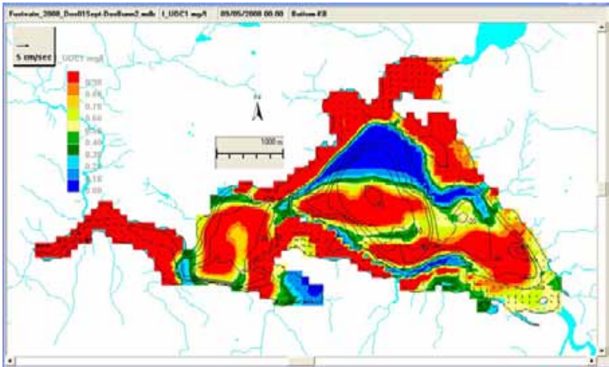
Figur 21. Konsentrasjoner langs bunnen. Dose 1. september. Ekstra dosering mellom 20 m og bunnen over de dypeste delene av innsjøen resulterte i at det meste av de dypeste områdene fikk tilfredsstillende konsentrasjoner.
