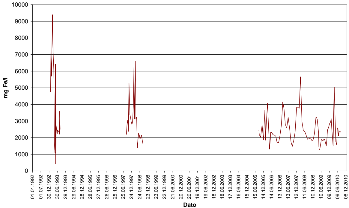
Figur 15. Jernobservasjoner ved stasjon C, Drensgrøft i Gammelgruva, 1992-2010.
