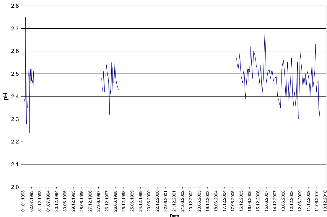
Figur 13. pH-observasjoner ved stasjon C, Drensgrøft i Gammelgruva, 1992-2010.
