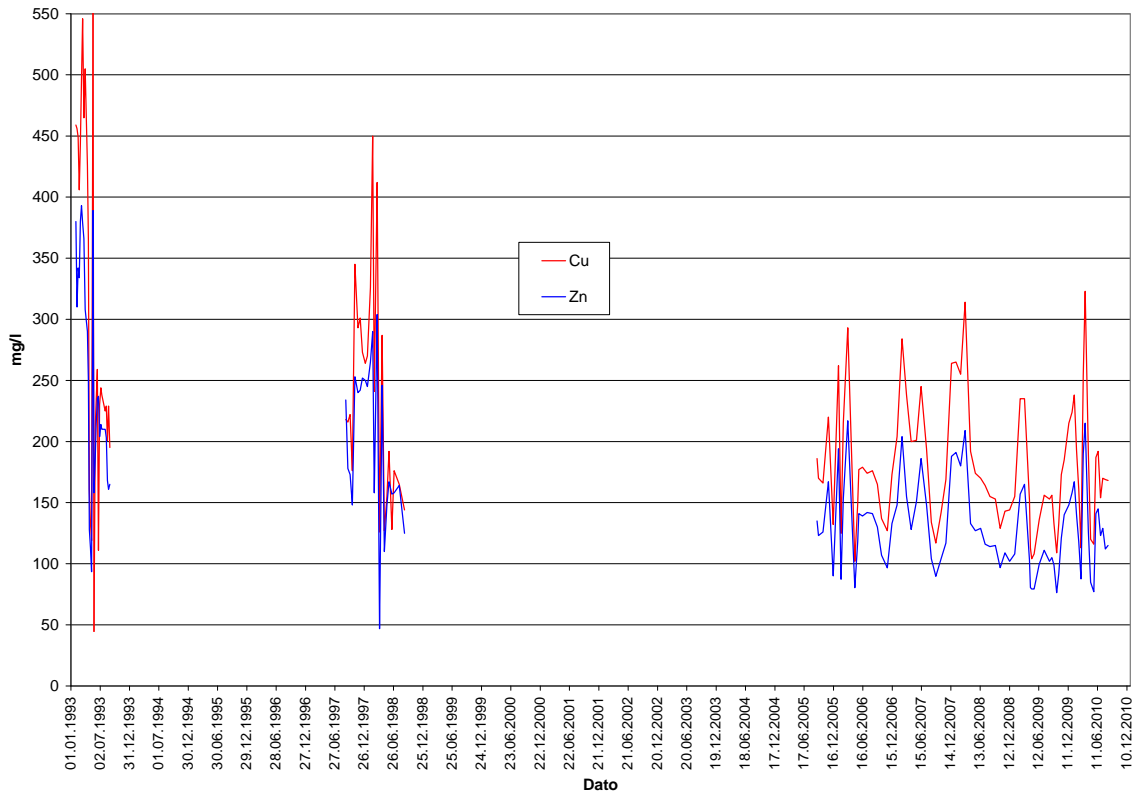
Figur 14. Kobber- og sinkobservasjoner ved Stasjon C, Drensgrøft i Gammelgruva, 1992-2010.
