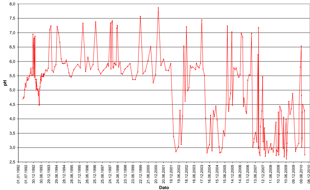
Figur 16. Laboratiemålinger av pH i prøver fra Wallenberg pumpestasjon 1992-2010.
