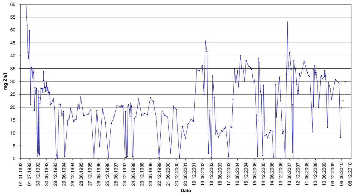
Figur 18. Sinkkonsentrasjoner ved Wallenberg pumpeasjon 1992-2010.
