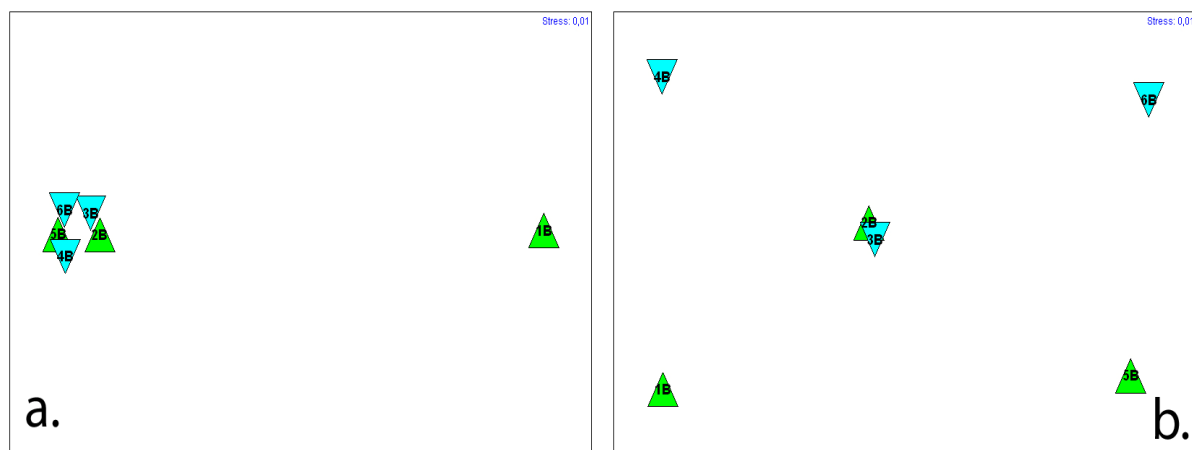
Figur 16. a. MDS-plott; likhet mellom de ikke-oljeeksponerte rammestasjonene mht. forekomst av alger. b. MDS-plott; likhet mellom de ikke-oljeeksponerte rammestasjonene mht. forekomst av dyr. Stasjoner nær hverandre er like. Stasjoner med høy bølgeeksponering er markert med grønne trekkanter, mens stasjoner med moderat bølgeeksponering er markert med blå trekkanter.
