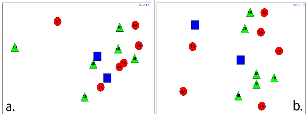
Figur 15. MDS-plott; likhet mellom alle rammestasjonene mht. forekomst av alger og dyr. Stasjoner nær hverandre er like. Stasjoner med registrert oljesøl er indikert med røde sirkler, stasjoner med lite/inget oljesøl med grønne trekantene og ikke-sanerte stasjoner med blå firkantene. a. Likhet mellom alle rutene mht. forekomst av alger. b. Likhet mellom alle rutene mht. forekomst av dyr
