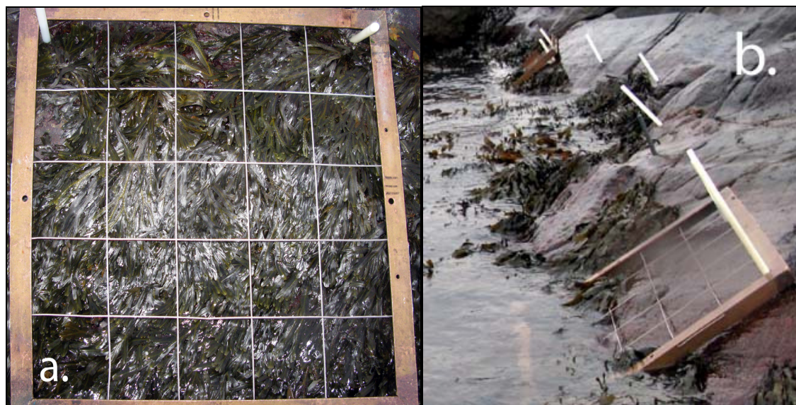
Figur 2. a. Ramme (0,5 x 0,5 m) inndelt i 25 hjelperuter (10 x 10 cm). b. 4 rammestasjoner merket med bolter i fjellet. Boltene blir fjernet mellom hver undersøkelse.
