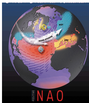
Positiv NAO-indeks
