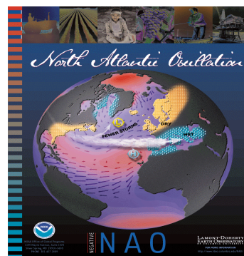
Negativ NAO-indeks
