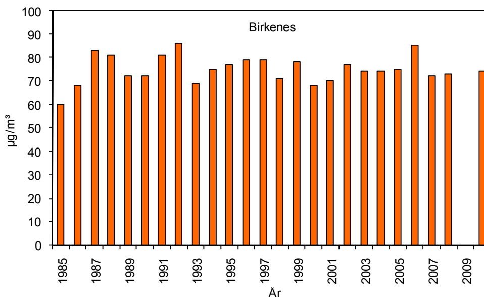
Figur 6. Middeldkonsentrasjon av ozon for 7 timer (kl. 09-16) i vekstsesongen (april-september) ved Birkenes i perioden 1985-2010.
