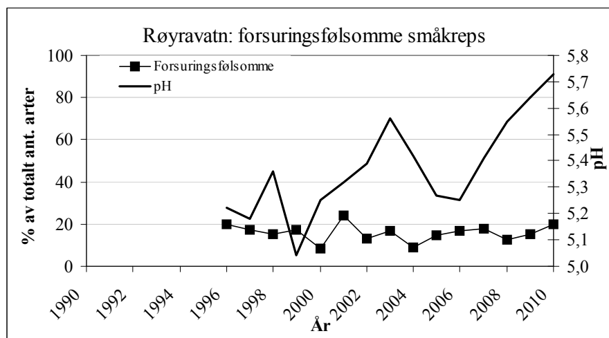
Figur 25. Andel (% arter) av forsuringfølsomme småkreat (Cladocera + Copepoda) i Røyrvatn (reg. VI, Vestlandet - Sør) i 1997-2010. pH er fra høstprøver.
