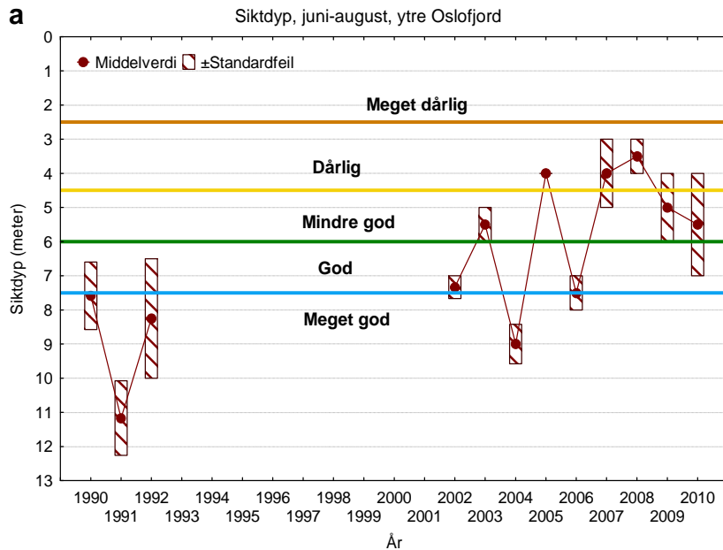
Figur 27. Siktdyp målt fra Torbjørnshjørn (OF-1) i sommerperioden juni-august. Data og figur fra kystovervåkingsprogrammet (Norderhaug et al. 2011).
