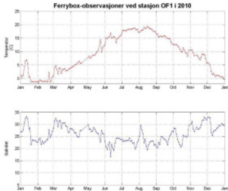
Figur 10. Temperatur og saltholdighet på ca. 4 m dyp for stasjon OF-1 Torbjørnshjær gjennom 2010. Data fra Ferrybox.
