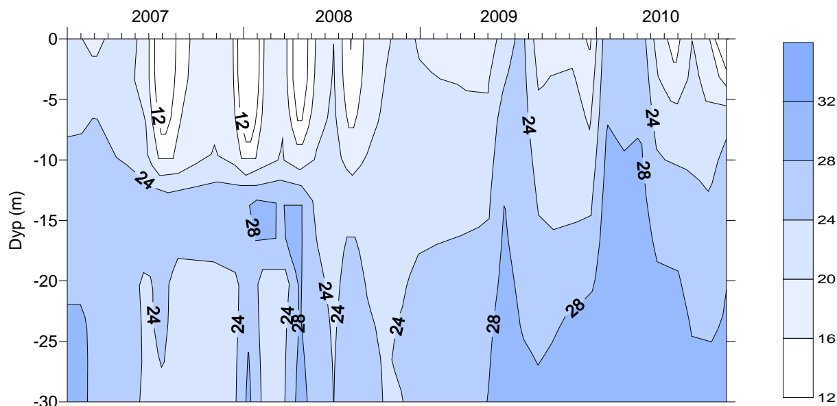
Figur 15. Saltholdighet i vannmassene på stasjon RA-5 Ringdalsfjorden i perioden 2007 til 2010.
