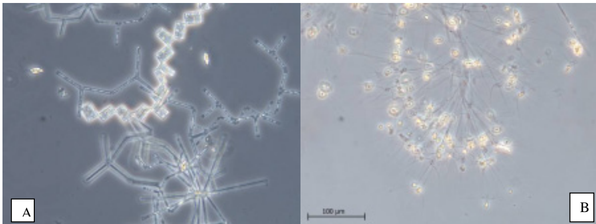
Figur 24. A. Brakkvanns kiselalger ( Diatoma tenuis , Tabellaria sp og Asterionellopsis glacialis ) i Drammensfjorden våren 2010. B. Chaetoceros socialis , en forholdsvis vanlig kiselalge våren 2010 ved OF-stasjonene. Foto: Havforskningsinstituttet, Algelaboratoriet
