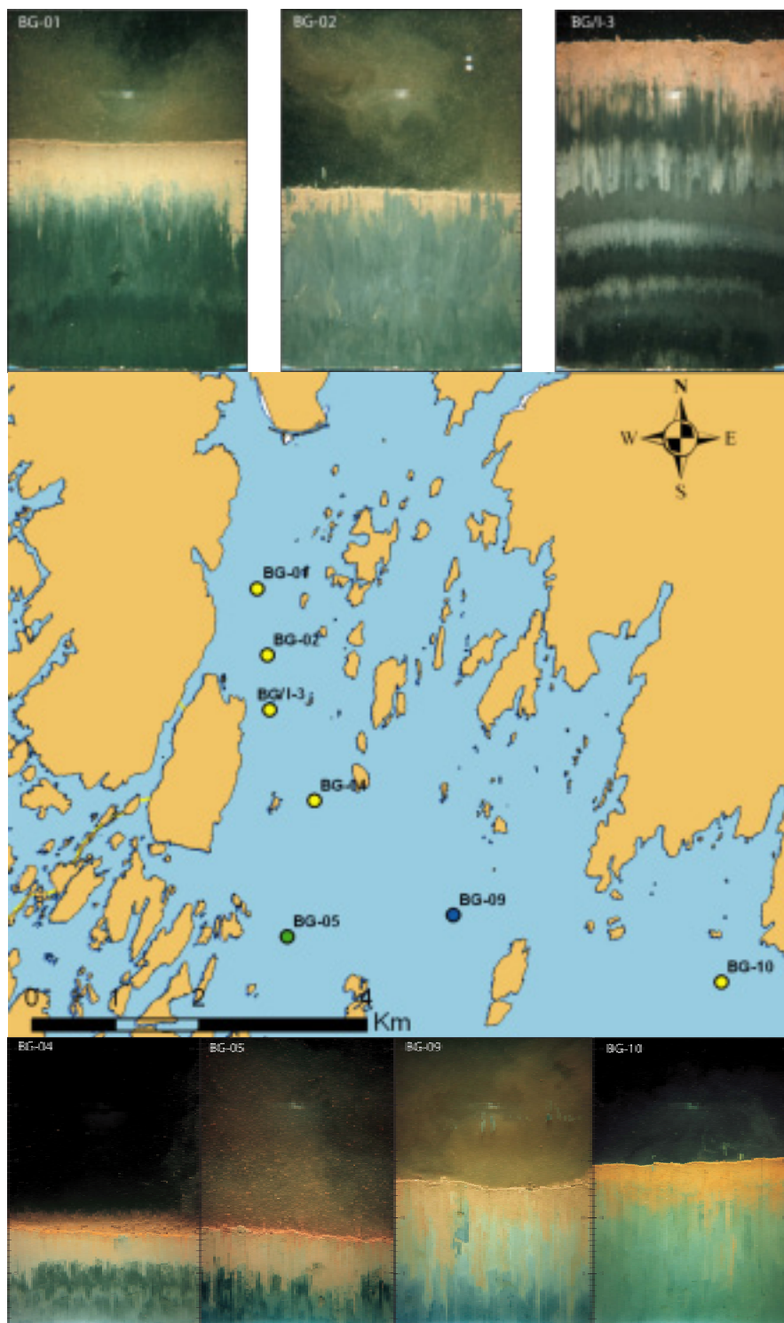
Figur 38. Tilstandsklasser på bløtbunn i henhold til BHQ-indeksen i 2010 og bilder fra stasjoner i intensivområdet i munningsområdet til Glomma.
