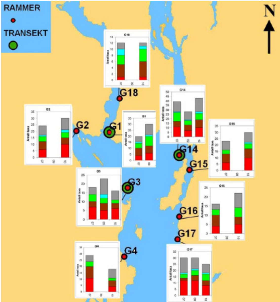
Figur 48. Antall taxa tilstede på ved rammeundersøkelser på strandsonestasjonene i nordlig del av Ytre Oslofjord i 2007, 2009 og 2010. Rødt illustrerer rødalger, brunt = brunalger, grønt = grønnalger, blått = kisel- og blågrønnalger, grått = dyr. Merk ulik skala på y-aksen.
