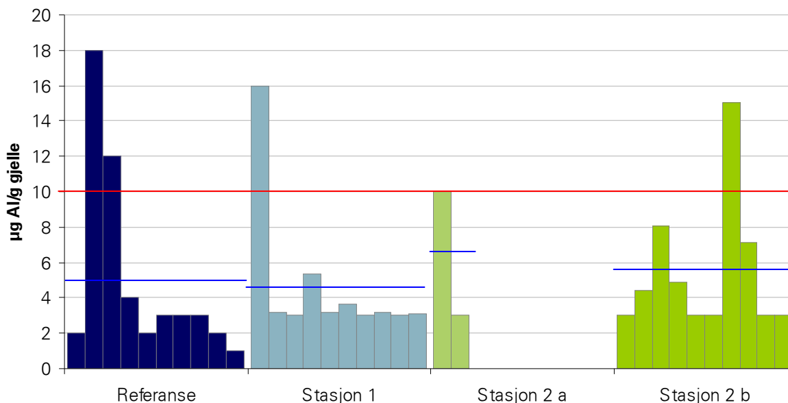
Figur 43. Aluminium (Al) akkumulert på gjeller av stedegen ørretsmolt i Begna. Fisken ble eksponert i 6 dager, fordelt på to grupper: Stasjon 1 (oppstrøms utslipp) og Stasjon 2 (nedstrøms utslipp). Stasjon 2a er fra perioden: 26. april – 2. mai 2011 og Stasjon 2b er fra perioden: 2. mai – 9. mai 2011. Det ble også tatt prøver av fisk før eksponering: Referanse. Hver søyle representerer en fisk. Blå horisontale linjer viser gjennomsnittet for gruppene. Rød horisontal linje viser normale bakgrunnsnivåer av Al i laks. Konsentrasjonene er oppgitt i µg Al/g tørrvekt gjelle.
