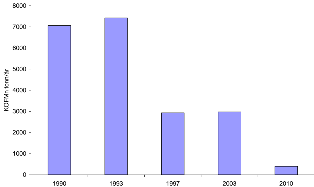
Figur 9. Årlig tilskudd til lett nedbrytbart organisk materiale målt som KOF-Mn til Begna forbi Follum før og etter installasjon av kjemisk rensanlegg, hhv 1990 og 1993, og biologisk rensanlegg, hhv 1993, 1997, 2003 og 2010/11.
