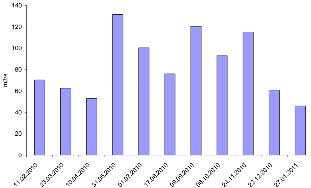
Figur 3. Gjennomsnittlig vannføring i Begna ved Strømstø i periodene mellom hver vannprøvetaking i 2010/11.
