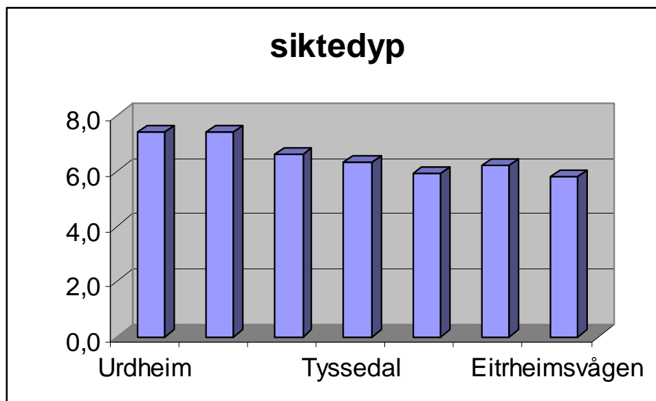
Figur 5. Gjennomsnittlig siktedyp (m) i Sør fjorden i 2010 (Urdheim er ytterst i Sør fjorden og Eitrheimsvågen innerst).
