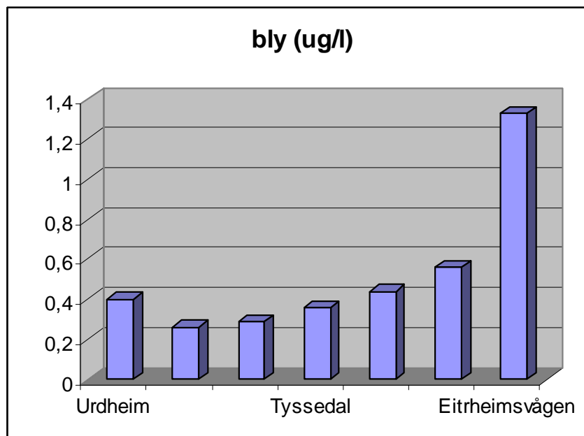
Figur 7. Konsentrasjonen av bly (µg/l) i overflatevann fra innerst (høyre) til ytterst (venstre) i Sør fjorden i 2010 (årgjennomsnitt).
