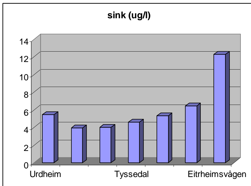
Figur 6. Årsgjennomsnittet av sink (µg/l) i overflatevann fra innerst (høyre) til ytterst (venstre) i Sørfjorden 2010.
