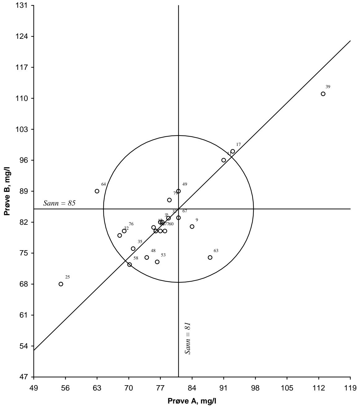
Figur 5. Youtendiagram for suspendert stoff, gløderest, prøvepar AB Akseptansegrensen, angitt med en sirkel, er 20 %
