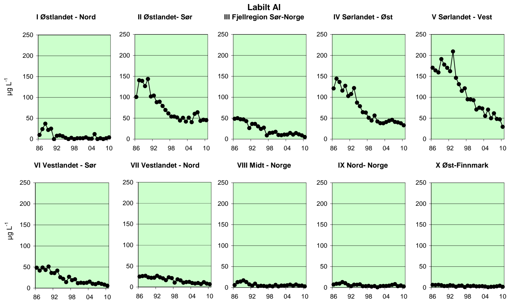
Figur 22. Trender i LAI (labilt uorganisk aluminium) for perioden 1986-2010 for innsjøer i de 10 regionene.
