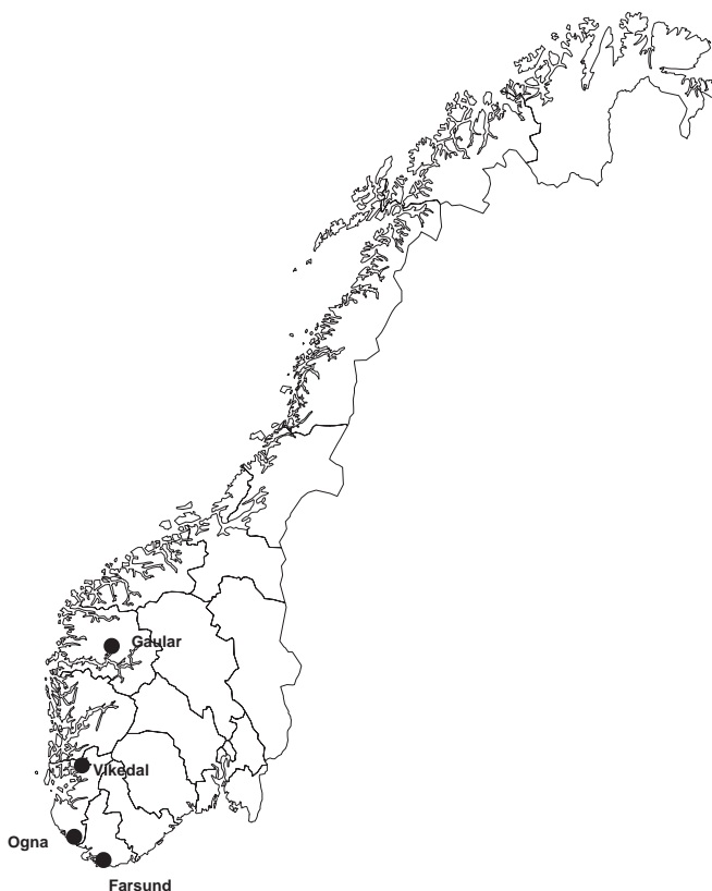
Figur 66. Lokalisering av overvåkingstasjonene for invertebratundersøkelser i vassdrag i 2010.
