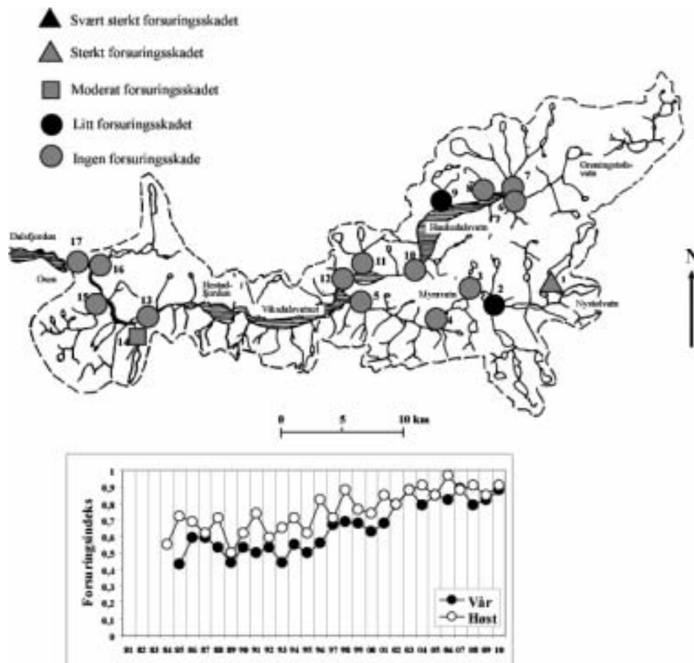
Figur 70. Oversikt over innsamlingslokaliteter og sammensetning av bunndyr i Gaularvassdraget i 2010. Figuren viser også gjennomsnittlige forurensningsverdier vår (V) og høst (H) i perioden 1984-2010.
