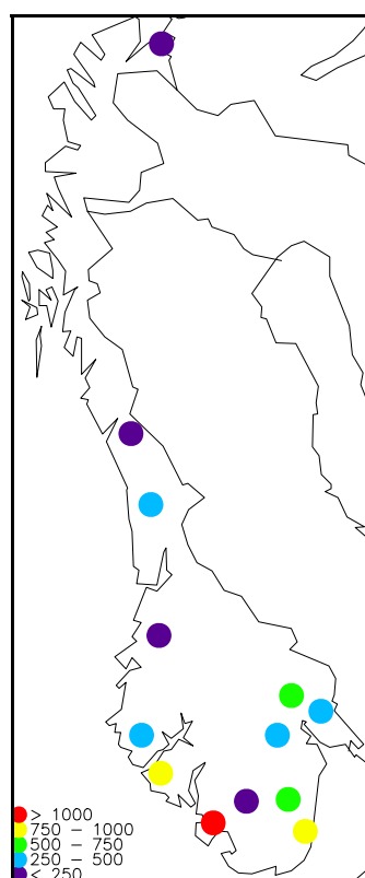
Figur 2. Middelskonsentrasjoner i nedbør av sulfat og pH, våtavsetning av sulfat og nitrat + ammonium på norske bakgrunnsstasjoner i 2010.
