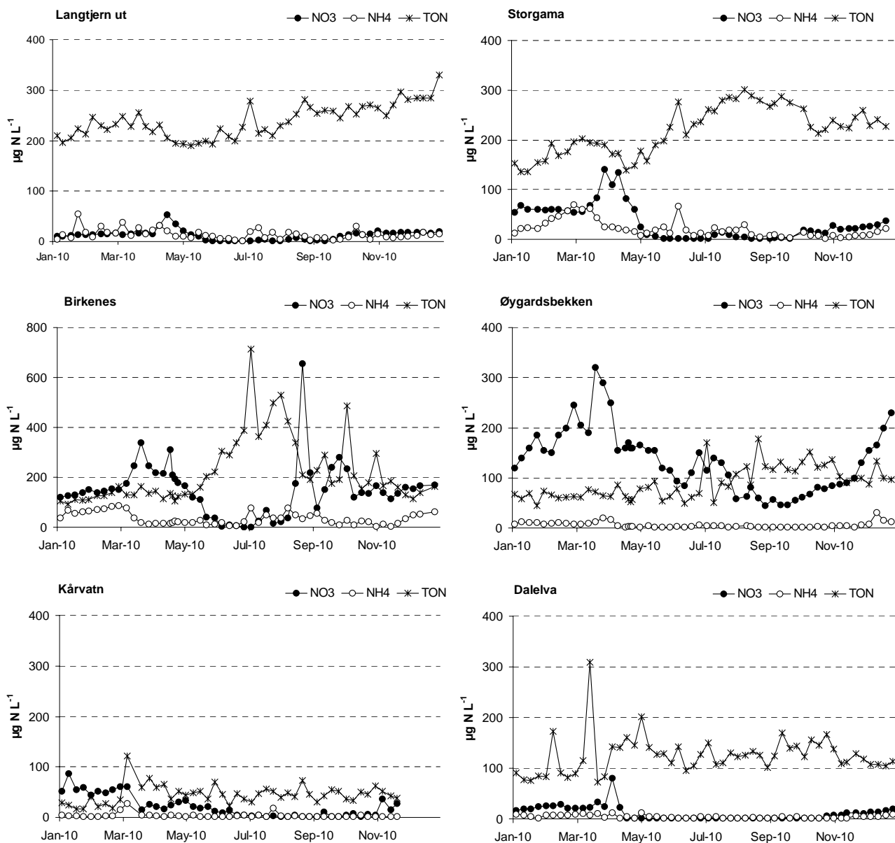
Figur 41. Sesongmessig fordeling av nitrat ( \text{NO}_3 ), ammonium ( \text{NH}_4 ) og totalt organisk nitrogen (TON) i feltforskningsområdene i 2010. TON = total nitrogen – \text{NO}_3 – \text{NH}_4 . Enhet: \mu\text{g N L}^{-1} .
