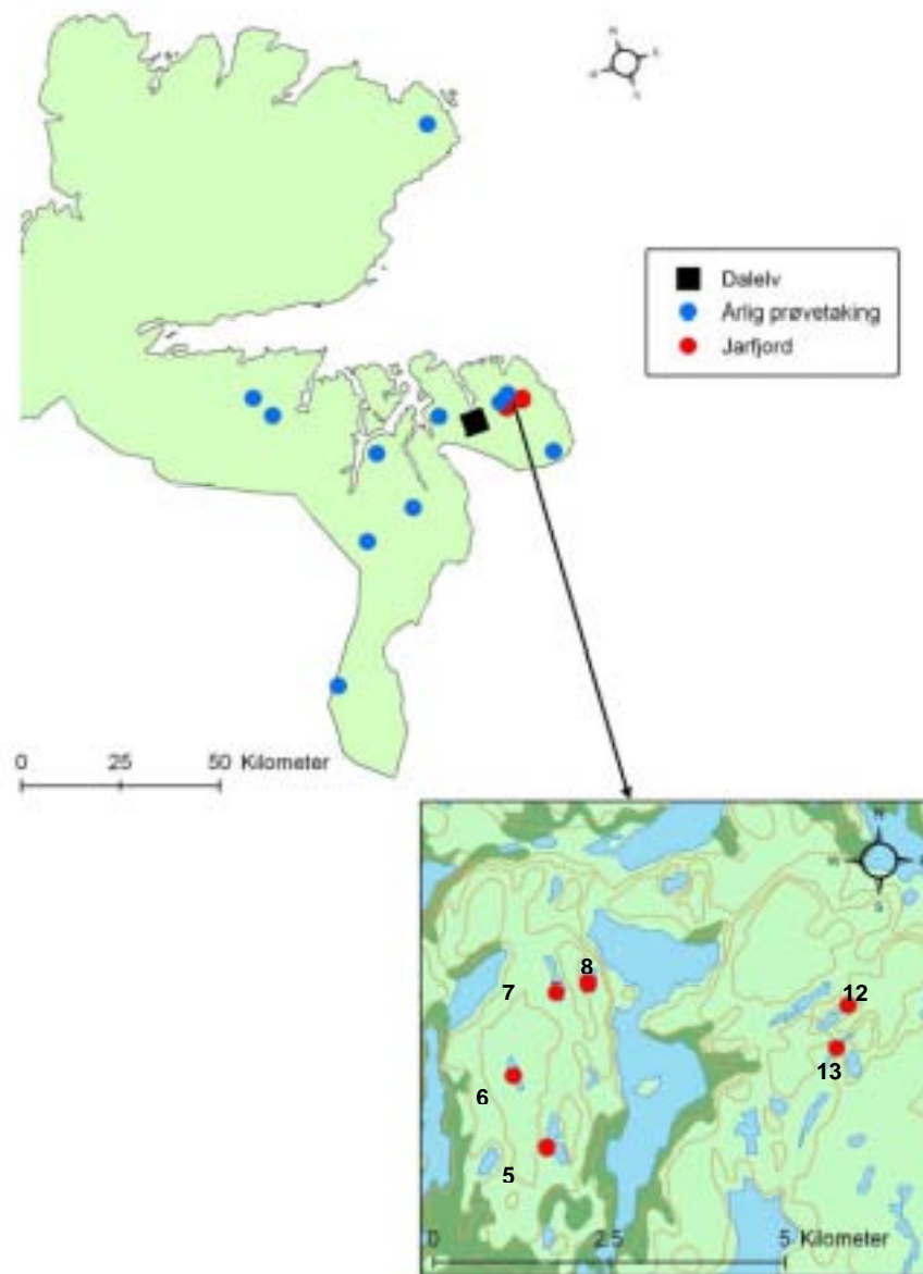
Figur 24. Lokalisering av overvåkingslokaliteter i Øst-Finnmark, i Sør-Varanger kommune. Både Jarlfjordfjell-sjøene, tidstrendsjøene (årlig prøvetaking) og feltforskningsstasjonen Dalelv er vist på kartet. Tallene er en forkortelse av identifikasjonen på lokalitetene (5 er JAR-05, 6 er JAR-06 osv.).
