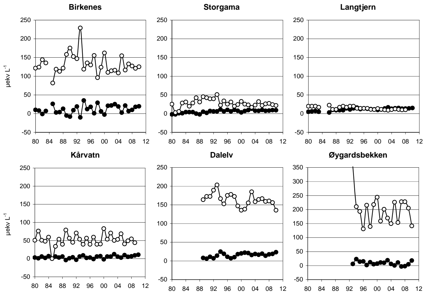
Figur 39. Klorid og ikke-marin natrium i feltforskningsstasjonene. Ikke-marin natrium ● og klorid ○. Enhet: \mu\text{ekv L}^{-1} . OBS! Skala Øygardsbekken.
