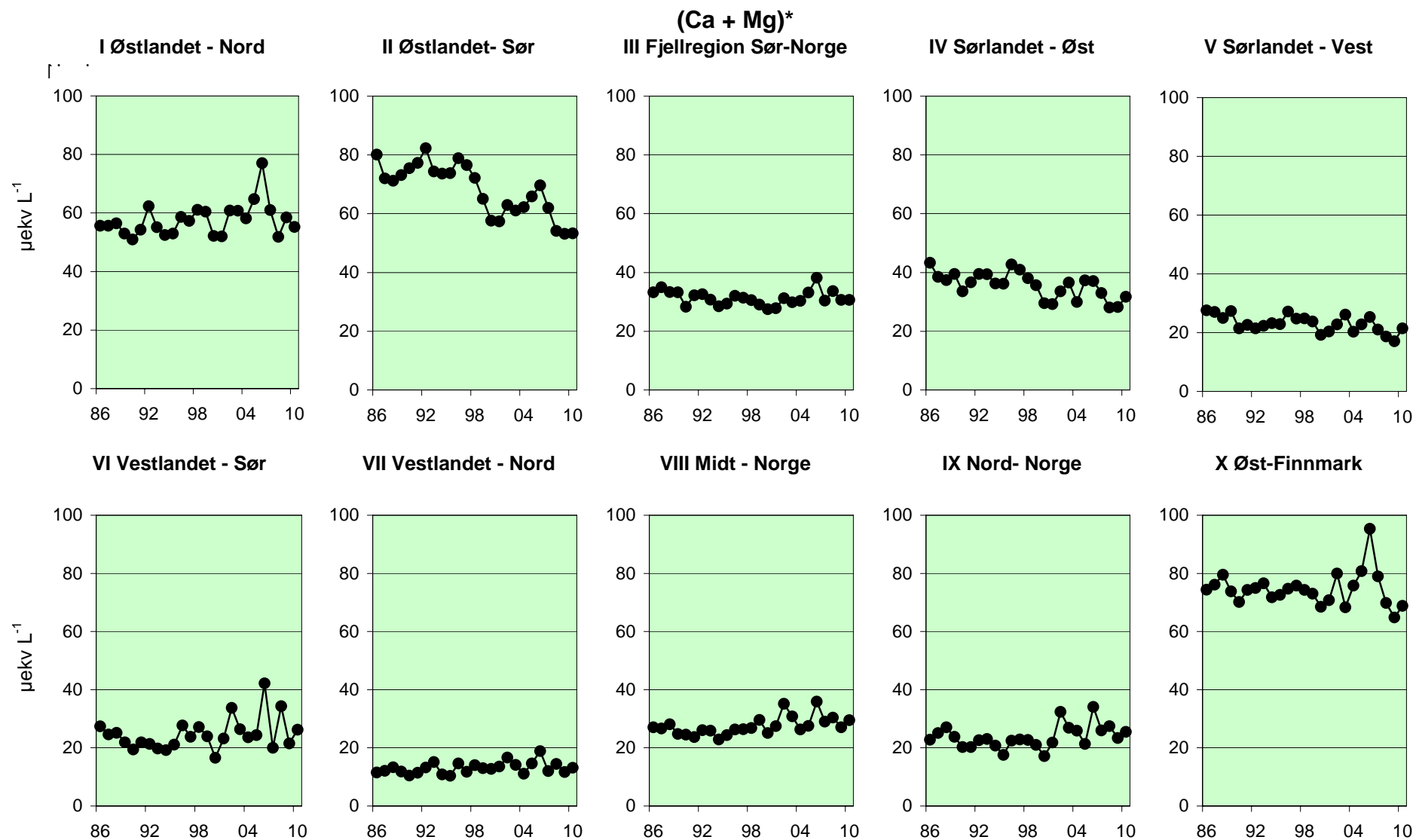
Figur 15. Trender for perioden 1986-2010 for basekationer for innsjøer i de 10 regionene.
