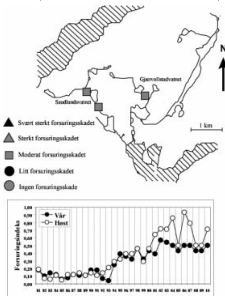
Figur 67. Oversikt over innsamlingslokaliteter og sammensetning av bunndyr i Farsundområdet i 2010. Figuren viser også gjennomsnittlige forursingsverdier vår (V) og høst (H) i perioden 1981-2010.
