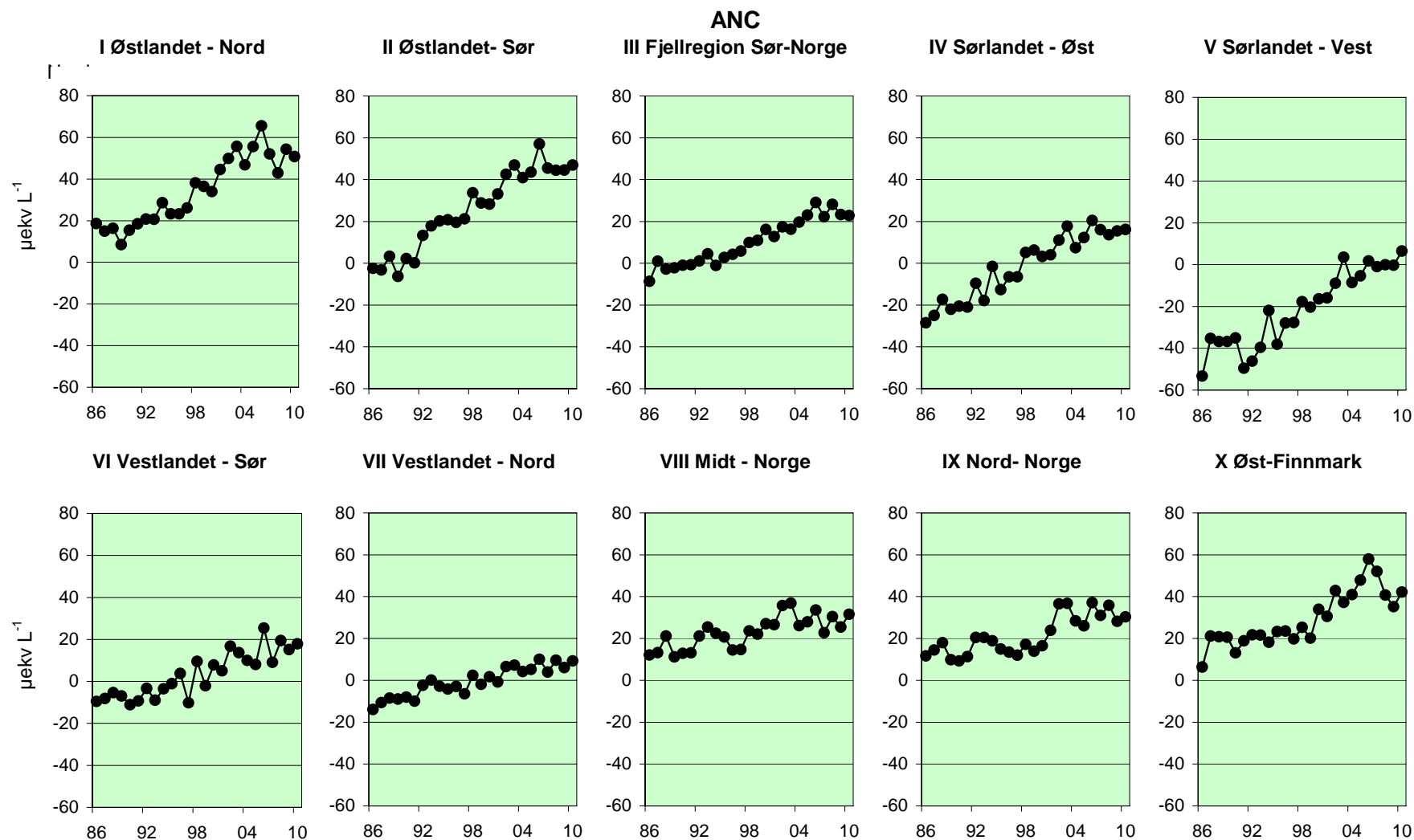
Figur 20. Trender for perioden 1986-2010 for ANC (syrenøytraliserende kapasitet) for innsjøer i de 10 regionene.
