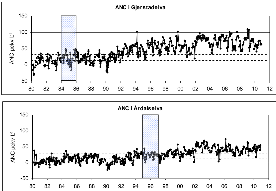
Figur 30. ANC i Gjerstadelva og Årdalselva for perioden 1980 - 2010. Enhet µekv L -1 . Området som er skyggelagt, angir tidsrom for antatt oppstart av kalkingsaktiviteter i nedbørfeltet til elvene. De stiplede linjene antyder antatte grenseverdier for laks (30 µekv L -1 ) og innlandsørret (15 µekv L -1 ) (Henriksen m.fl. 1995, Kroglund m.fl. 2002).
