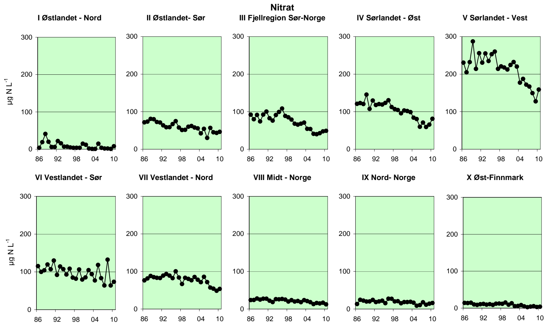
Figur 19. Trender for perioden 1986-2010 for nitrat for innsjøer i de 10 regionene.
