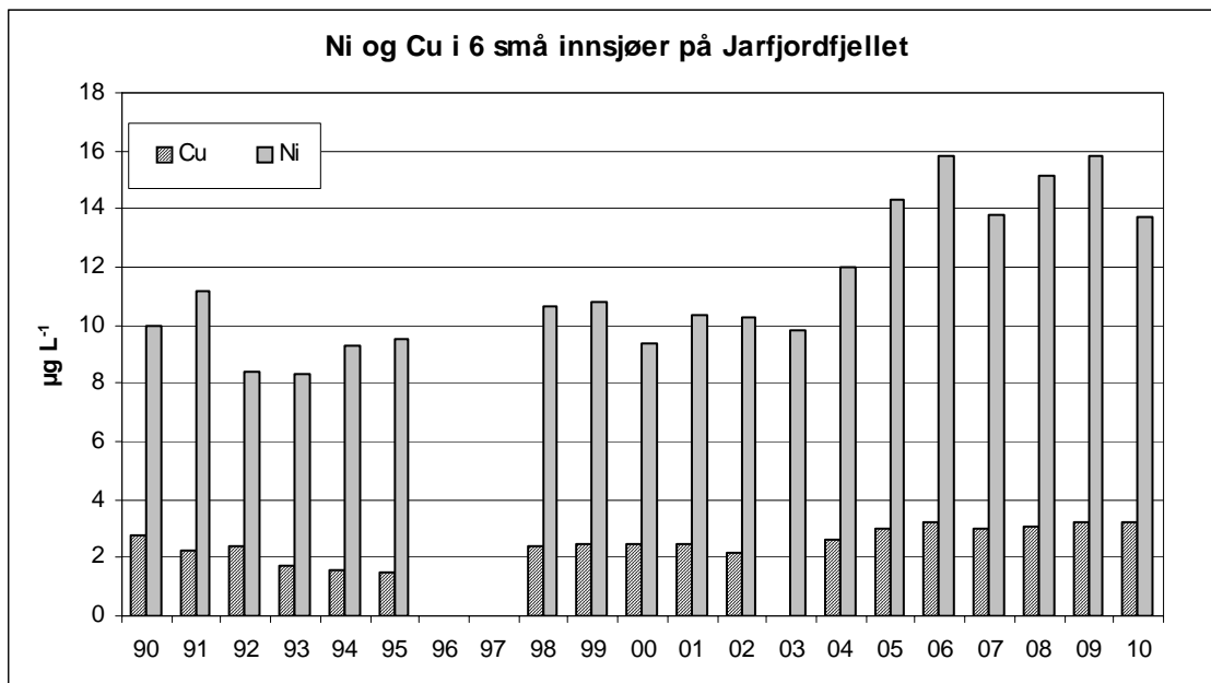
Figur 26. Årlige middelværdier for nikkell og kobber i seks små innsjøer på Jarfjordfjellet fra 1990 til 2010.
