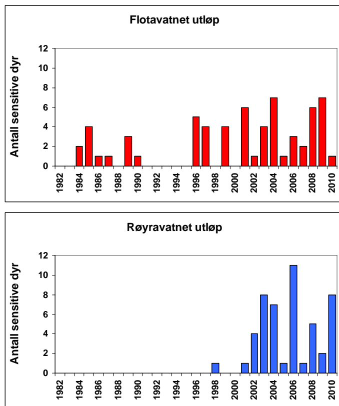
Figur 61. Forekomst av forsuringssensitive bunndyr i utløpselvene fra Flotavatnet og Røyrvatnet (Vikedal) i perioden 1982-2010.
