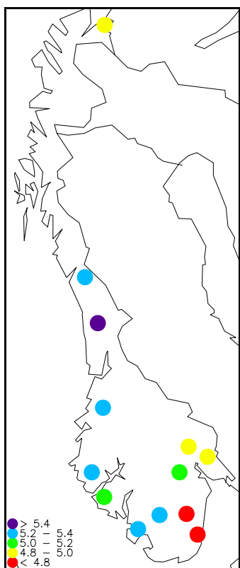
Figur 2. Middelskonsentrasjoner i nedbør av sulfat og pH, våtavsetning av sulfat og nitrat + ammonium på norske bakgrunnsstasjoner i 2010.
