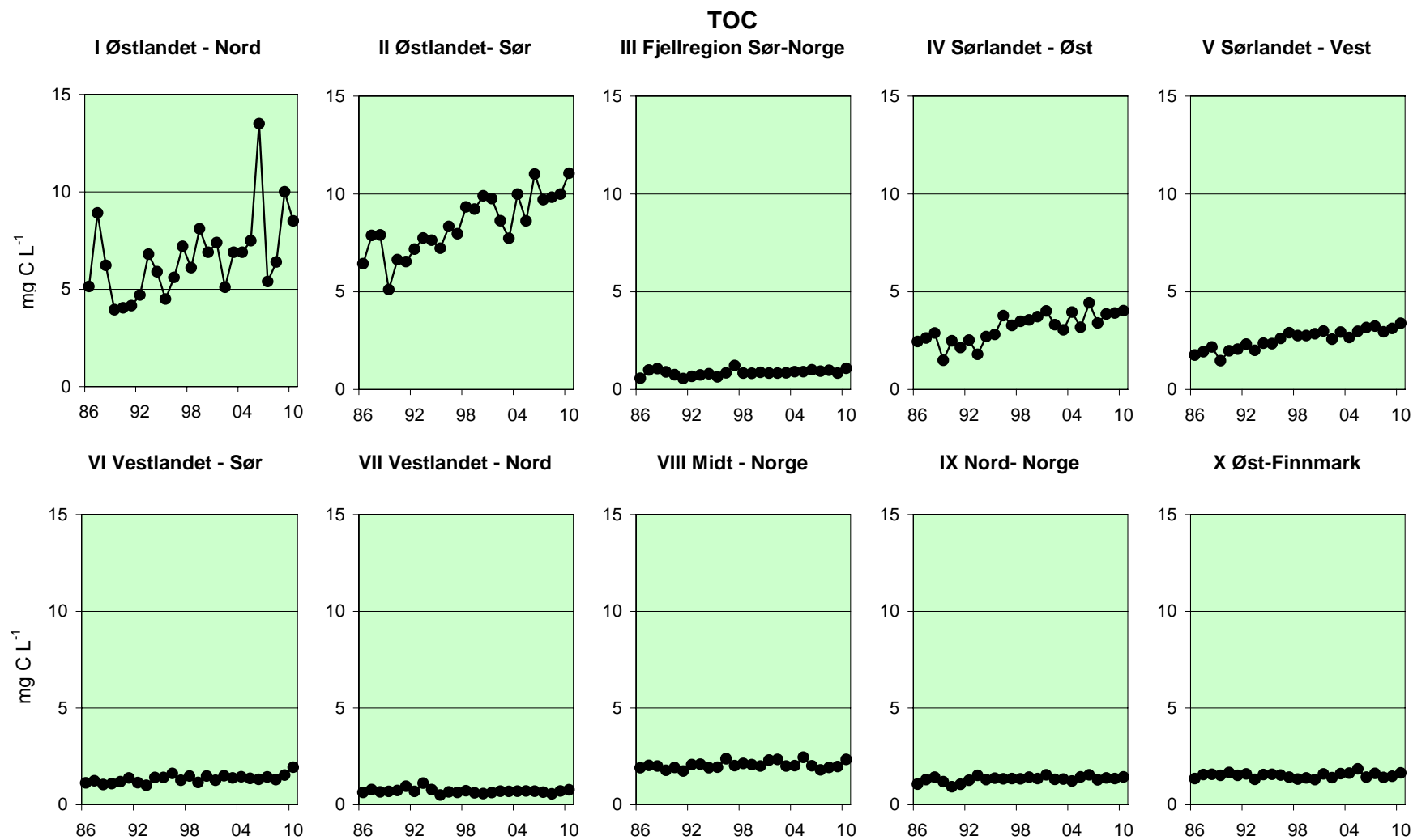
Figur 23. Trender i TOC (total organisk karbon) for perioden 1986-2010 for innsjøer i de 10 regionene.
