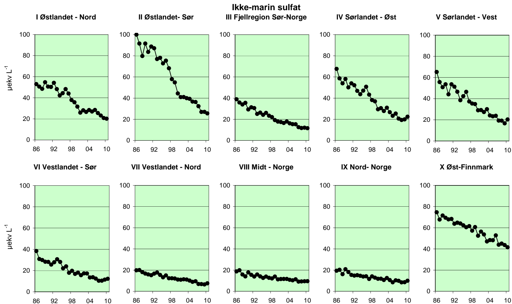
Figur 18. Trender for perioden 1986-2010 for ikke-marin sulfat for innsjøer i de 10 regionene.
