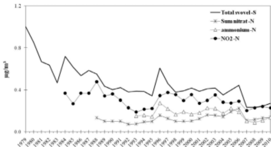
Figur 4. Midlere årlige konsentrasjoner i luft av total svovel ( \text{SO}_2 + \text{SO}_4^- ), oksidert nitrogen ( \text{HNO}_3 + \text{NO}_3 ), redusert nitrogen ( \text{NH}_4 ) og \text{NO}_2 på tre norske EMEP-stasjoner (Birkenes, Kårvatn og Tustervatn).
