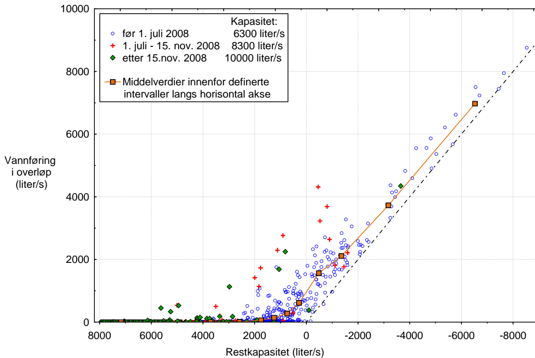
Figur 28. Vannføring i overløp som funksjon av nominell restkapasitet. Horizontalaksen er snudd slik at totalvannføringen øker mot høyre innenfor hver periode. Stiplet linje markerer hvor mye som må gå i overløp dersom kapasiteten blir fullt utnyttet ved ulike totalvannføringer.
