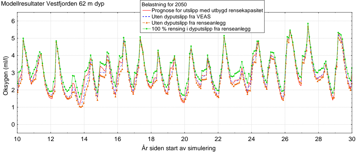
Figur 38. Oksygeninnhold på 62 m dyp - modellresultater fra teoretiske scenarier med reduksjon/fjerning av tilførsler fra renseanlegg og/eller overløp fra Indre Oslofjord.
