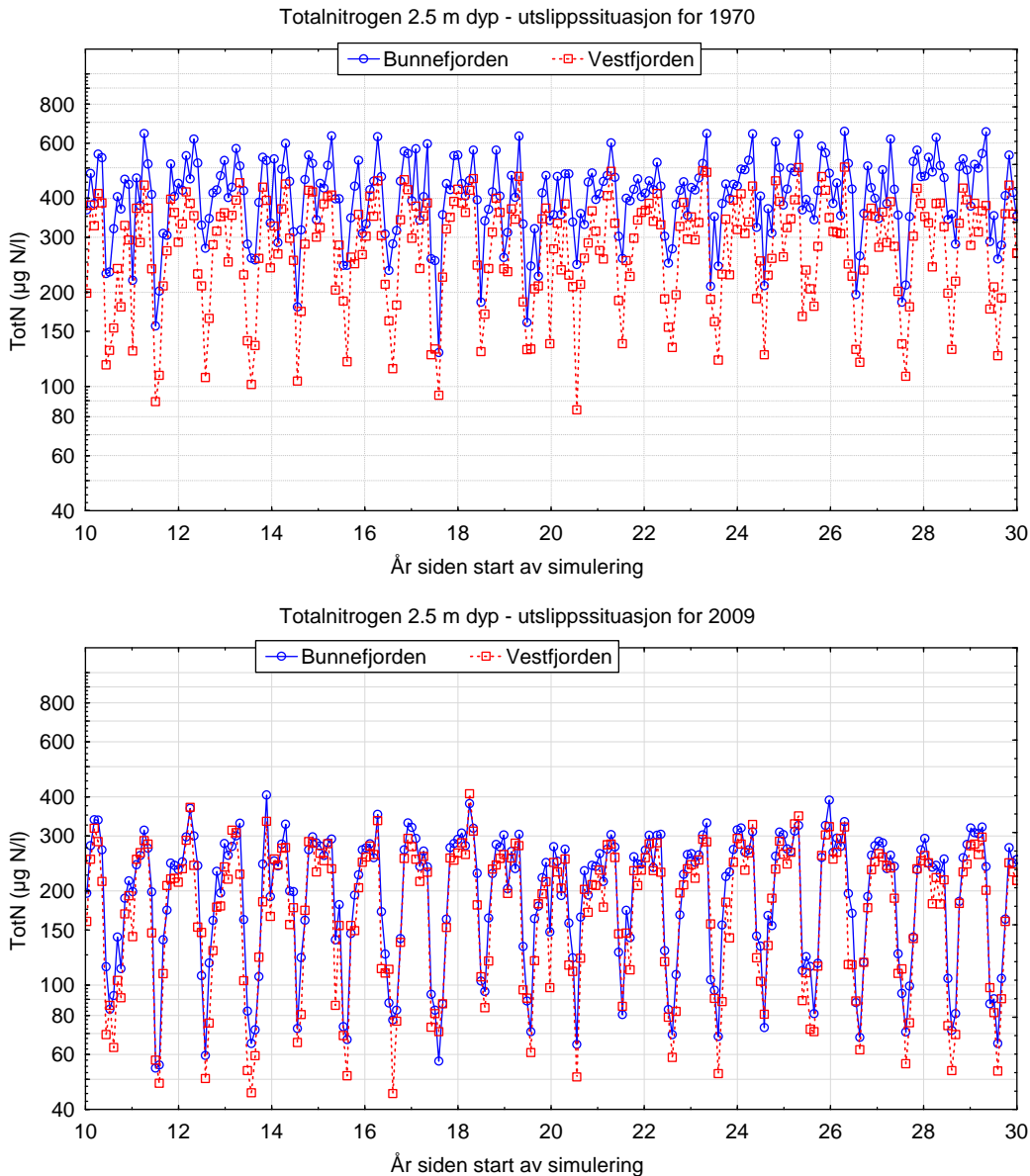
Figur 5. Modellresultater, totalnitrogen i 2.5 m dyp i Bunnefjorden og Vestfjorden for utslippsituasjon pr. 1970 og 2009
