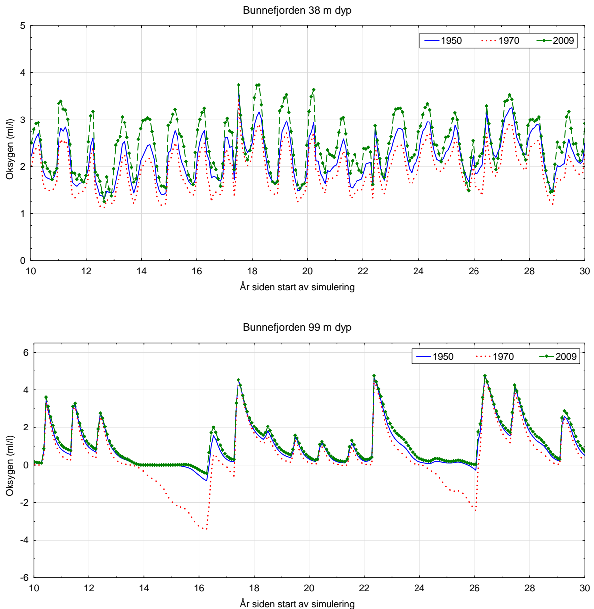
Figur 17. Modellresultater for oksygenkonsentrasjon i Bunnefjorden for parallelle kjøring med utslippsituasjon for 1950, 1970 og 2009. Bemerk ulik vertikal akse i øvre og nedre del av figuren.
