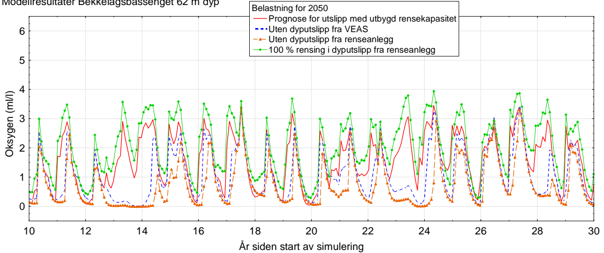
Modellresultater Bunnefjorden 62 m dyp
