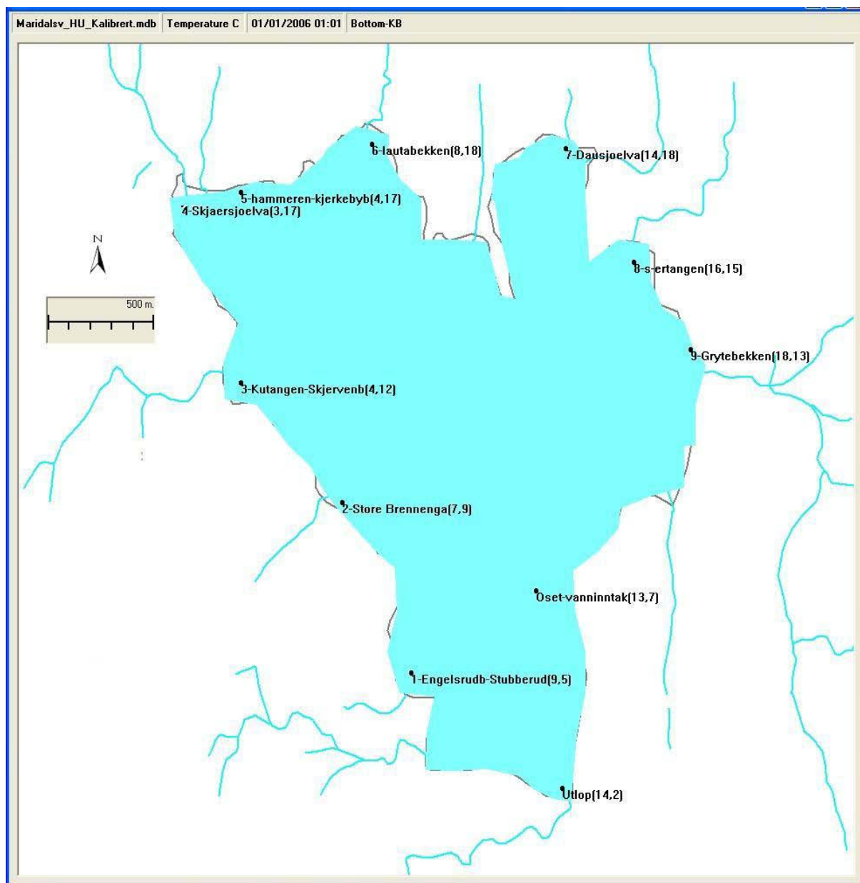
Figur 3-17. Tilførslene ble fordelt på 9 bekker/elver
