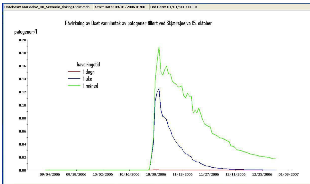
Figur 3-29. Utslipp den 15. oktober av 10^{10} patogener ved Skjærstjøelva. Figuren viser påvirkning av Oset vanninntak av patogener med ulik overlevelsessevne/halveringstid. Påvirkningen av patogenene økte med økt overlevelsessevne, men forskjellene var betydelig mindre enn ved utslippet 31. august.
