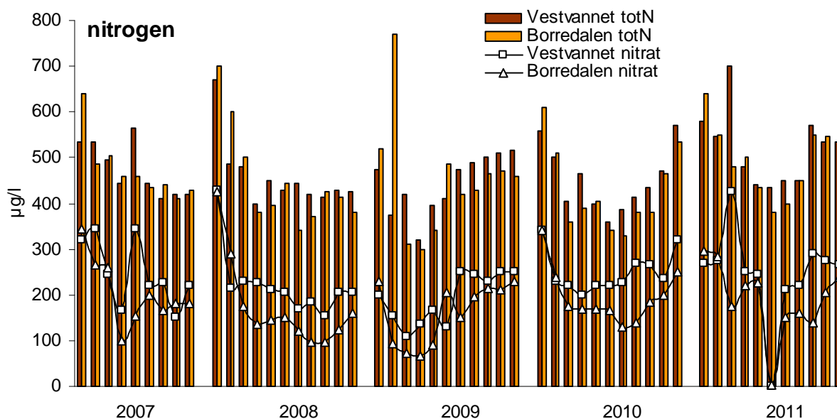
Figur 8. Nitrogen i overflatevannet (0-4 m) for perioden 2007-2011. Søyler angir totalt nitrogen, og linjer angir løst nitrat.
