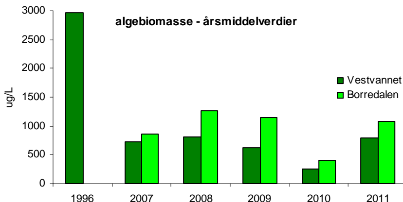
Figur 12. Algebiomasse ( \mu\text{g/L} ) i Vestvannet (mørk grønn) og Borredalen (lys grønn) – årsmiddelerdien for de fem siste årene, samt for 1996 (kun Vestvannet).
