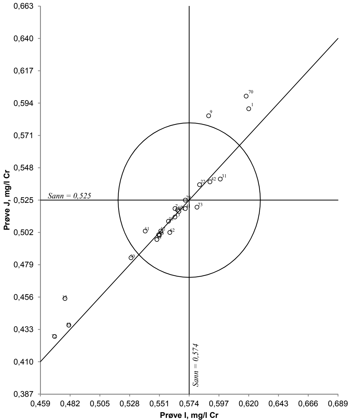
Figur 29. Youdendiagram for krom, prøvepar IJ Akseptansgrensen, angitt med en sirkel, er 10 %
