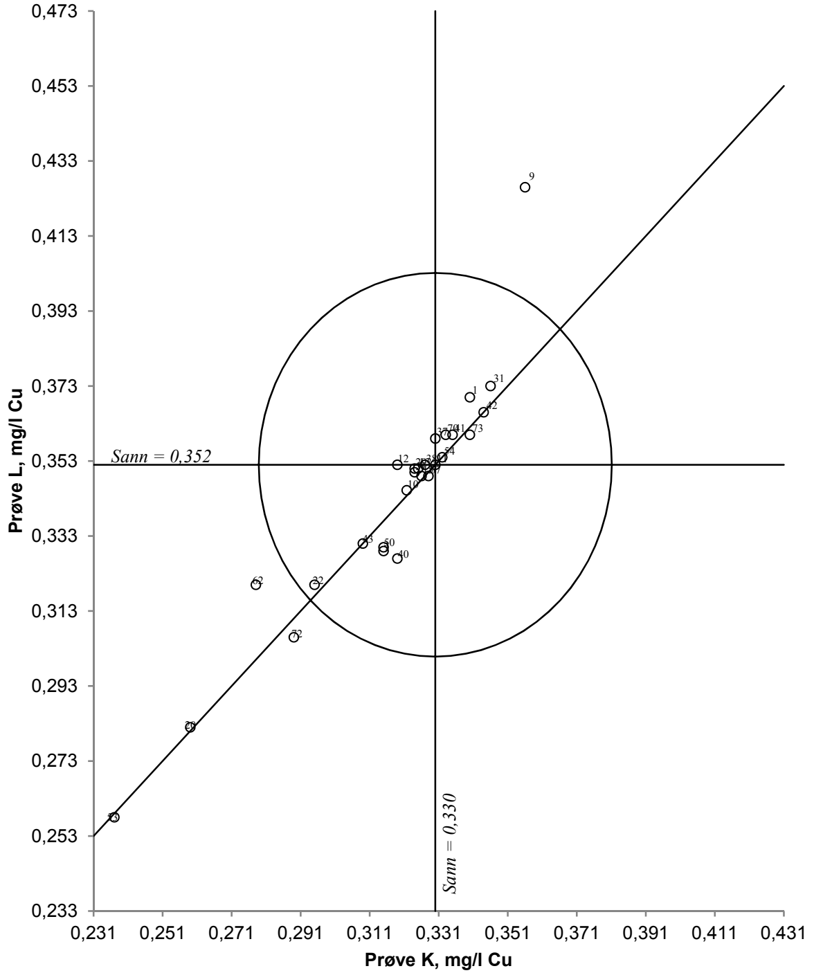
Figur 28. Youdendiagram for kobber, prøvepar KL Akseptansegrensen, angitt med en sirkel, er 15 %
