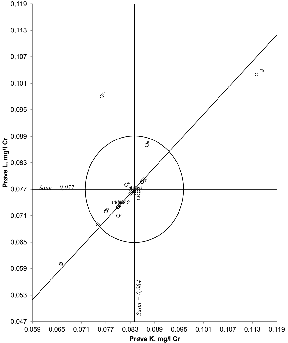
Figur 30. Youndendiagram for krom, prøvepar KL Akseptansegrensen, angitt med en sirkel, er 15 %
