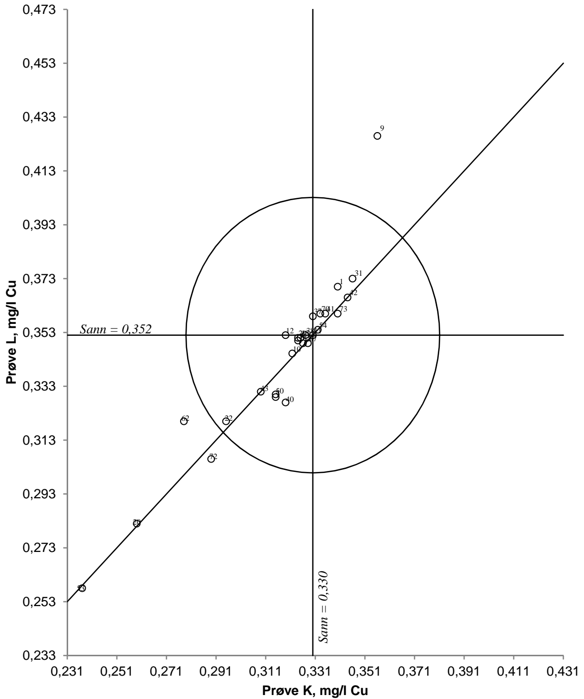
Figur 28. Youndendiagram for kobber, prøvepar KL Akseptansegrensen, angitt med en sirkel, er 15 %
