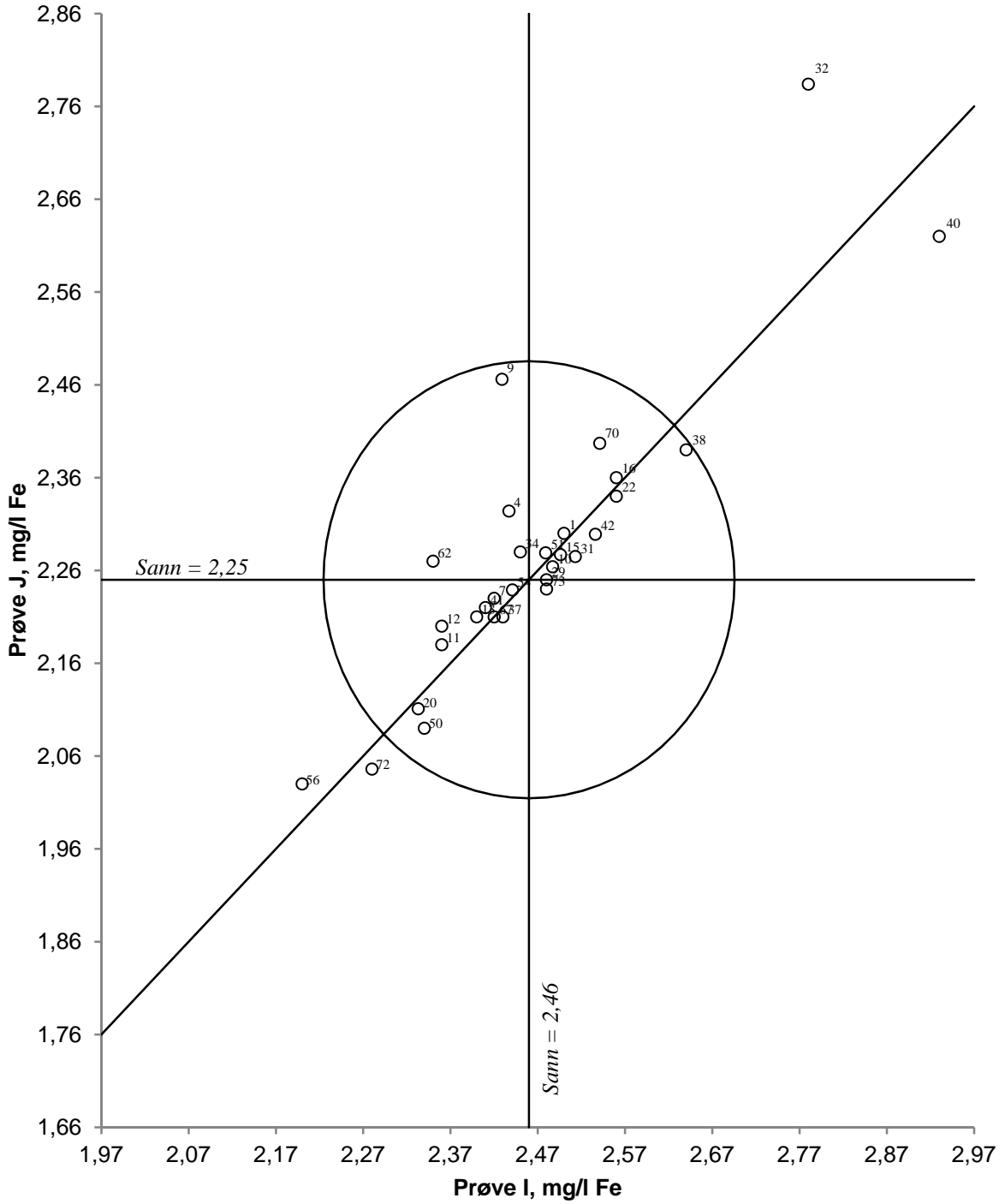
Figur 23. Youndendiagram for jern, prøvepar IJ Akseptansegrensen, angitt med en sirkel, er 10 %
