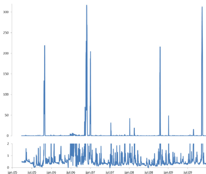
Figur 4. Vannføring ( \text{m}^3/\text{s} ) i Sireåna 2005-2009. Data er hentet fra NVE vannføringsstasjon 26.18 Langhølen. Brudd på y-aksen ved 2\text{m}^3/\text{s} indikerer ulik vannføringskalka over og under.
