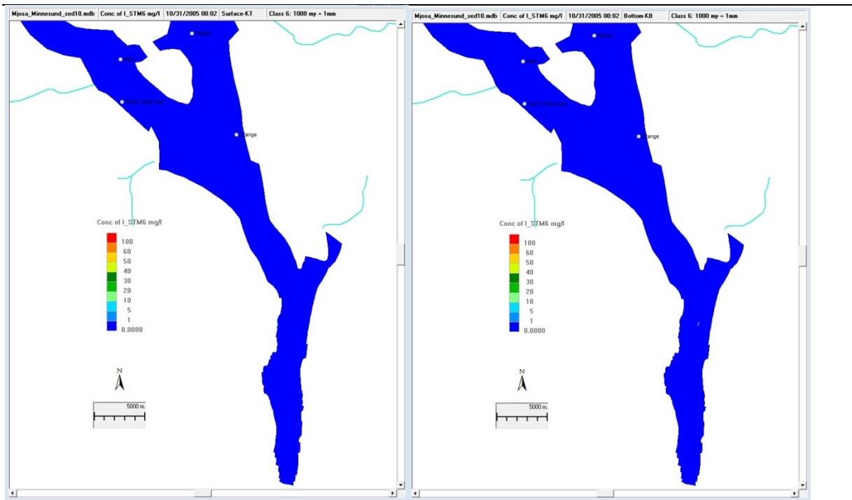
Figur 48. Kornstørrelses klasse 6, diameter = 1000 µm = 1 mm. Overflatestrøm nordover 31. oktober. Partiklene forventes å sedimentere raskt.
