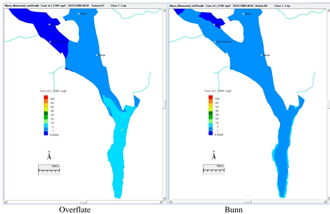
Figur 43. Kornstørrelses klasse 1, diameter = 2 \mu\text{m} . Overflatestrøm nordover 31. oktober. Konsentrasjoner over 5mg/l forventes i overflaten sør for Tangen. For øvrig forventes verdier over 1 mg/l jevnt fordelt i hele innsjøen sør for Hamar.
