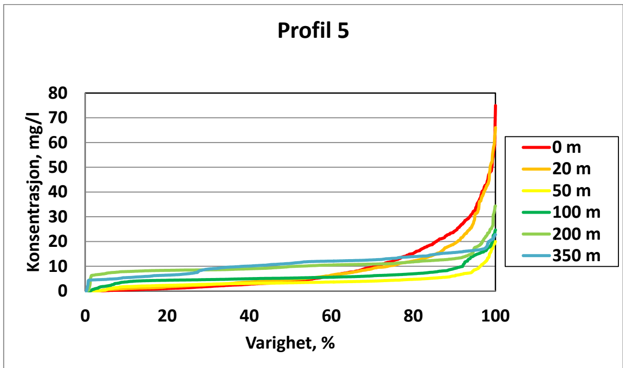
Figur 34. I halvparten av tiden ble konsentrasjonene i overflaten og på bunnen mindre enn henholdsvis 5 mg/l og 12 mg/l. Tilsvarende maksimumkonsentrasjoner ble 75 mg/l og 25 mg/l. Konsentrasjonene i overflaten varierte mye, men langt mindre på dypt vann.
