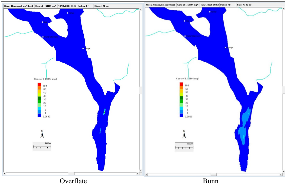
Figur 46. Kornstørrelses klasse 4, diameter = 40 µm. Overflatestrøm nordover 31. oktober. Partiklene sedimenterte raskt. De høyeste konsentrasjonene, over 5 mg/l, forventes kun ved dumpingstedene.
