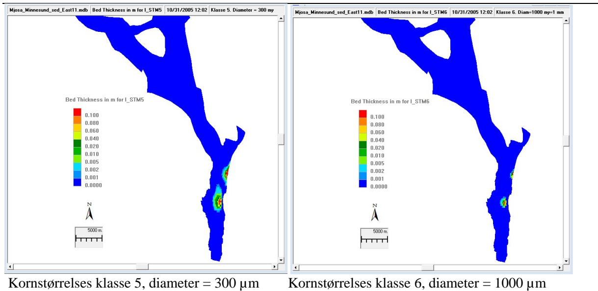
Figur 10. De største partiklene sedimenterte innen noen kilometre fra dumpingstedene, og tykkelsen kan bli over 10 cm.
