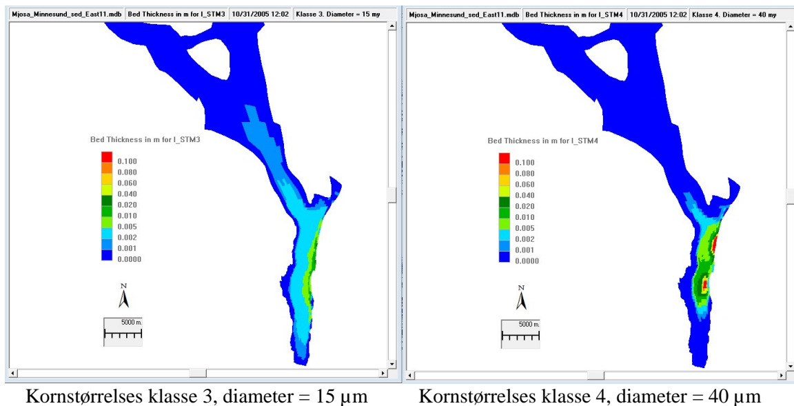
Figur 9. Klasse 3, med diameter på 15 µm, sedimenterte i et tynt lag på noen millimeter i de dypeste partiene sør for Stange vannverksinntak økende til et par cm nær dumpingstedene. Klasse 4, med diameter på 40 µm, sedimenterte noe nærmere dumpingstedene enn de finere partiklene og med en tykkelse på over 10 centimeter.
