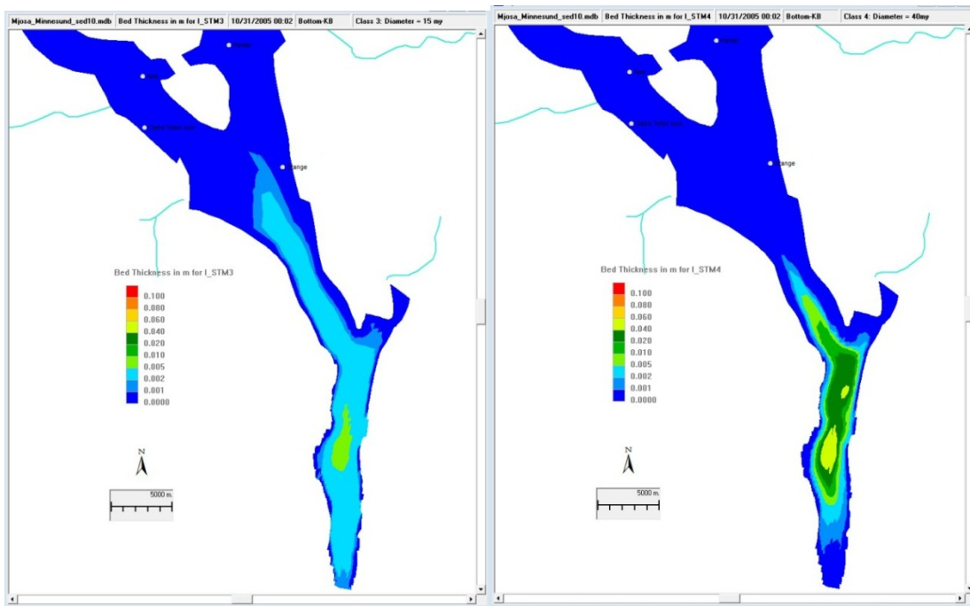
Kornstørrelses klasse 3, diameter = 15 \mu\text{m}
