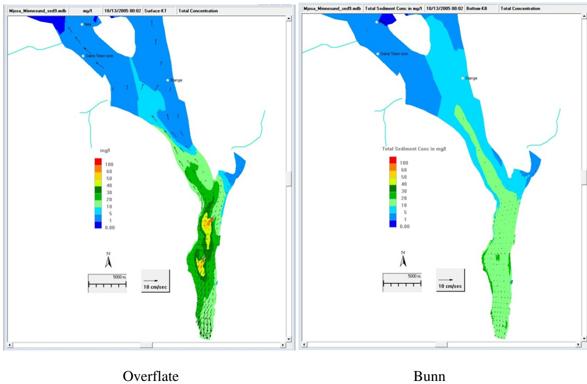
Figur 51. Total konsentrasjon av partikler.
