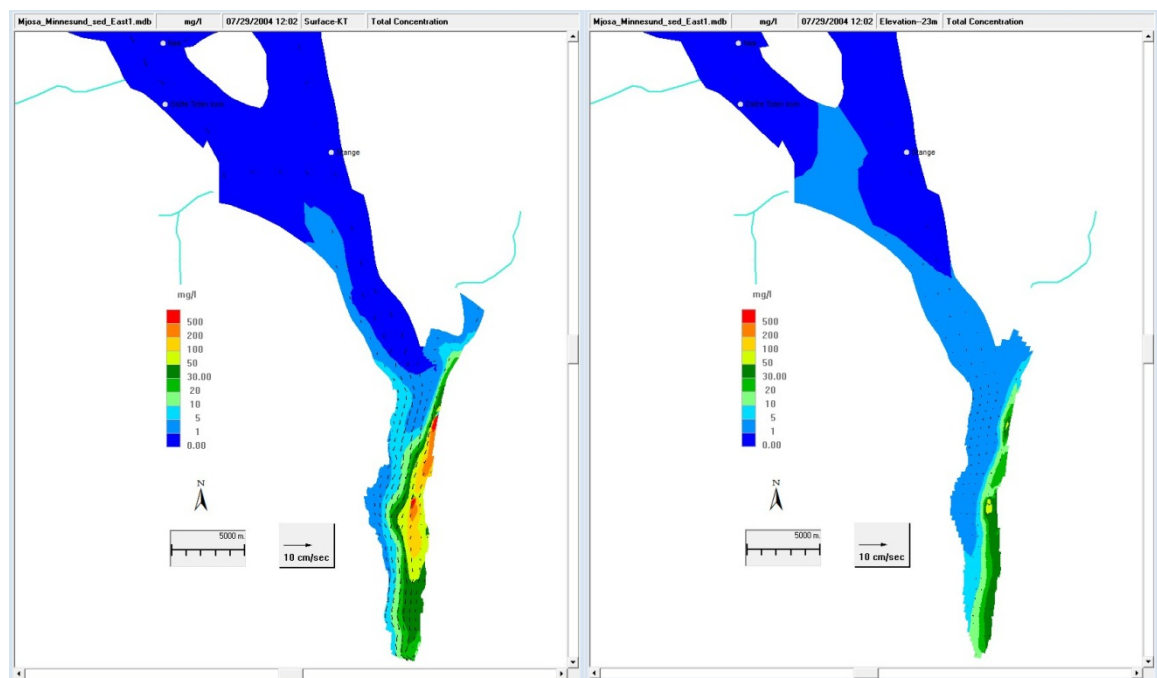
Figur 21. Total konsentrasjon av partikler gitt en overflatestrøm sørover den 29. juli.
