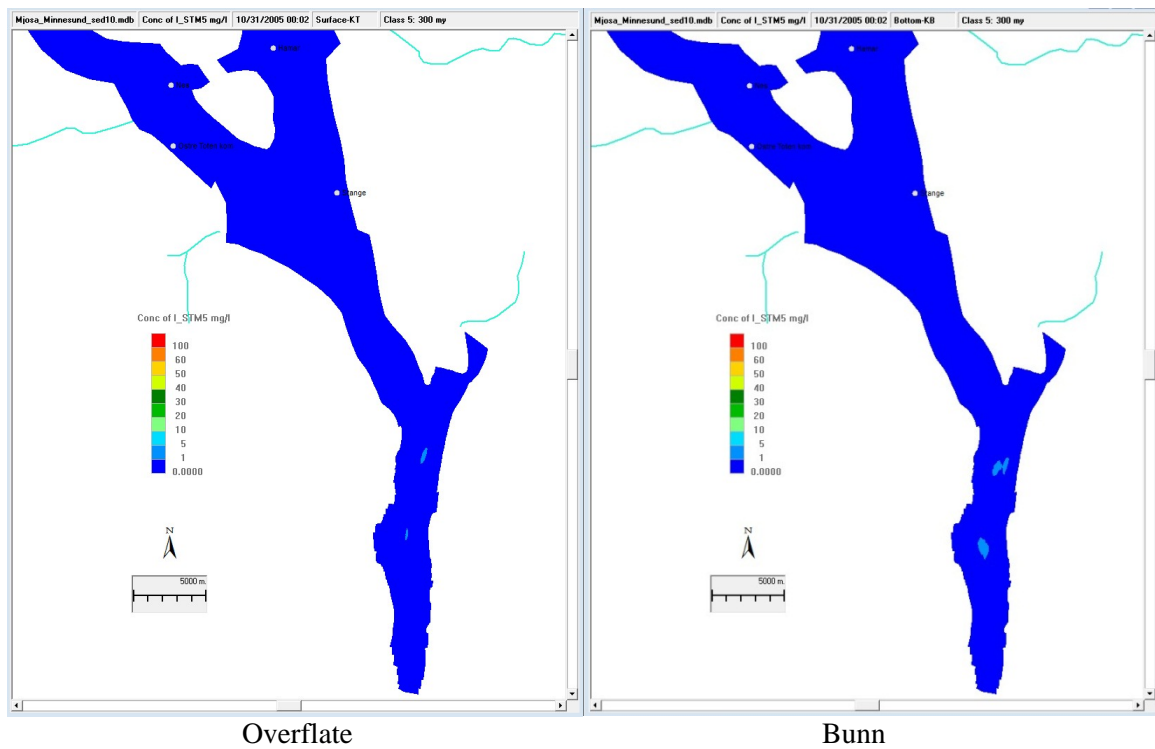
Figur 47. Kornstørrelses klasse 5, diameter = 300 µm. Overflatestrøm nordover 31. oktober. Partiklene forventes å sedimentere raskt.
