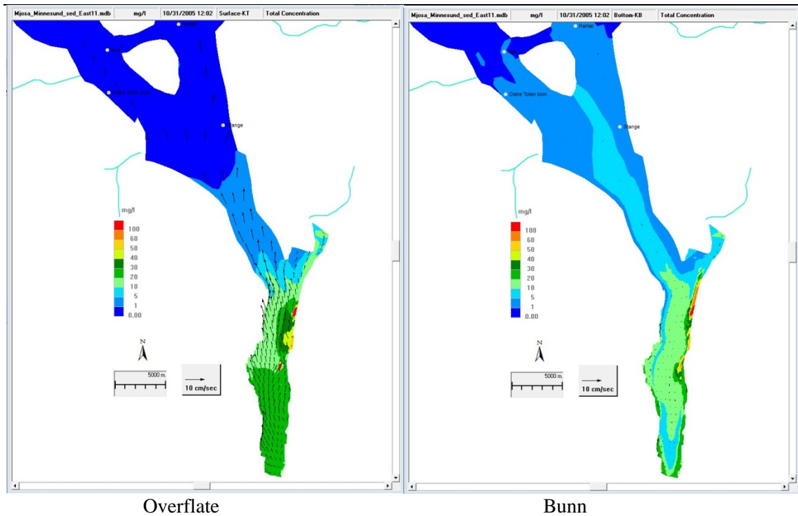
Figur 42. Total konsentrasjon av partikler. Overflatestrøm sørøver 31.oktober.
