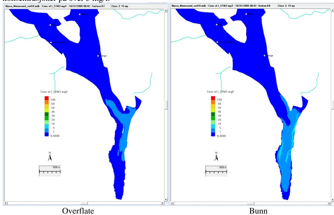
Figur 14. Modellerte konsentrasjoner av partikler i kornstørrelses klasse 3, diameter = 15 µm, gitt en overflatestrøm nordover den 31. oktober.
