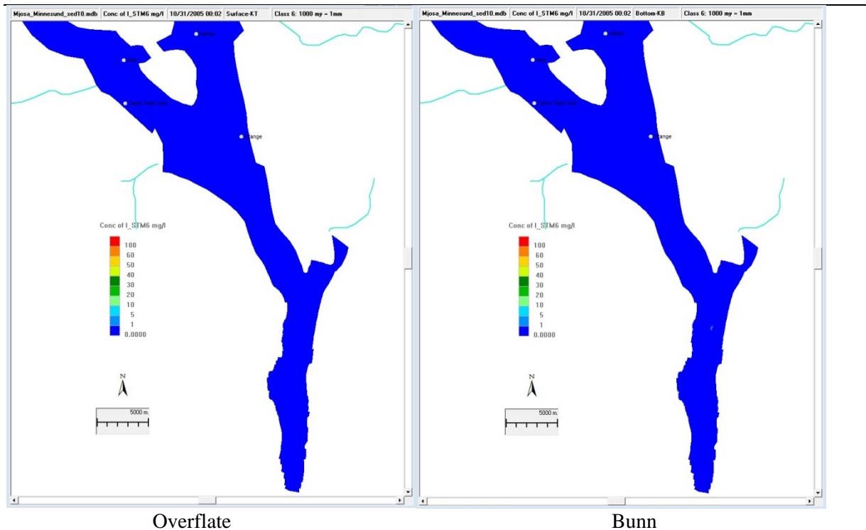
Figur 17. Modellerte konsentrasjoner av partikler i kornstørrelses klasse 6, diameter = 1000 \mu\text{m} = 1 mm, gitt en overflatestrøm nordover den 31. oktober.
