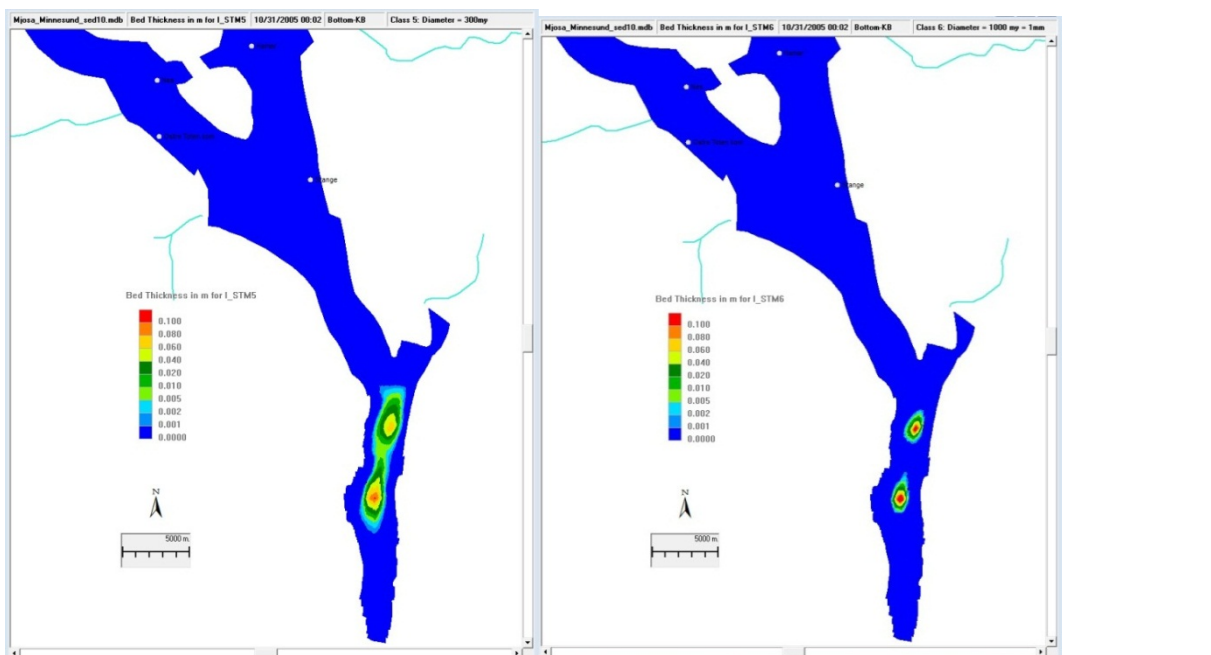
Kornstørrelses klasse 5, diameter = 300 \mu\text{m}
