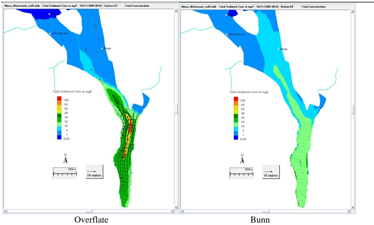
Figur 50. Total konsentrasjon av partikler. Overflatestrøm nordover.
