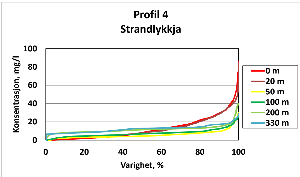
Figur 33. Strandlykkja. I halvparten av tiden ble konsentrasjonene i overflaten og på bunnen mindre enn henholdsvis 12 mg/l og 7 mg/l. Tilsvarende maksimumkonsentrasjoner ble 85 mg/l og 30 mg/l. Konsentrasjonene i overflaten varierte mye, men langt mindre på dypt vann.
