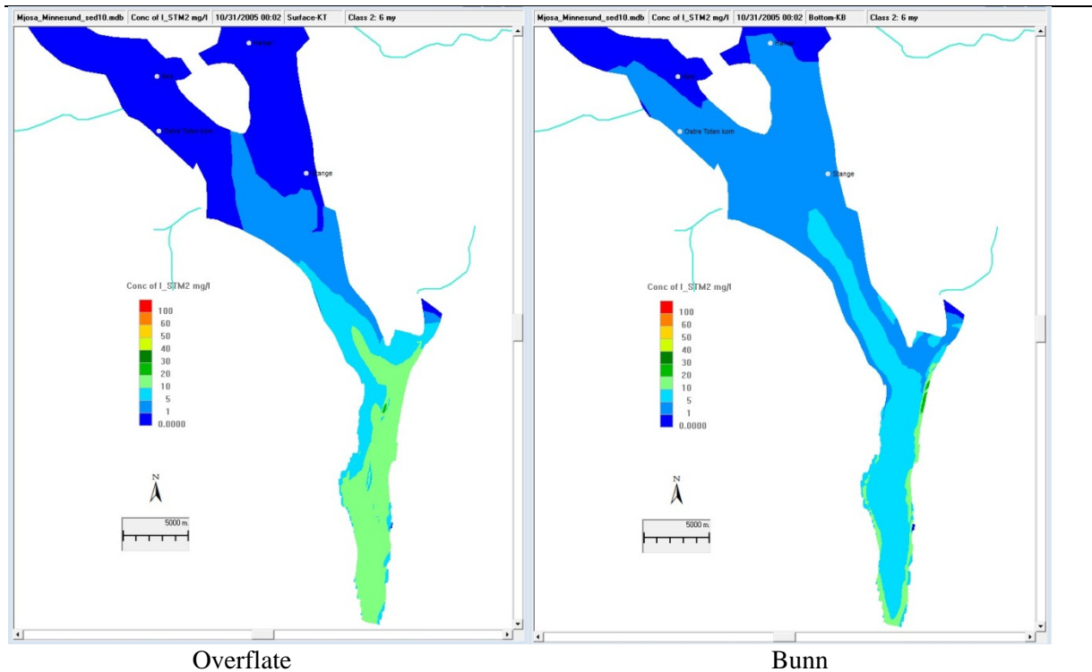
Figur 13. Modellerte konsentrasjoner av partikler i kornstørrelses klasse 2, diameter = 6 µm, gitt en overflatestrøm nordover den 31. oktober.
