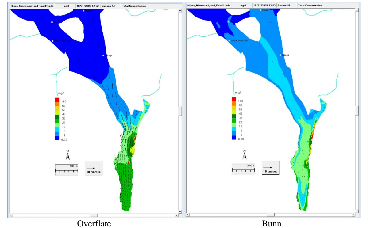
Figur 11. Beregnede total konsentrasjoner av partikler i overflatelaget og bunnære vannmasser gitt en situasjon med overflatestrøm nordover 31. oktober.
