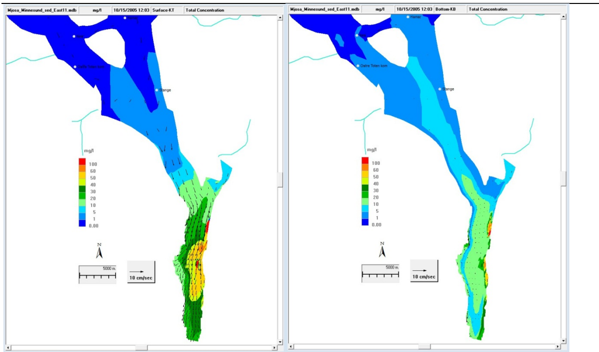
Figur 26. Total konsentrasjon av partikler gitt en overflatestrøm sørover den 15.oktober
