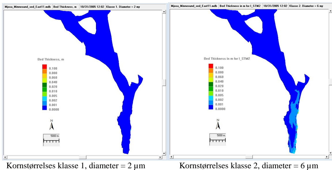
Figur 8. Partikler med diameter mindre enn 2 µm (leire og finere), sedimenterer praktisk talt ikke i strømmende vann. De ender tilslutt i havet. Klasse 2, med typisk diameter 6 på µm, mellom Tangen og Minnesund i et tynt lag på omkring et par millimetre.
