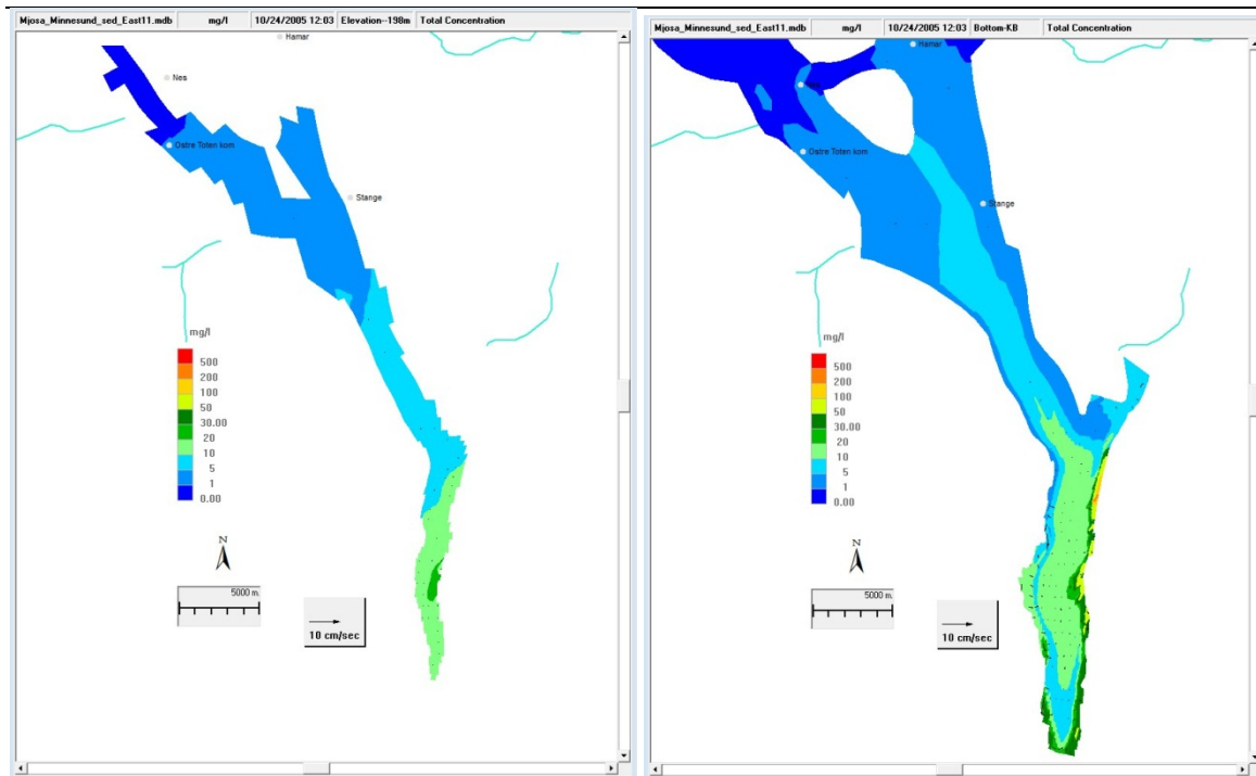
Figur 20. Total konsentrasjon av partikler gitt en overflatestrøm sørover den 24. oktober.
