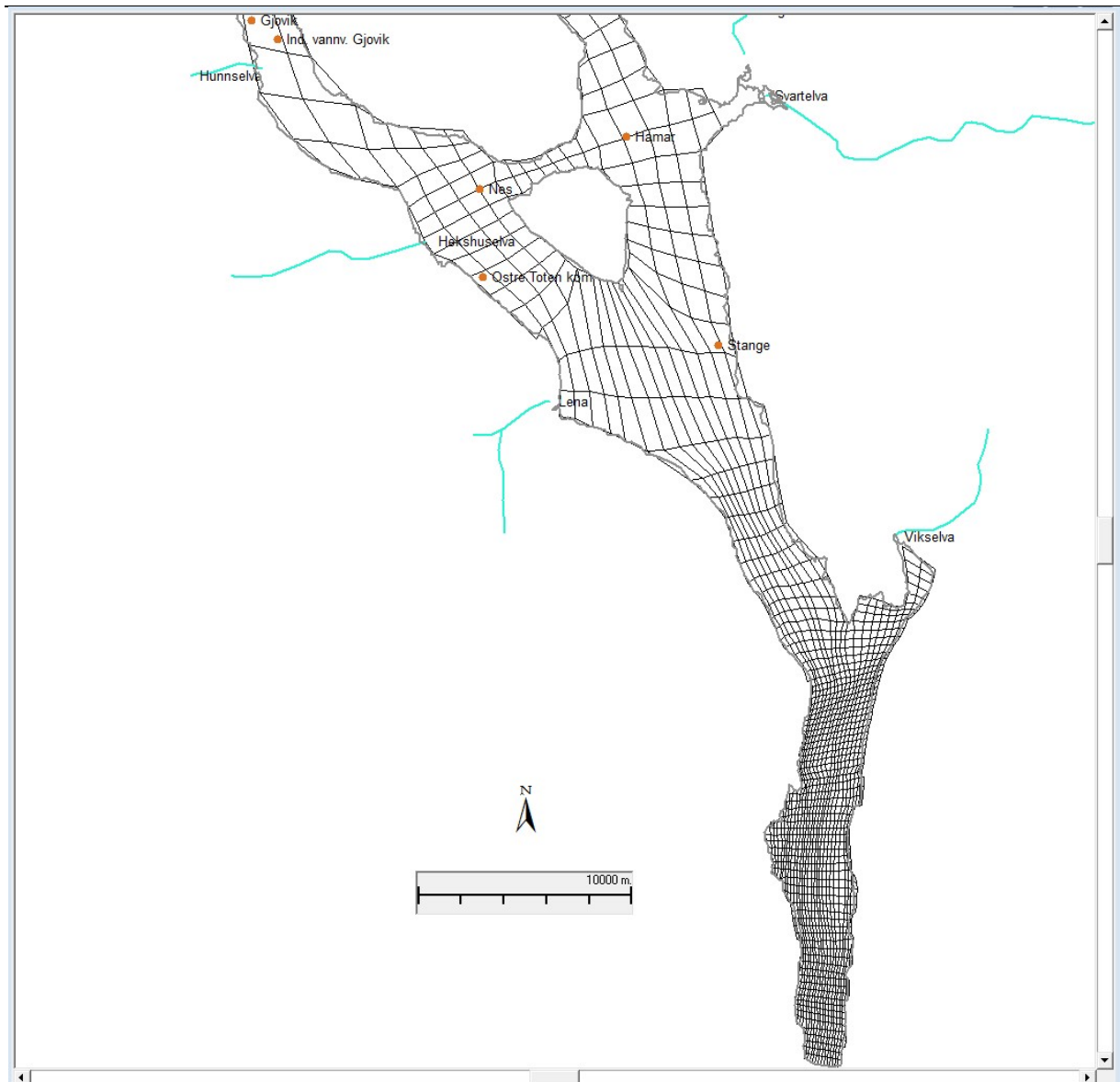
Figur 4. Mjøsa ble delt inn i beregningsceller som grunnlag for modelleringen. Vertikalt var cellene adskilt av horisontale lag.
