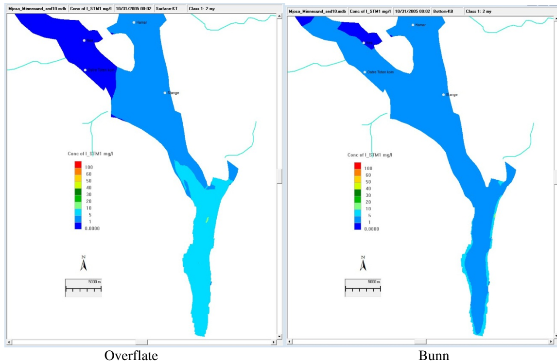
Figur 12. Modellerte konsentrasjoner av partikler i kornstørrelses klasse 1 ( diameter = 2 µm ) i overflate- og bunnære vannmasser gitt en overflatestrøm nordover 31. oktober. De minste partiklene (leire) spredte seg mest i overflaten, over 5 mg/l. På bunnen ble konsentrasjonene nær de naturlige bakgrunnsverdiene på ca. 1 mg/l.
