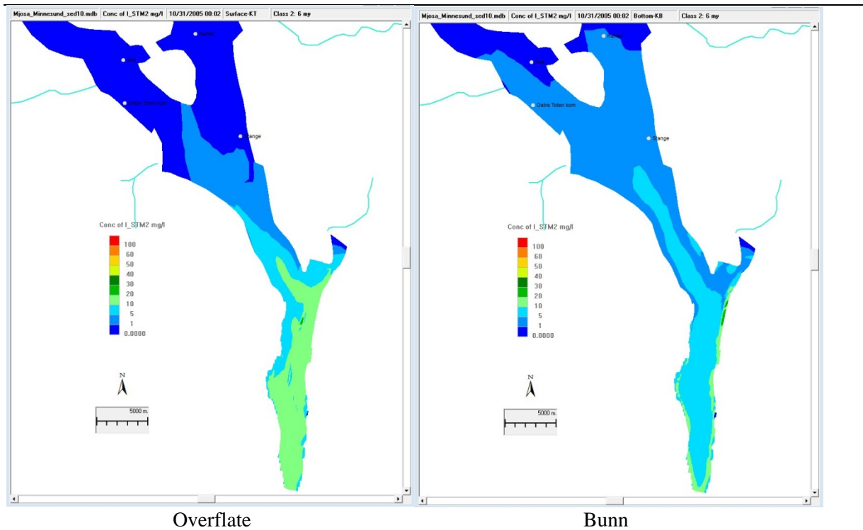
Figur 44. Kornstørrelses klasse 2, diameter = 6 µm. Overflatestrøm nordover 31. oktober. Verdier over 10 mg/l forventes i overflaten sør for Tangen. Langs bunnen på stort dyp forventes konsentrasjoner på over 5 mg/l.
