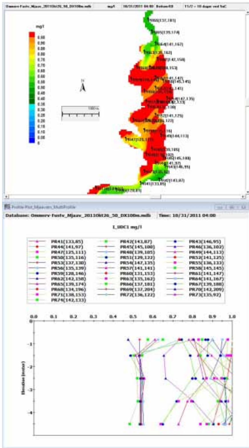
Figur 41. I den sentrale delen av Mjøvatn var konsentrasjonene i alle dybdeprofilene over 0,6 mg/l. I begge endene av strekningen, med stor elveliknende vannutskifting, var konsentrasjonene lavere. Disse delene fikk konsentrasjoner over 0,7 mg/l via en «bølge» av høye konsentrasjoner som forplantet seg nedstrøms.
