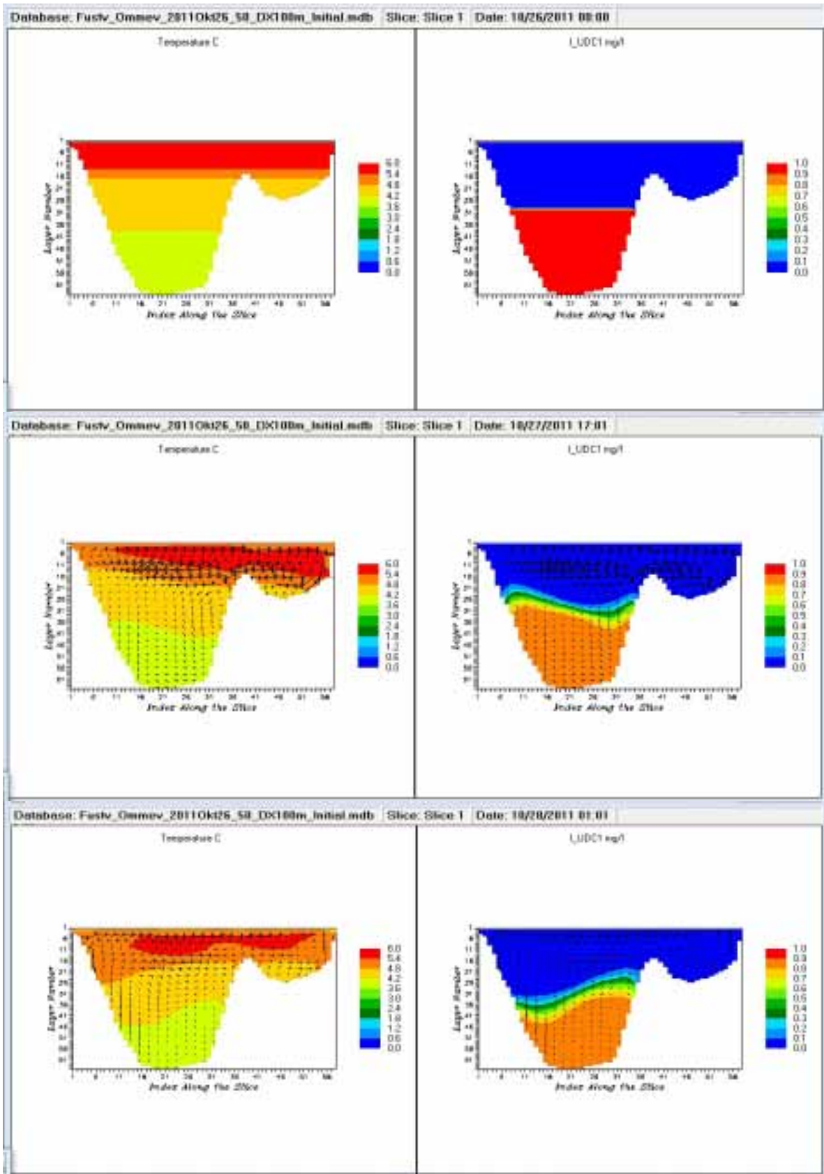
Temperatur Konsentrasjon av konservativt sporstoff Figur 32. Eksempel på hvordan varierende vind kan sette i gang indre bølger. Stoffet vil fortrinnsvis strømme fram og tilbake i samme nivå. (Samme tverrsnitt i Ømmervatn som på de øvrige figurene.)
