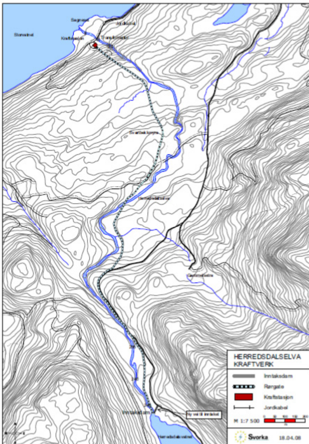
Figur 2. Detaljkart over utbyggingsområdet som viser inntakssted og rørgate samt lokalisering av kraftstasjon. Kilde: Konsesjonssøknad.
