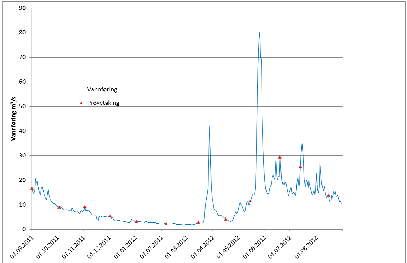
Figur 3. Døgnmiddelvannføring i Folla ved Grimsmoen i 2011-12 med markering av prøvetakinger.
