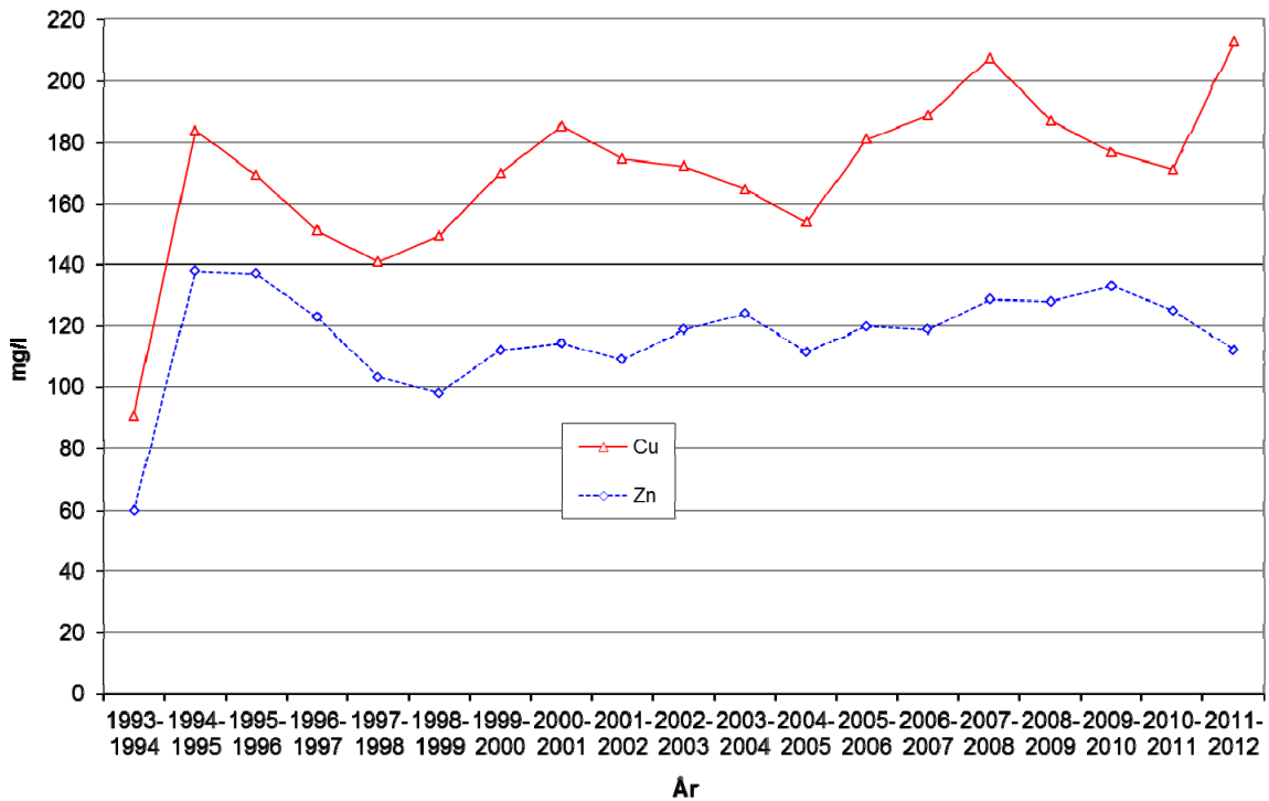
Figur 8. Stoll2. Tidsveiede årsmiddelverdier for kobber og sink 1993-2012.
