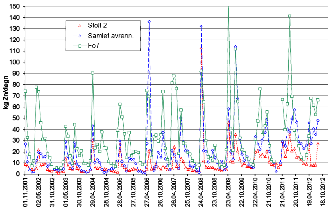
Figur 15. Døgntransportverdier for sink i perioden 2001-2012.
