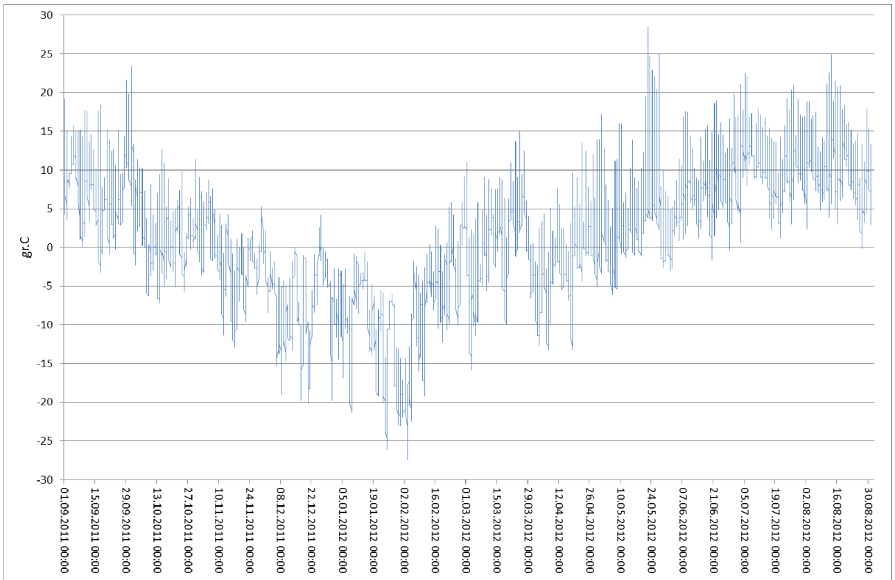
Figur 2. Lufttemperaturer ved Stoll 2 i Folldal sentrum 2011-2012.
