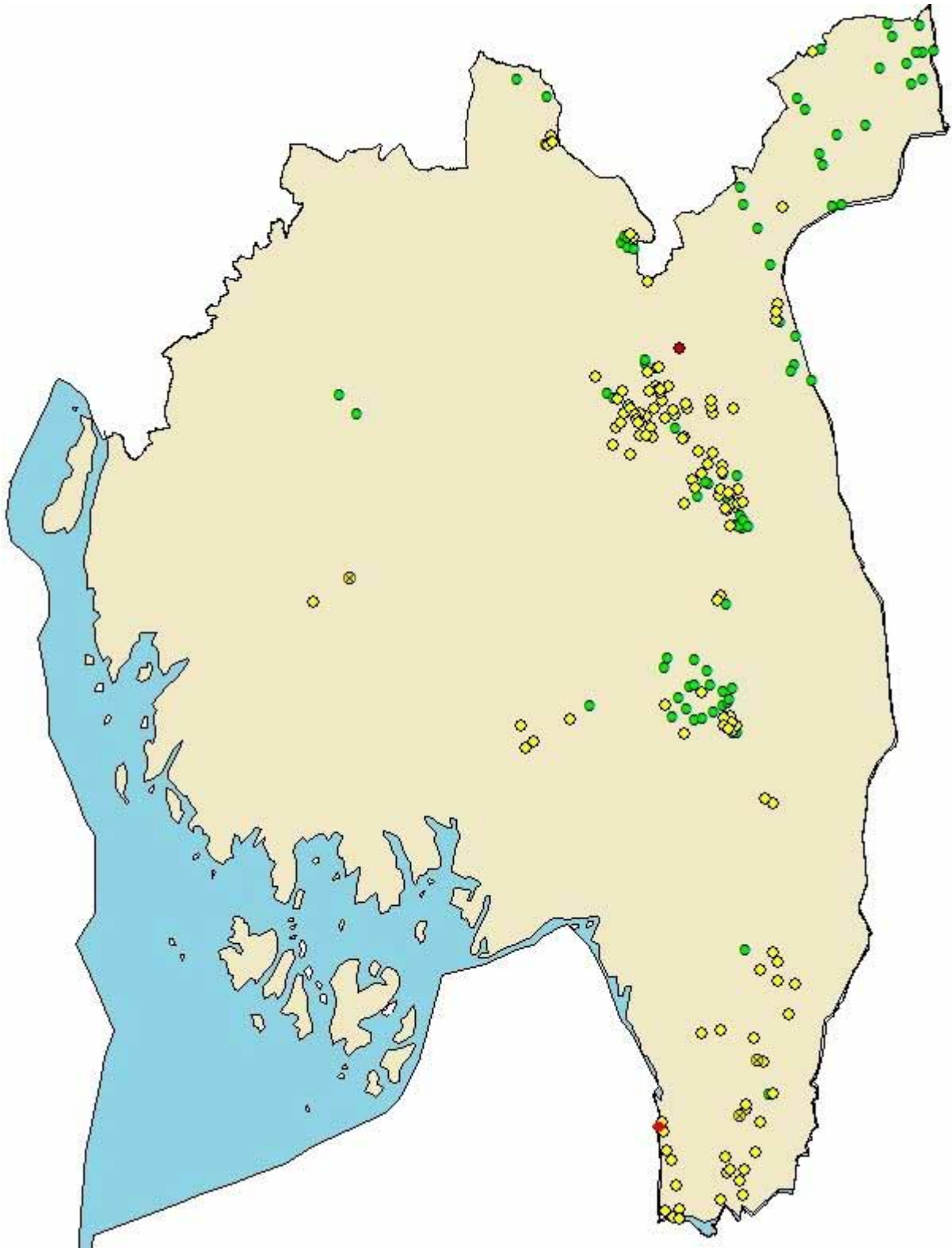
Figur 8. Vurdering av fortsatt kalkingsbehov for 212 kalkede innsjøer i Østfold. Grønn sirkel: kalking kan avsluttes. Gul sirkel: usikkert om kalking kan avsluttes. Gul sirkel med kryss: innsjøer med sulfat og/eller kloridkonsentrasjon utenfor området som modellen er gyldig for. Rød sirkel: kalking må fortsette.
