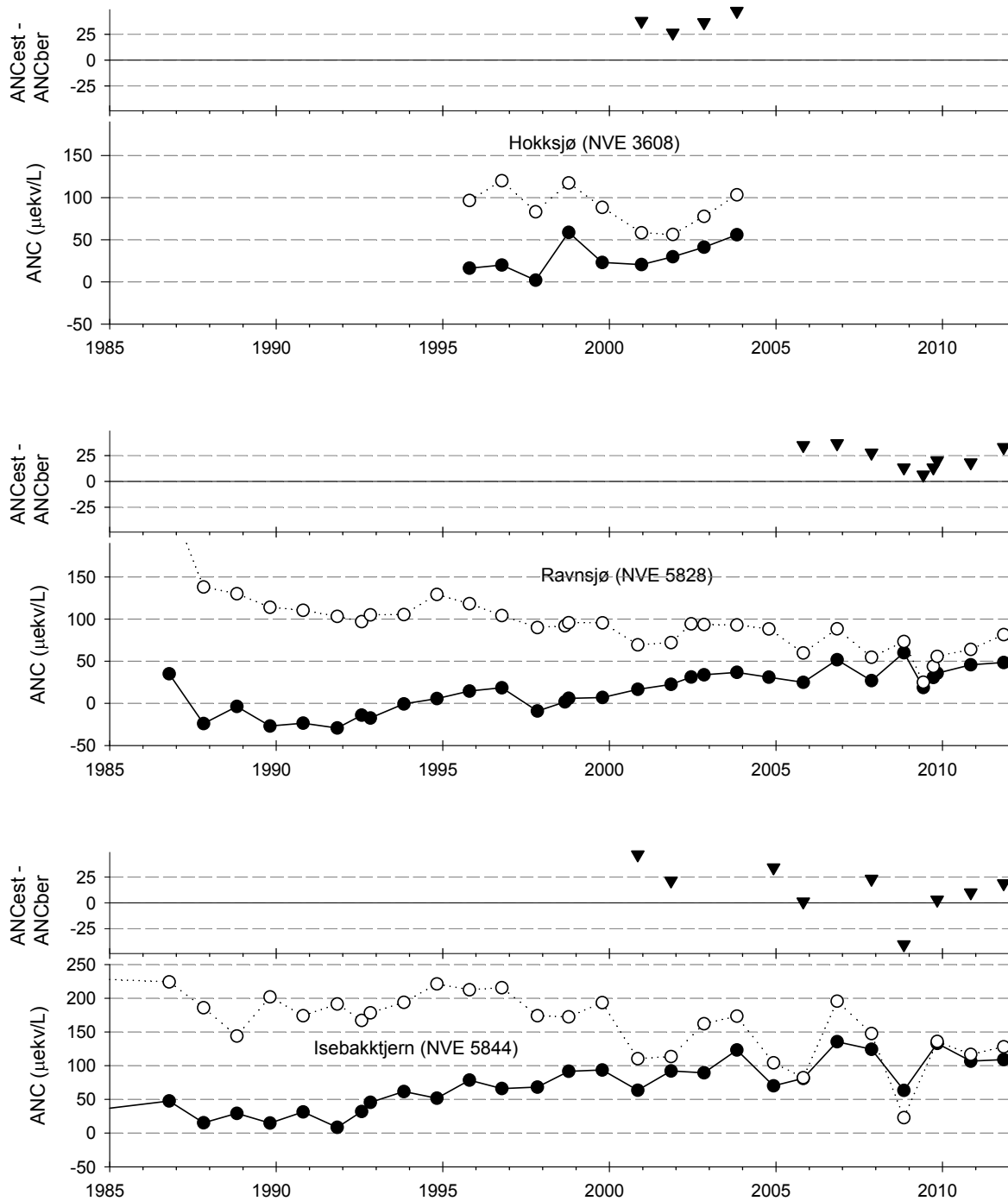
Figur 6. ANC estimert med modellert Ca (åpne sirkler), og ANC beregnet med målte Ca-konsentrasjoner (fylte sirkler). Fylte trekanter viser differansen mellom disse. NB, skalaen på y-aksen til det nederste panelet er forskjellig fra de andre.
