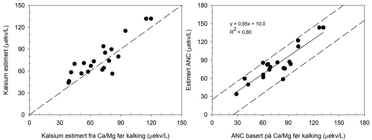
Figur 7. Estimert «ukalket» Ca-konsentrasjon i 2011 mot Ca-konsentrasjon basert på Ca/Mg-forholdet før kalking og målt Mg-konsentrasjon i 2011 (venstre), og hvilken betydning det har for ANC (høyre). Hele linjer representerer beste lineære tilpasning og stiplede linjer viser 1:1 linjen (venstre) eller 1:1 linjen +/- 25 µekv/L (høyre).
