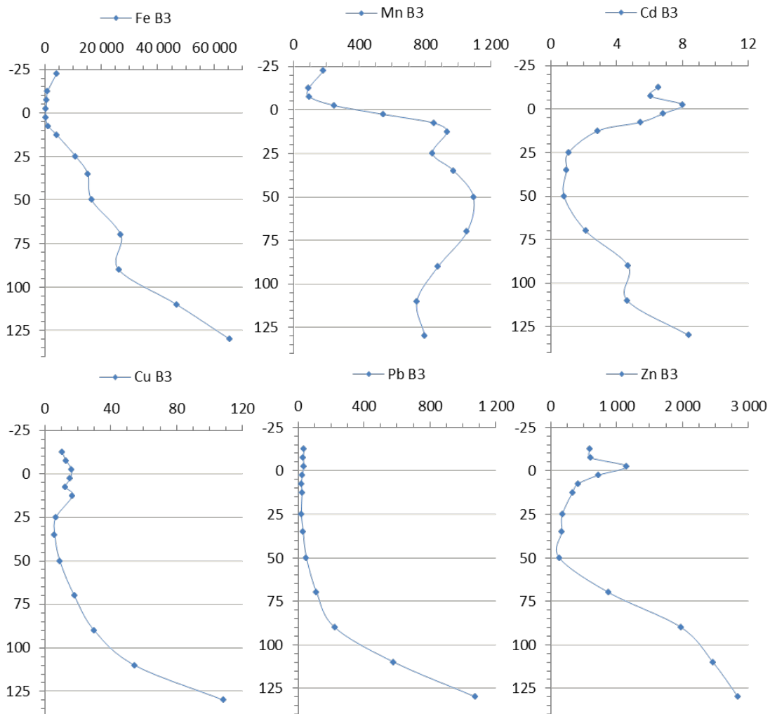
Figur 25. Vertikalprofiler målt med DGT-prober i boks 3 fra område D. Enhet er ng\ cm^{-2} .
