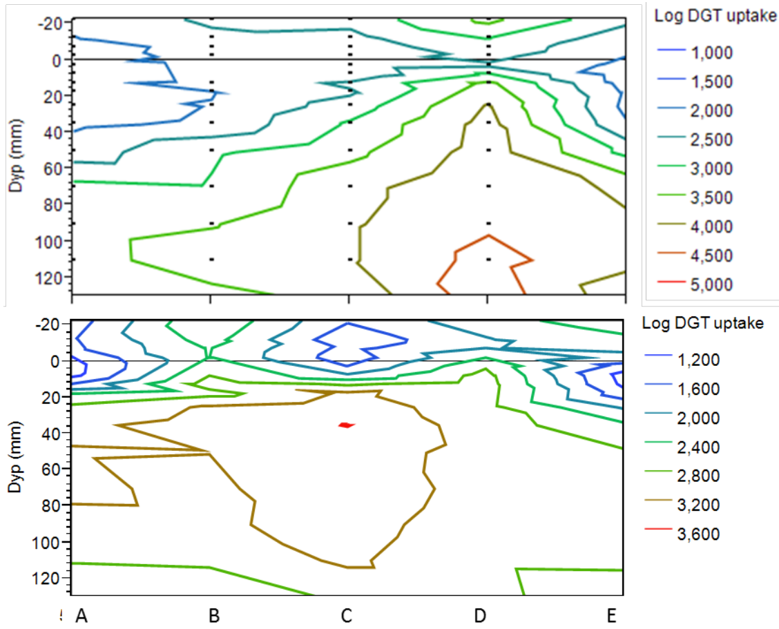
Figur 17. DGT opptak av jern (øverst) og mangan (nederst) i de fem områdene i Sjørfjorden. Merk logaritmisk skala som viser at opptaket av Fe øker fra mindre enn 100 \text{ ng cm}^{-2} i sediment-vann grenseflaten i område A til mer enn 50\,000 \text{ ng cm}^{-2} i dypere lag i område D.
