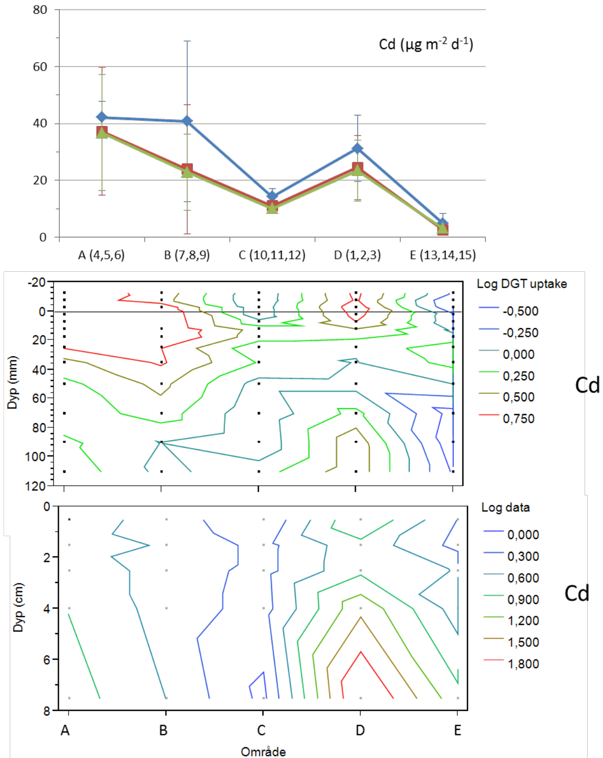
Figur 18. Konsentrasjonen av kadmium i sediment ( \text{mg kg}^{-1} \text{TS} ) (nederst), opptak i DGT ( \text{ng cm}^{-2} ) (midten) og utlekking til vannmassen (øverst) fra de fem områdene i Sørfjorden fra innerst i havnebassenget (område A) til Tyssedal (område E). Isoplet-diagrammene er konstruert fra logaritmiske verdier.
