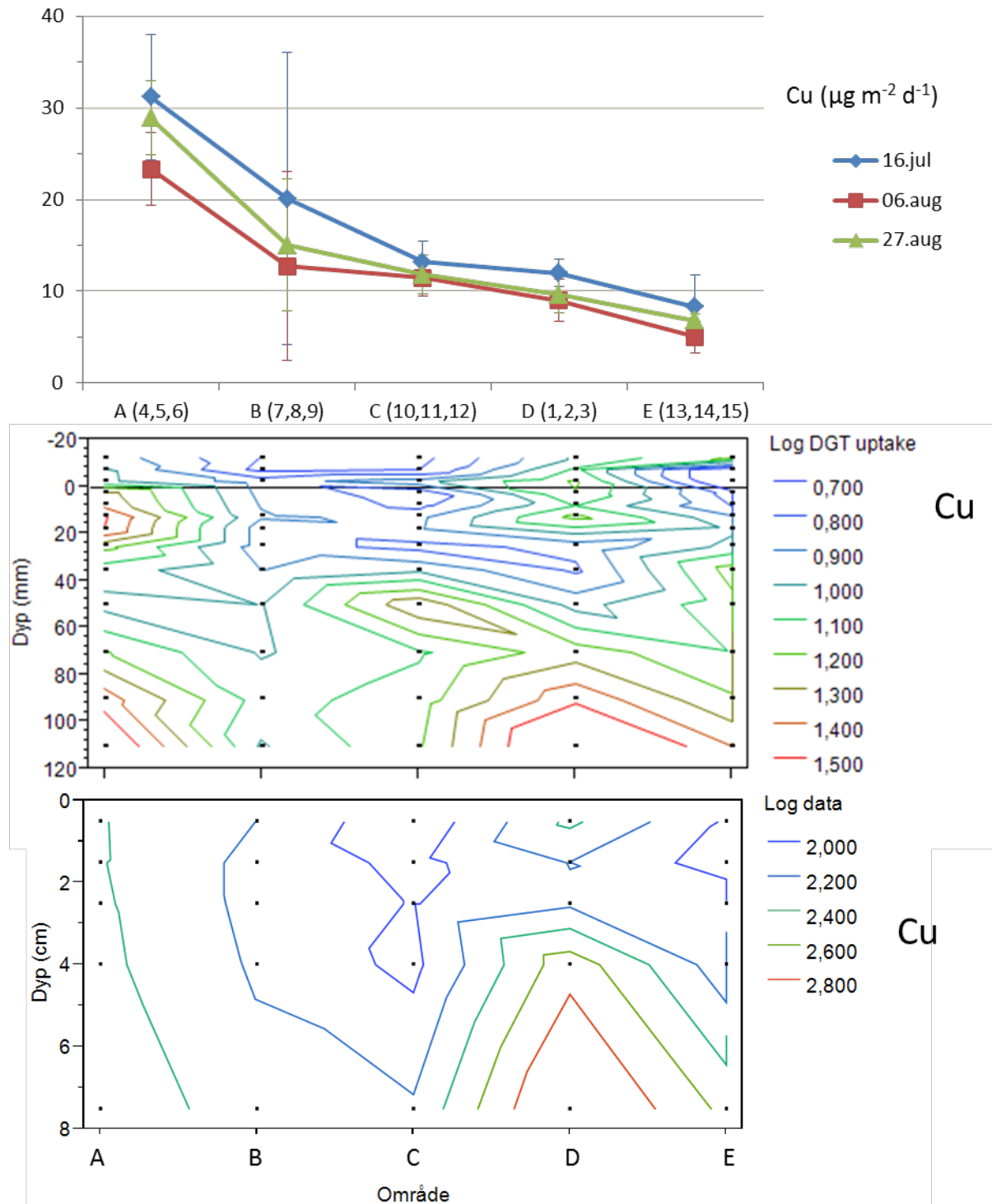
Figur 19. Konsentrasjonen av kopper i sediment ( \text{mg kg}^{-1} \text{TS} ) (nederst), opptak i DGT ( \text{ng cm}^{-2} ) (midten) og utlekking til vannmassen ( \mu\text{g m}^{-2} \text{d}^{-1} ) (øverst) fra de fem områdene i Sør fjorden fra innerst i havnebassenget (område A) til Tyssedal (område E). Isoplet-diagrammene er konstruert fra logaritmiske verdier.
