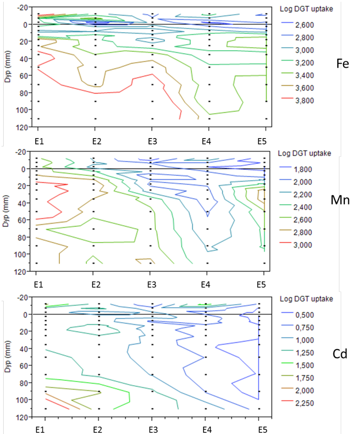
Figur 22. Opptak av jern (øverst), mangan (midten) og kadmium (nederst) på DGT'er utplassert i Eitrheimsvågen. E5 innerst i bukta, E1 ca 400m lenger ut.
