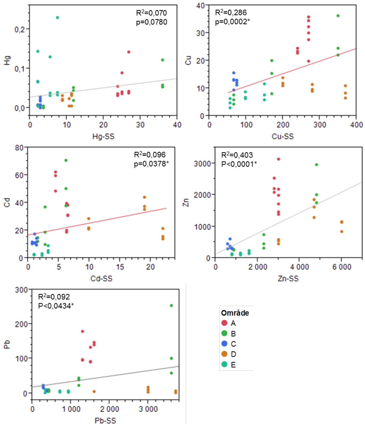
Figur 15. Plot av metall utlekking (y-aksen) mot respektive metall konsentrasjon i 0-1 cm av sedimentene (x-akse). Regresjonslinje, korrelasjonskoeffisient ( R^2 ) og sannsynligheten (p) for at utlekking ikke øker med økende konsentrasjon i sedimentet er vist i hvert enkelt diagram.
