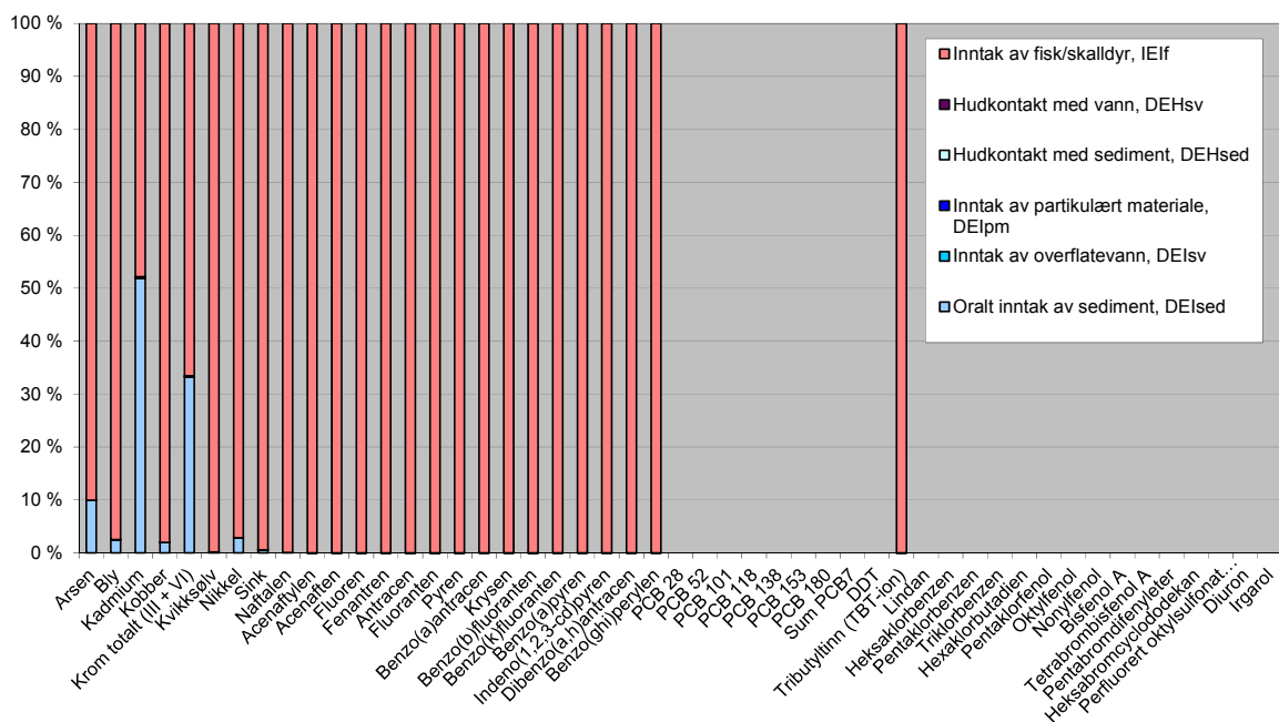
Figur 17. Prosentvis fordeling av miljøgiftspredning på de ulike spredningsveiene fra sedimentet i området utenfor Bulkterminalen til mennesker.
