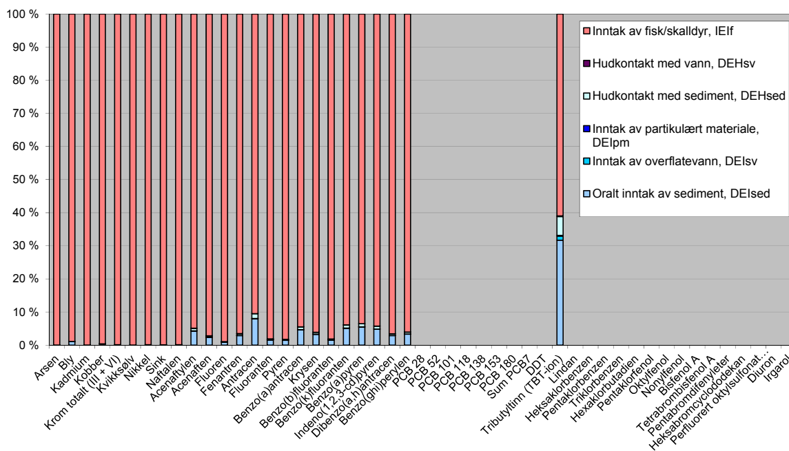
Figur 13. Prosentvis fordeling av miljøgiftspredning på de ulike spredningsveier fra sedimentet i området utenfor Rana Industriterminal til mennesker.
