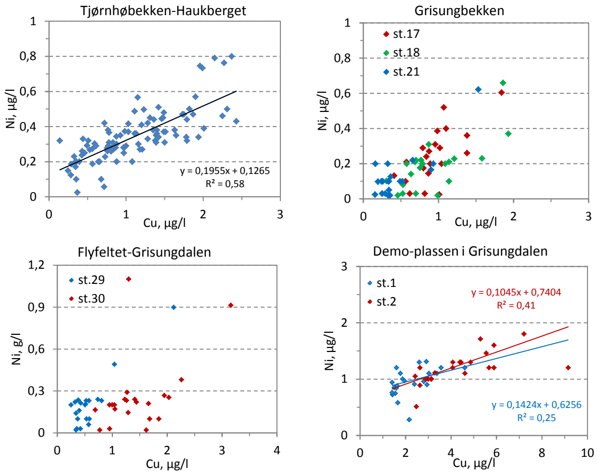
Figur 5. Samvariasjonen mellom konsentrasjonene av kobber og nikkell på alle stasjonene i Tjørnhøbekken, Grisungbekken, flyfeltet og demoleringsplassen i Grisungdalen.
