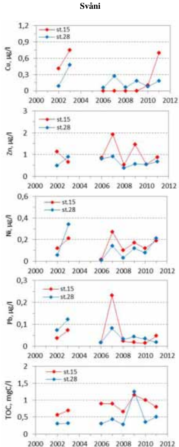
Figur 12. Middelskonsentrasjoner (mai-okt.) av totalt organisk materiale (TOC), sink (Zn), kobber (Cu) og nikkel (Ni) i Svåni inn (st.28) og ut av feltet (st.15) i perioden 2002 til 2011.
