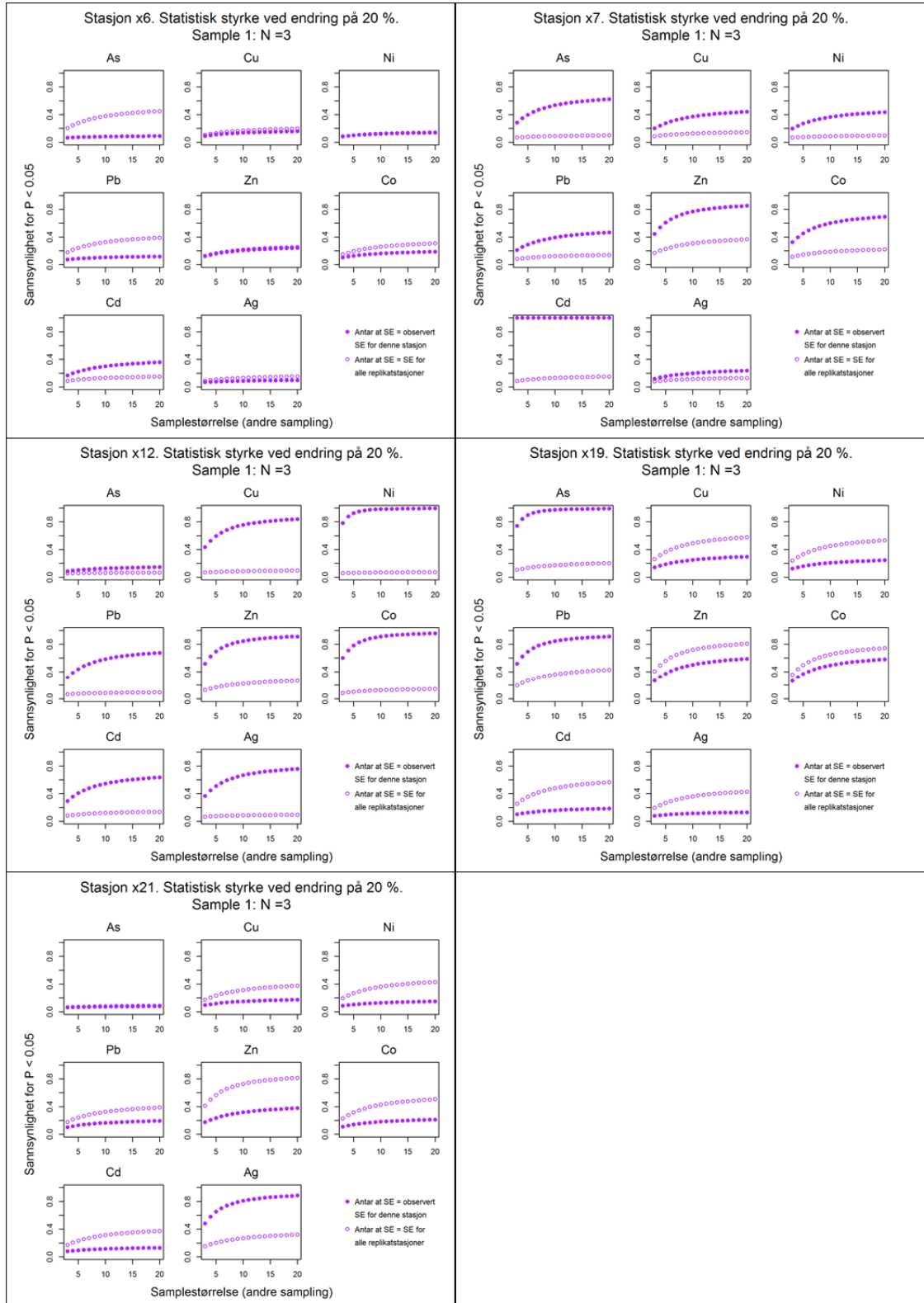
Figur 25. Sannsynlighet for å detektere en 20% endring i konsentrasjon gitt et utgangspunkt på triplikate prøver.
