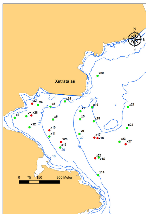
Figur 8. Sedimentprøvetakingsstasjoner i Hanneviksbukta. Grønne punkt markerer stasjoner det ble tatt godkjente sedimentprøver fra. Røde punkt markerer stasjoner der det ikke ble godkjente sedimentprøver pga. steinbunn, fjell eller for tynt sedimentlag.
