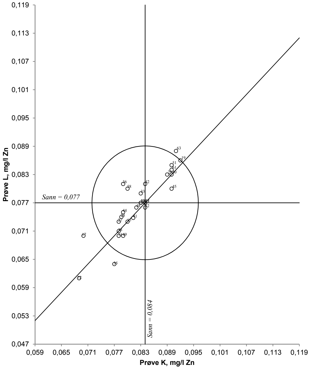
Figur 36. Youndendiagram for sink, prøvepar KL Akseptansegrensen, angitt med en sirkel, er 15 %
