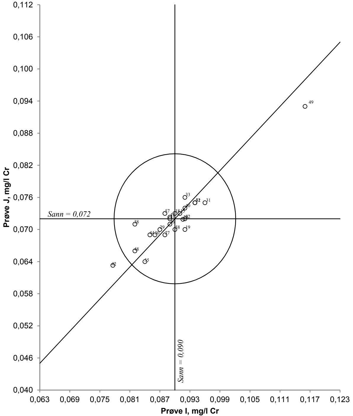
Figur 29. Youdendiagram for krom, prøvepar IJ Akseptansegrensen, angitt med en sirkel, er 15 %
