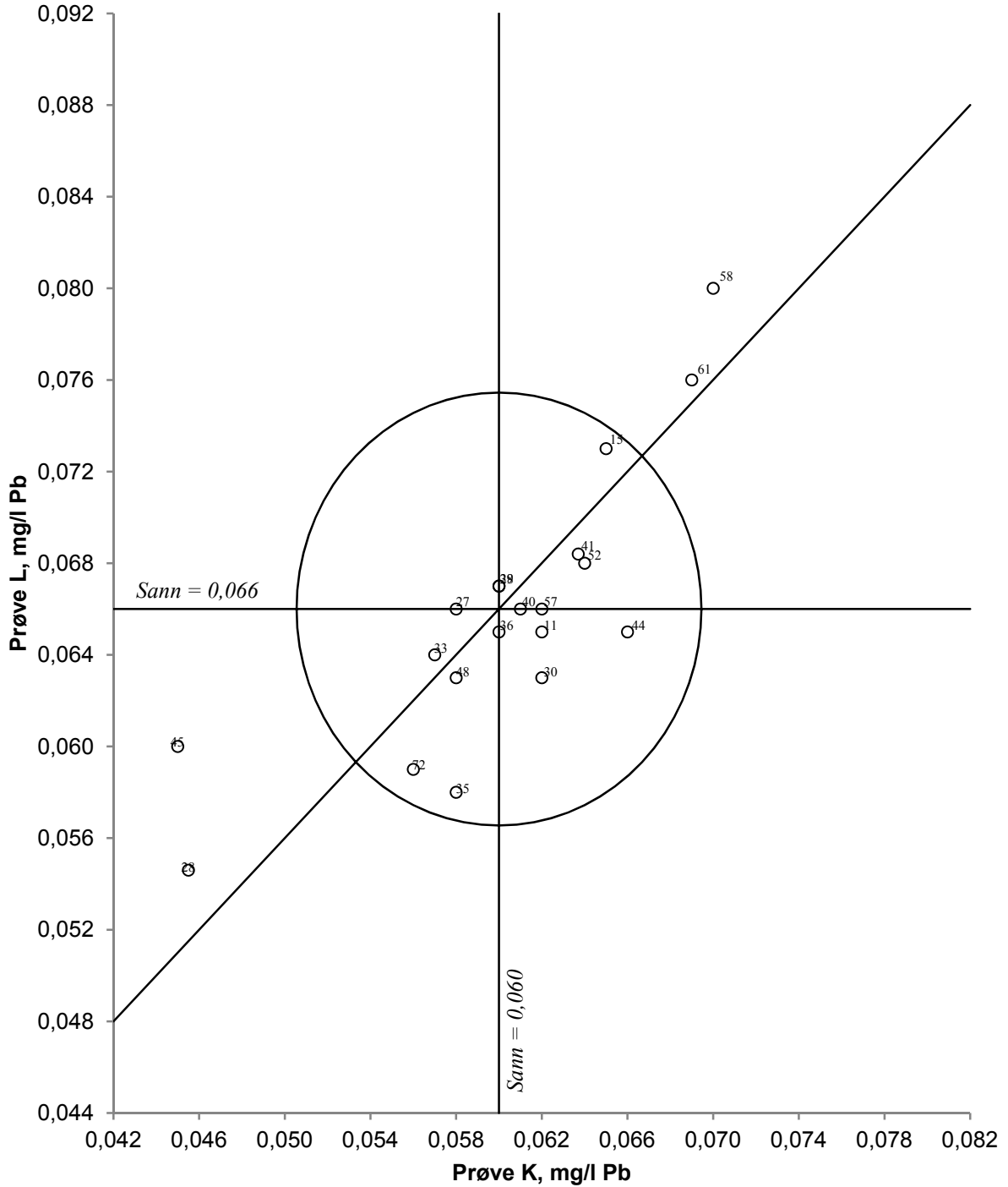
Figur 22. Youdendiagram for bly, prøvepar KL Akseptansegrensen, angitt med en sirkel, er 15 %
