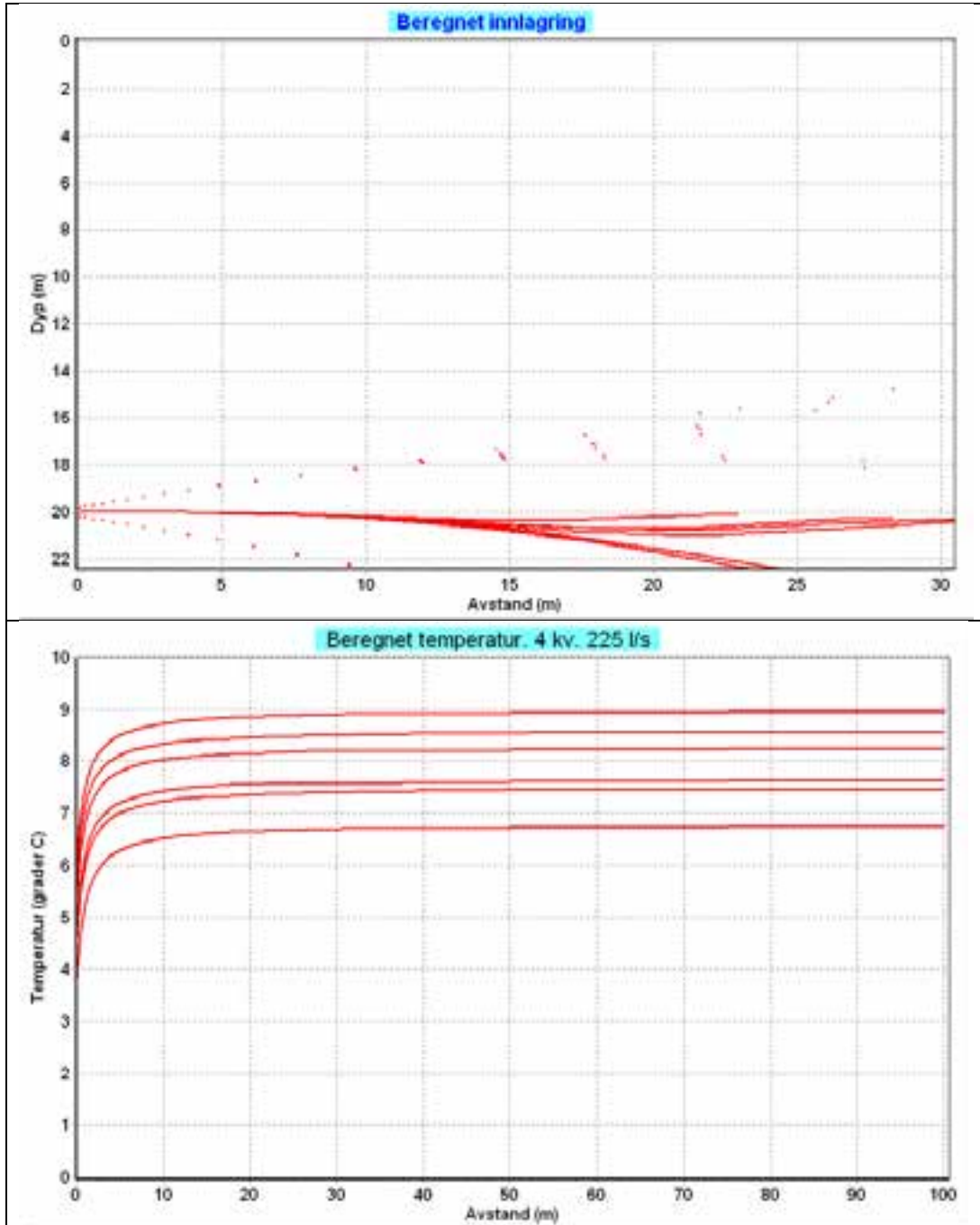
Figur 16. Utslipp av 225 l/s i oktober og desember. Avkjøling 3 °C. Øverst: kjølevannets innlagring. Nederst: kjølevannets temperatur.
