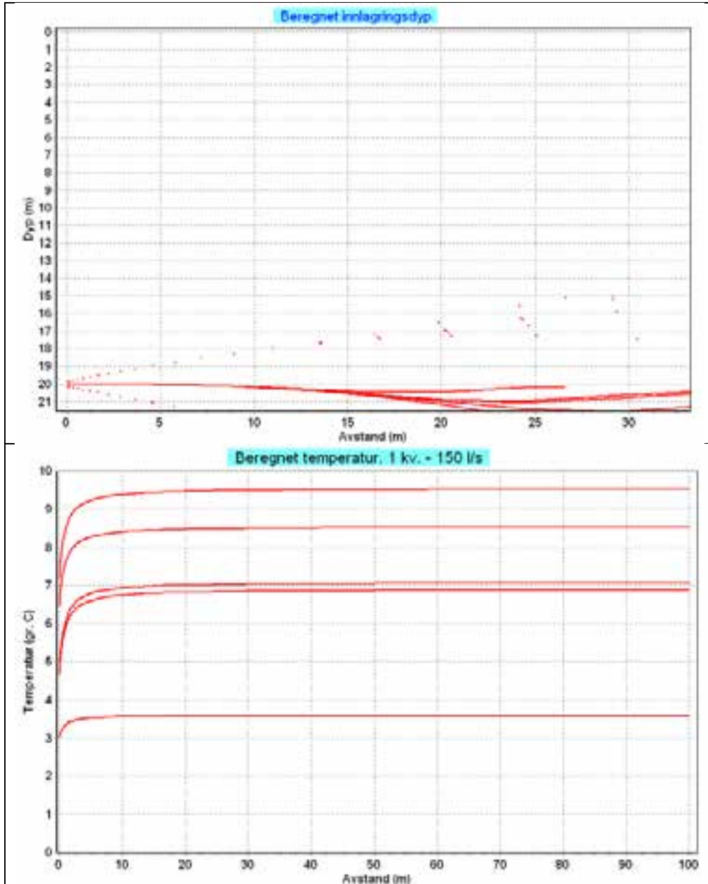
Figur 6. Utslipp av 150 l/s i januar-februar. Avkjøling 2,4 °C. Øverst: kjølevannets innlagring. Nederst: kjølevannets temperatur.
