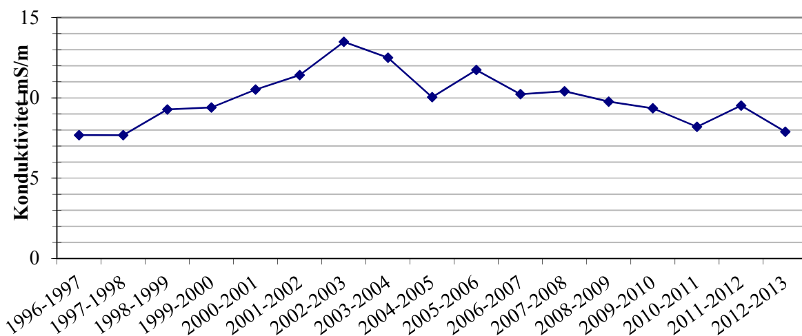
Figur 8 Tidsveiede årsmiddelverdier for konduktivitet i Orva. Hydrologiske år 1996-2013.
