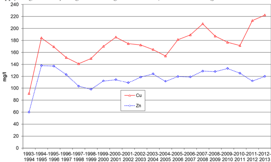
Figur 8. Stoll 2. Tidsveiede årsmiddelveier for kobber og sink 1993-2013.
