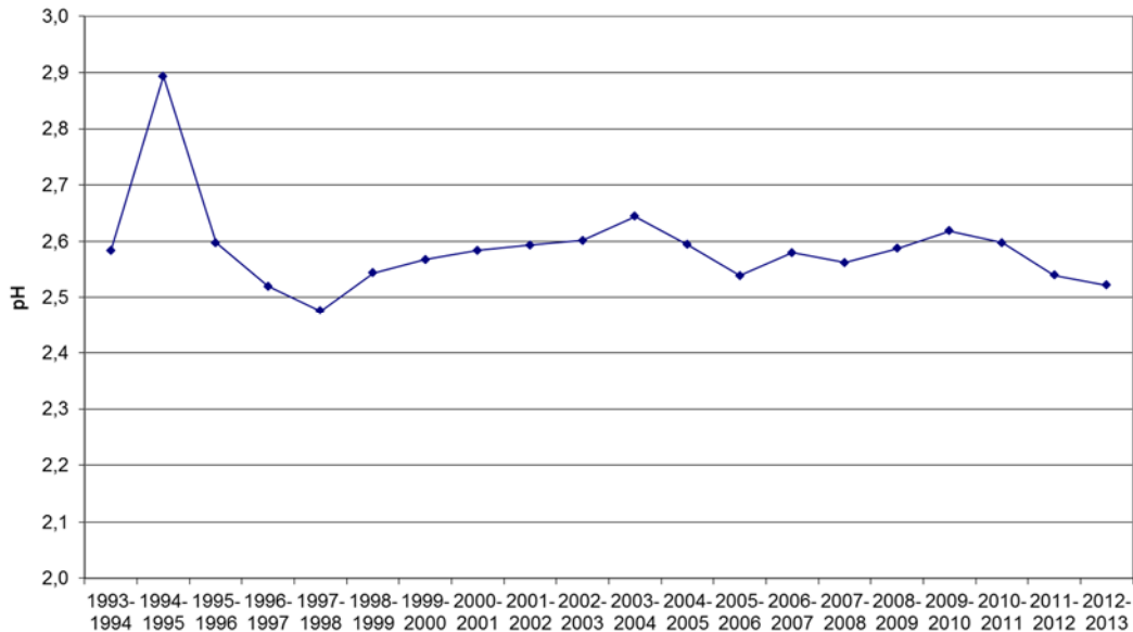
Figur 7. Stoll 2. Tidsveiede årsmiddelveier for pH 1993-2013.
