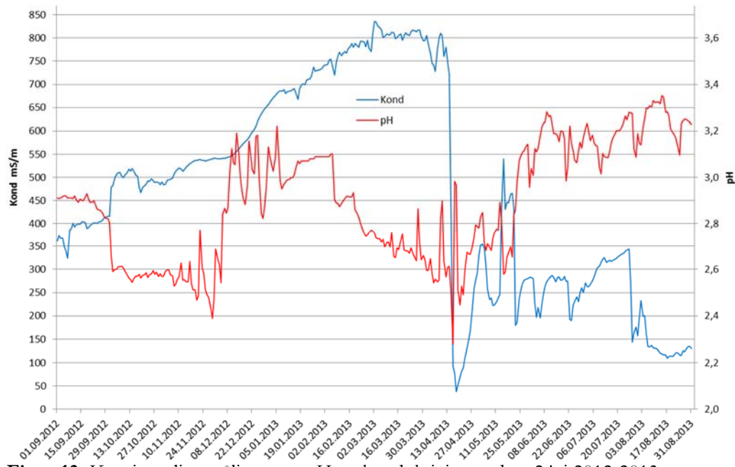
Figur 13. Kontinuerlige målinger av pH og konduktivitet ved st. 2A i 2012-2013.
