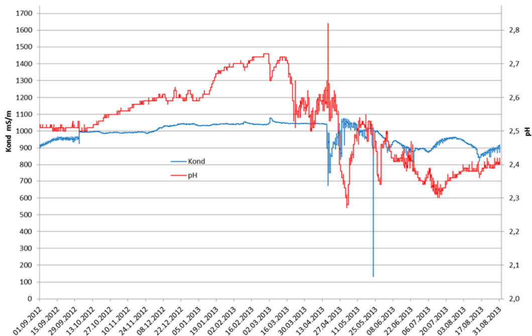
Figur 10. Kontinuerlige målinger av pH og konduktivitet ved utløpet av stoll 2 i 2012-2013.
